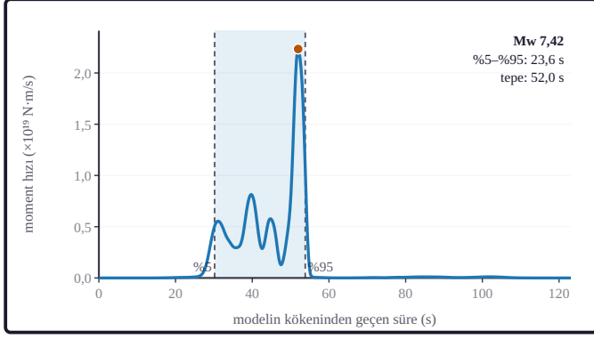
Şekil 6a. Eğri USGS sonlu fay modelinin (sürüm 1; gözden geçirilmiş ürün; 14.08.2026) moment hızı fonksiyonudur; zaman modelin kendi kökenine göre; modelin toplam sismik momenti M_0 = 1,72 \times 10^{20} N·m, Mw 7,42; gölgeli bant birikimli momentin %5'ine (30,2 s) ve %95'ine (53,8 s) ulaşılan anlar arasıdır; aradaki süre (moment salınımının %90'ının gerçekleştiği süre) 23,6 s'dir; dolu daire en büyük moment hızıdır: 2,2 \times 10^{19} N·m/s, 52,0 s'de; eğri ters çözümün model çıktısıdır, ölçülmüş bir zaman serisi değildir (kurum ürünü: USGS sonlu fay modeli [U.S. Geological Survey, 2017]; yöntem: Ji vd., 2002).
