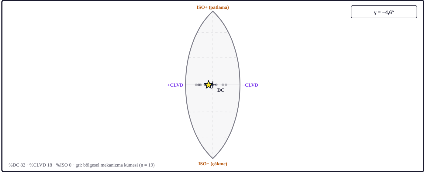
Şekil 7a. Tape ve Tape kaynak tipi lune'unda sarı yıldız bu olayın moment tensörünü, artı imi saf çift kuvvet (DC) merkezini gösterir. Çerçeve \gamma \in [-30^\circ, +30^\circ] ve \delta \in [-90^\circ, +90^\circ] aralığının Hammer eşit alan izdüşümüdür; kesikli yaylar \delta = 0, \pm 30^\circ ve \pm 60^\circ enlemleridir. Sağ ve sol kenarlar \pm CLVD uçları, kutuplar izotropik patlama ve çökme uçlarıdır. Gri noktalar bölgesel mekanizma kümesinin çözümleridir; alt satırdaki yüzeler DC/CLVD/ISO ayrışımıdır (lune: Tape ve Tape, 2012; ayrışım: GCMT tensöründen).
