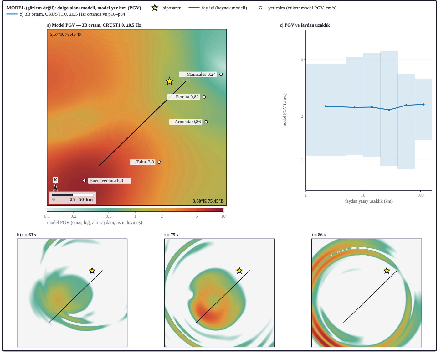
Şekil 16. Dalga alanı modeli, MODEL — gözlem değil: a) 3B ortam, CRUST1.0 çözümünde \leq 0,5 Hz model yer hızı (PGV); renk ölçeği logaritmik, 0,1–10 cm/s, alt sınırın altı saydam, üst sınırın üstü doymuş; b) aynı çözümün t = 63, 75 ve 86 s anlarındaki hız büyüklüğü |v|, aynı renk ölçeğiyle; c) PGV ile faydan yatay uzaklık, model başına kuşak ortancası (çizgi) ve p16–p84 aralığı (bant), iki eksen logaritmik; kinematik kaynak: us6000tjl2; kırılma süresi 120 s; havza büyütmesi ve yerel zemin etkisi hesapta yoktur; 3B ortamda kayma dalgası hızı tabanı 2,571 km/s (model: Seismo Lab dalga alanı hesabı — 3B ortam: Seismo Lab kendi sonlu farklar çözücüsü yz-sf3b/2 [Virieux, 1986; Graves, 1996, Q sönümü: Day, 1998], CRUST1.0, Laske vd., 2013; kaynak: us6000tjl2).
