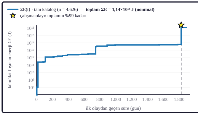
Şekil 5c. Mavi basamak eğrisi kümülatif ısınan sismik enerjidir ( \Sigma E , logaritmik eksen). Kesikli düşey çizgi çalışma olayını işaretler; en büyük tek katkı bu olaydır (Gutenberg ve Richter, 1956 enerji bağıntısı).
