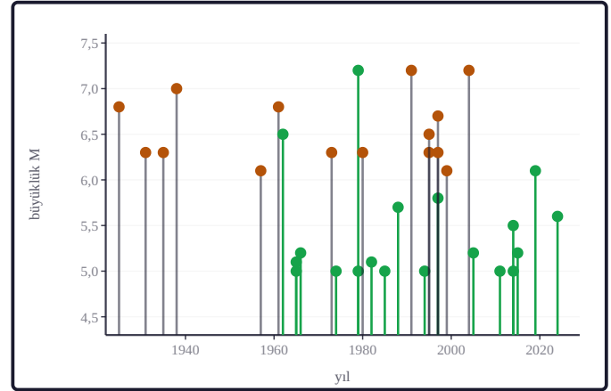
Şekil 18b. Tarihsel çişik üstü depremlerin büyüklükleri yıllara göre çizilmiştir; yeşil yakın kuşak, turuncu bölge kuşağıdır; sap rengi aynı ayrımı verir (yeşil sap yakın kuşak, gri sap bölge kuşağı) (birleşik katalog, 1900 sonrası; büyüklükler, varsa ISC-GEM Mw: International Seismological Centre, 2026; Di Giacomo vd., 2015, 2018).
