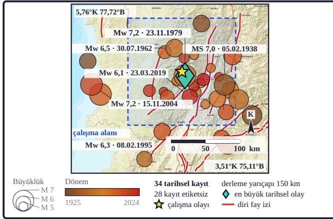
Şekil 18a. Çalışma olayından önceki eşik üstü kayıtlarda daire çapı büyüklüğü, dolgu rengi oluş dönemini gösterir. Turkuaz elmas derlemenin en büyük kaydı, sarı yıldız çalışma olayıdır. Kayıt eşiği yakın kuşakta M \geq 5 , bölge kuşağında M \geq 6 olarak alınmıştır. Mavi kesikli dikdörtgen çalışma alanıdır (birleşik katalog, 1900 sonrası; derleme yarıçapı 150 km, yakın kuşak 60 km).
