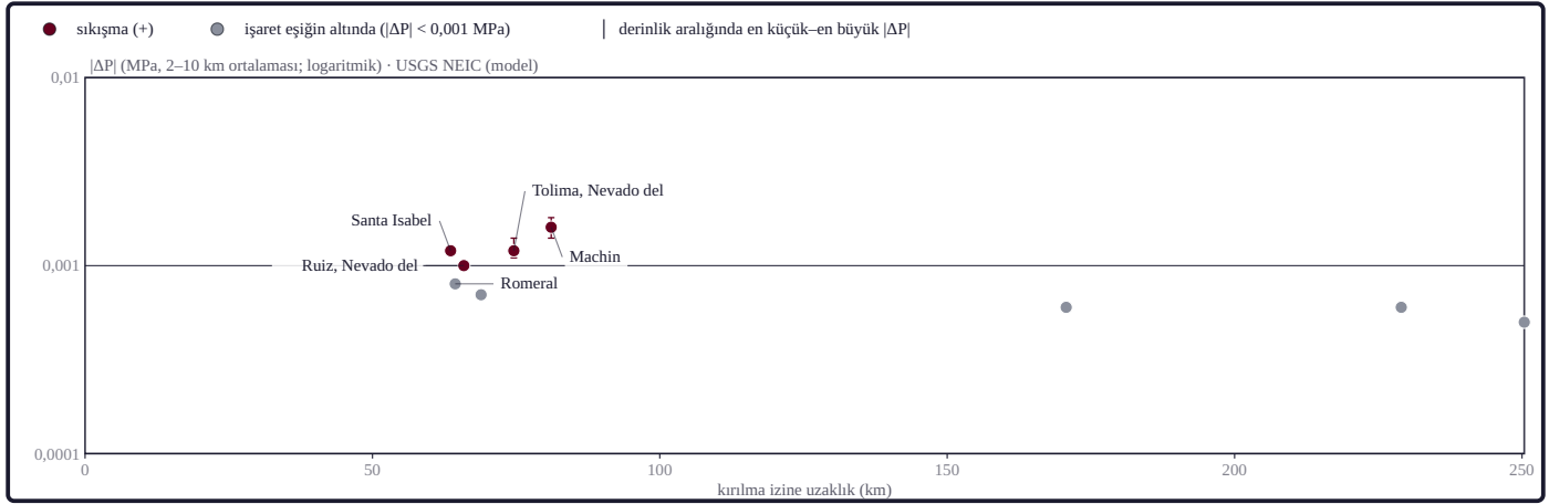
Şekil 12. 9 volkanın kırılma izine uzaklığının göre altındaki eşşismik kaya basıncı değişiminin büyüklüğü ( |\Delta P| , 2–10 km derinlik ortalaması; logaritmik eksen); basınç MODEL çıktısıdır: USGS NEIC kayma modeliyle. Nokta rengi işareti verir: koyu kırmızı sıkışma (+), koyu mavi genişleme (-); |\Delta P| < 0,001 MPa olan 5 volkanın işareti belirsiz sayılır (gri). Dikey çizgi 2–10 km arasındaki derinliklerde en küçük ve en büyük |\Delta P| 'dir. İnce yatay çizgiler logaritmik |\Delta P| ekseninin onluk izgarasıdır; eşik ya da başvuru değeri değildir. Adı yazılanlar |\Delta P| 'si en büyük 5 volkandır. Öbür imler Şekil 11'deki gibidir (volkanlar ve püskürmeler: Global Volcanism Program, Smithsonian Institution; basınç: bu çalışma [model; Okada, 1992]; model: kurum ürünü: USGS NEIC sonlu fay modeli us6000tj2 [U.S. Geological Survey, 2017]).
