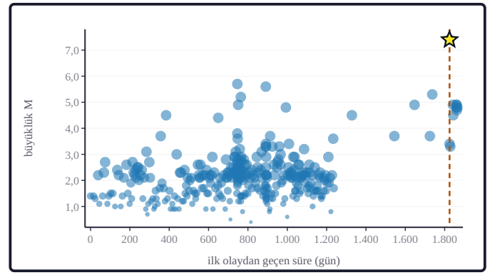
Şekil 2b. Pencere kataloğu 4.626 olaydır (320 olay çizilidir); en büyük olay çalışma olayıdır (Mw 7,4); M_c = 1,7 üstünde 1.855 olay vardır. Büyüklük-zaman dağılımı: yatay eksen ilk olaydan geçen süre (gün), dikey eksen büyüklüktür. Her mavi daire bir olaydır ve daire çapı büyüklükle ölçeklidir; turuncu kesikli dikey çizgi ve yıldız çalışma olayını işaretler (seyreltme eşit adımlıdır; en büyük 10 olay her durumda çizilmiştir).
