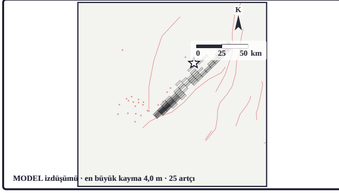
Şekil 13a. Koyu çokgenler USGS sonlu fay modelinin yüzeye izdüşürülmüş yamalarıdır, koyuluk kayma büyüklüğüyle artar; en büyük kaymanın %2'sinin altındaki yamalar çizilmez. Model bir ters çözüm ürünüdür. Kırmızı noktalar bu izdüşümün üzerine bindirilen artçı bulutunu, yani çalışma olayından sonraki katalog olaylarını, beyaz yıldız çalışma olayının dış merkezini, ince çizgiler ise haritalanmış diri fayları gösterir. Uyarı: Bu bir Arazide ÖLÇÜLMÜŞ yüzey kırığı haritası değildir — model izdüşümüdür; arazi ölçümüyle aynı sembolle gösterilmesi modeli gözlem gibi sunmak olurdu. Artçılar da yeniden konumlandırılmamış katalog çözümleridir ve saçılımlarının bir bölümü bölgesel ağ konum belirsizliğinden gelir (Kayma modeli [kurum ürünü]: USGS sonlu fay modeli sürüm 1 [gözden geçirilmiş ürün; 14.08.2026], U.S. Geological Survey, 2017; yöntem Ji vd., 2002 · faylar: GEM Global Active Faults Database [harmonized] [Styron ve Pagani, 2020]).
