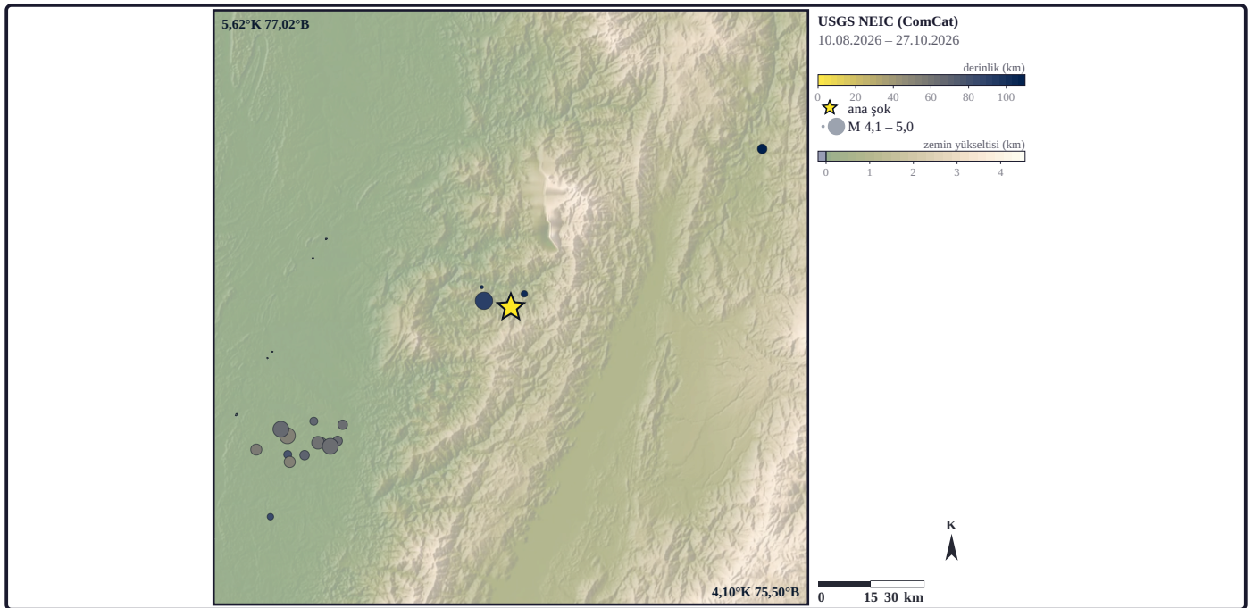
Şekil 4b. Noktalar USGS NEIC (ComCat) kataloğunun kendi raporlarıdır: ana şoktan sonraki 78 gün (10.08.2026 - 27.10.2026), dış merkezin artçı yarıçapı kutusu, n = 17 ; boyut büyüklüğe göre; renk derinliktir (0-110 km; 1 olay daha derin, en koyu renkte); sarı yıldız ana şokun dış merkezidir; sabit olmayan derinliklerin ortancası 66,9 km (çeyrekler 61,9-89,4 km); zemin GMRT gölgeli kabartmasıdır (oleron: mavi tonlar deniz, yeşil-kahve tonlar kara); ince koyu çizgi aynı ızgaranın 0 m eğrisidir (gelgit kıyı çizgisi değildir) (katalog: USGS NEIC [ComCat] [U.S. Geological Survey, 2017]; altlık ve kıyı çizgisi: GMRT v4.5.0 [Ryan vd., 2009; CC BY 4.0] + Mapzen / AWS Terrain Tiles kara yükseltisi [SRTM [USGS], GMTED2010 [USGS]]; renk: oleron [Crameri, 2018a, 2018b]).
