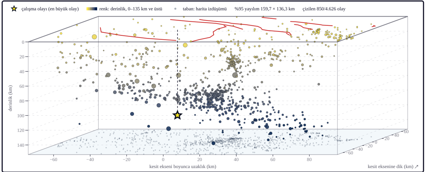
Şekil 4a. Yatay eksen kesit eksen (kutu yayılımının uzun eksen) boyunca, sağ üste kaçan eksen ona dik uzaklığı, düşey eksen derinliği verir. Derinlik eksen kesitlerle ayırılır. Üst yüzdeki kırmızı çizgiler diri fay izleridir; yıldızdan üst yüze çıkan kesikli çizgi olayın yüzeydeki izdüşümünü gösterir (kabinet izdüşümü; üç eksen ayrı ölçeklidir; blok kenarları %95 yayılımın 1,06 katıdır).
