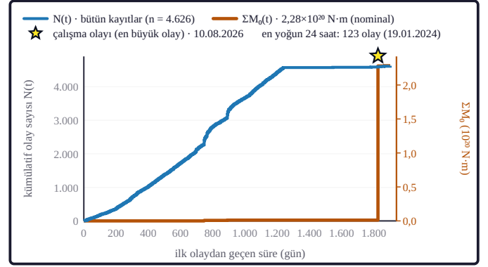
Şekil 5b. Mavi eğri kümülatif olay sayısı N(t) , turuncu eğri kümülatif sismik moment \Sigma M_0(t) değeridir. Sarı yıldız çalışma olayıdır; penceredeki en büyük olay da odur ( M_0 = 10^9[1,5 \cdot M + 9,1] \text{ N} \cdot \text{m} ; 9,1 sabiti Kanamori, 1977).
