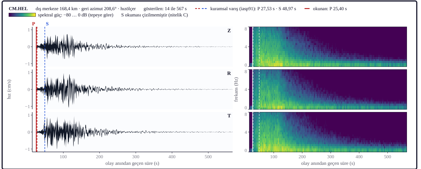
Şekil 15. Solda dalga formu, sağda Hann pencereli kısa zamanlı Fourier spektrogramı (pencere 2,56 s, %50 örtüşme) verilir; P ve S varışları işaretlidir. Şekil kaydın sinyal taşıyan bölümünü gösterir; aralık lejantıdır. Dalga formunda yatay eksen olay anından geçen süre (s), dikey eksen cm/s birimindedir ve bileşenler ortak ölçektedir; spektrogramda dikey eksen frekans (Hz), renk tepeye göre dB'dir ve üç bileşen ortak renk ölçeğindedir. Yatay bileşenler geri azimuta göre ışınsal (R) ve teğetsel (T) bileşene döndürülmüştür. Genlikler cihaz yanıtı giderilerek fiziksel birime çevrilmiştir. Kesikli dikey çizgiler kuramsal P ve S varışlarını, dolu çizgiler kayıttan okunan varışları gösterir. Kuramsal P, okunan P'den yalnız 2,13 s ayrıldığından bu ölçekte dolu çizginin altında kalır. S okuması düşük nitelikli olduğundan çizilmemiştir (kayıt: CM ağı, EarthScope veri merkezi, FDSN dataset; süzgeç: Butterworth bant geçiren, sıfır fazlı, 0,025–8,0 Hz).
