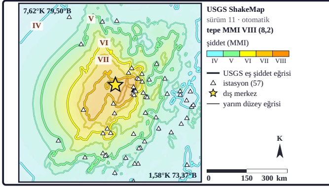
Şekil 14a. Harita USGS ShakeMap model kestiriminin (sürüm 11; otomatik ürün; 11.10.2026) eş şiddet (MMI) eğrilerini gösterir; ince eğriler yarım düzeylerdir; bu sürümde 66 sismik istasyon kaydından işaretlenmeyen 57'si ve 458 şiddet gözleminde işaretlenmeyen 456'sı yer hareketi bağıntılarıyla birlikte kullanılmıştır; dış merkezin 66 km içinde ShakeMap'in kullandığı sismik istasyon kaydı yoktur (USGS belirsizlik derecesi C); üçgenler ShakeMap listesindeki 66 sismik istasyondan kadraj içinde kalan 57'sini gösterir (dolu üçgen: en yüksek PGA); yıldız dış merkezdir; renkli zemin orta çözünürlüklü USGS ShakeMap şiddet ızgarasının her 4. hücresidir; zeminin en büyük değeri 7,8'dir (ürünün beyan ettiği tepe 8,2) (kurum ürünü: USGS ShakeMap; yöntem: Wald ve Worden, 2020; Worden vd., 2018).
