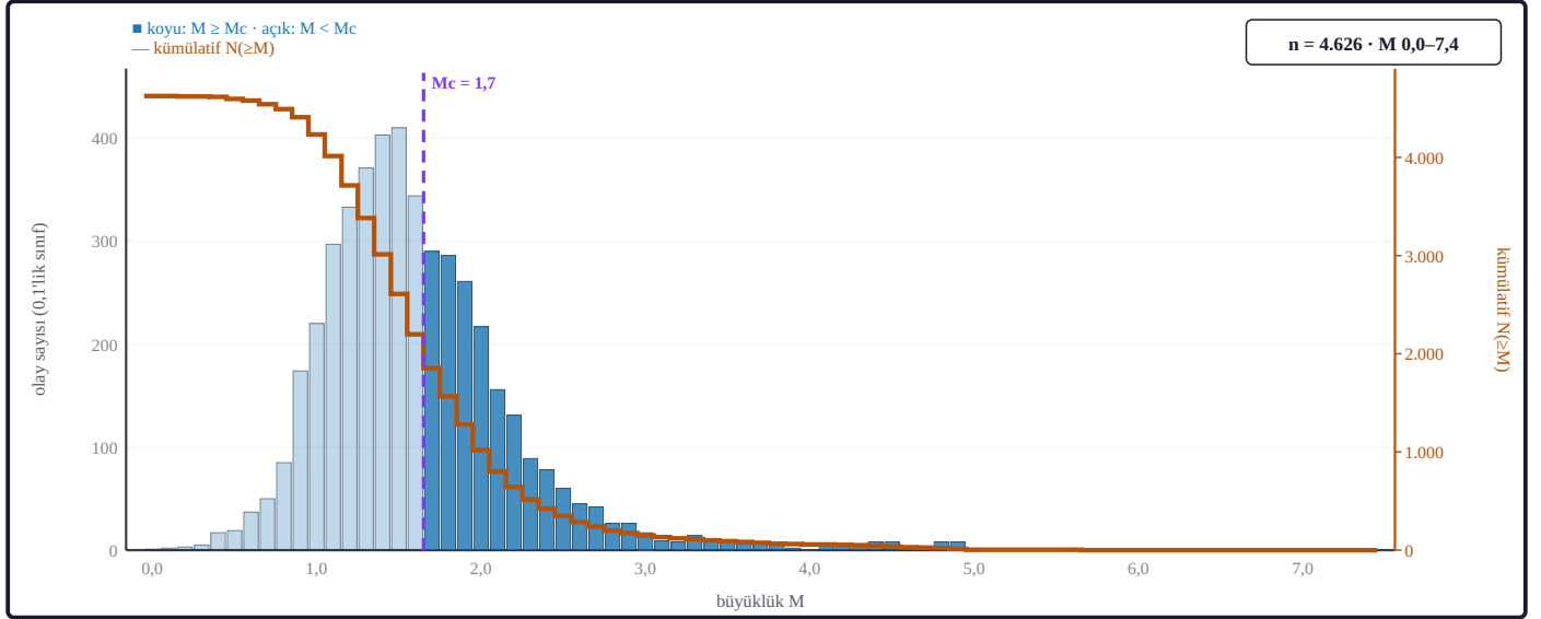
Şekil 17. Pencere kataloğunun tamamında tamlık büyüklüğü M_c = 1,7 olarak benimsenmiştir (azami eğrilik + 0,2 ölçütü); bu eşikte uyum iyiliği %89,7 düzeyindedir; pencerenin en büyük olayı çalışma olayıdır (Mw 7,4). Mavi çubuklar 0,1 genişliğindeki büyüklük sınıflarına düşen olay sayısıdır (sol eksen); turuncu eğri kümülatif N(\geq M) sayımıdır (sağ eksen). Mor kesikli çizgi pencere kataloğunun tamamının tamlık büyüklüğüdür; altındaki sınıflar açık dolguludur (tam katalog, n = 4.626 ).
