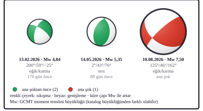
Şekil 6b. Arama penceresindeki (ana şoktan 180 gün önce – 30 gün sonra, 180 km yarıçap) odak mekanizması çözümleri ( n = 3 ) zaman sırasıyla odak küresi olarak verilmiştir. Her küre bir moment tensörü çözümüdür. Küre rengi çözümün ana şoka göre zamanını (yeşil önce, kırmızı ana şok, siyah sonra), çapı büyüklüğü taşır; kürelerin altında tarih, Mw, doğrultu/eğim/kayma açısı, Frohlich ve Apperson (1992) sınıfı ve ana şoka göre süre yazılıdır. Çözüm sayısı 5'ten az olduğundan harita ve P/T eksen stereogramı çizilmemiştir. Arama penceresi raporun analiz penceresinden farklıdır (moment tensörleri ve Mw: Global CMT, Ekström vd., 2012; izdüşüm: Lambert alt yarıküre eşit alan).
