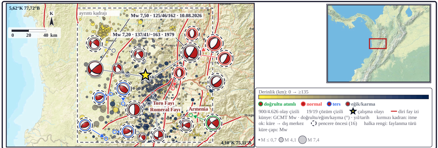
Şekil 18c. Bölgesel odak mekanizması çerçevesi: harita, çevrede yayımlanmış çözümlerin Mw sırasıyla en büyüklerini gösterir; ötelenen küreler okla konumlarına bağlıdır. Küreler alt yarıküre izdüşümünde odak mekanizmalarıdır; kırmızı kadranlar P dalgasının ilk hareketinin itme olduğu bölgelerdir. Mw sırasıyla en büyük 2 çözüm künyelidir (öbür 17 küre künyesizdir); künye çözümün moment büyüklüğünü (GCMT Mw), bir düğüm düzleminin doğrultu, eğim ve kayma açısını ve yılını (çalışma penceresi içindeki çözümlerde tarihini) verir. Küçük daireler pencere olayları, kesikli dikkörtgen ayrıntı haritasının kadrajıdır. Yalnız bu depremle aynı derinlik sınıfındaki (ara derinlik, 70–300 km) 19 çözüm kümeye alınmıştır; başka derinlik sınıfındaki 8 çözüm gösterilmez (mekanizma kümesi: bölgesel küme [ n = 19 ]; bu kümeyle gerilme inversiyonu raporlanmamıştır; faylar: GEM Global Active Faults [Styron ve Pagani, 2020] — CC BY-SA 4.0).
