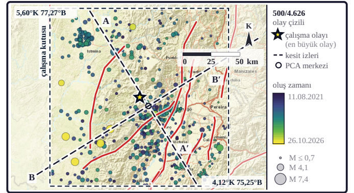
Şekil 3d. Daire rengi oluş zamanını (koyu mor en eski → sarı en yeni), çapı büyüklüğü verir. Öbür imler Şekil 3c'deki gibidir (kesikli dikdörtgen çalışma kutusudur).
