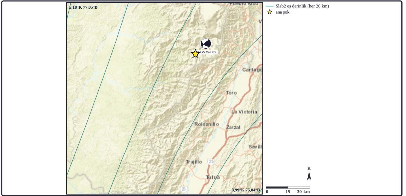
Şekil 7b. Tektonik çerçeve: levha geometrisi: küre ana şokun moment tensörü çözümüdür (kurum ürünü: USGS NEIC W-fazı [Mww]; 124/59/159); ince çizgi dış merkeze bağlar; sarı yıldız ana şoktur; yeşil eğriler Slab2 levha yüzeyinin 20 km aralıklı eş derinlik eğrileridir; dış merkezde yüzey 87,8 \pm 23,5 km derinlikte, 25,7^\circ eğimlidir (Slab2'nin Güney Amerika bölge modeli; Hayes, 2018) (ana şok mekanizması: kurum ürünü: USGS NEIC W-fazı [Mww] [U.S. Geological Survey, 2017]; levha yüzeyi: Slab2 [Hayes, 2018], Seismo Lab hesabı).
