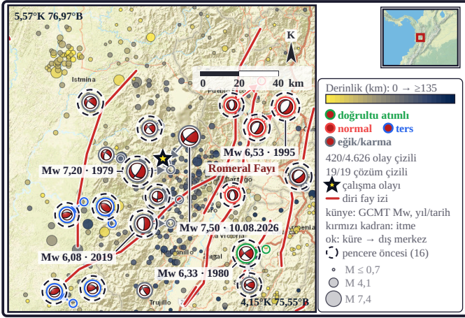
Şekil 1. Harita 4.626 olaylık katalogdan 420 olayı gösterir; odak mekanizmaları 19 çözümlük bölgesel mekanizma kümesindedir. Daire rengi odak derinliğini, çapı büyüklüğü verir; kadranlı kürelere odak mekanizması çözümleridir; kırmızı kadranslar P dalgasının ilk hareketinin itme olduğu bölgelerdir. Sarı yıldız çalışma olayı, kırmızı çizgiler diri fay izleridir. Mw sırasıyla en büyük 5 çözüm künyelidir (öbür 14 küre künyesizdir); künye çözümün Global CMT (GCMT) katalogundaki moment büyüklüğünü (Mw) ve yılını (çalışma penceresi içindeki çözümlerde tarihini) verir; bu büyüklük gövdedeki katalog büyüklüğünden farklı olabilir. İnce çizgi künyeyi küresine, ok küreyi çözümün dış merkezine bağlar. Kesikli halkalı küreler çalışma penceresinden önceki çözümlerdir (faylar: GEM Global Active Faults [Styron ve Pagani, 2020] — CC BY-SA 4.0; mekanizmalar: bölgesel mekanizma kümesi; katalog: ISC · USGS · EMSC · GFZ; altlık: Esri, HERE, Garmin, OSM katkıcıları).
