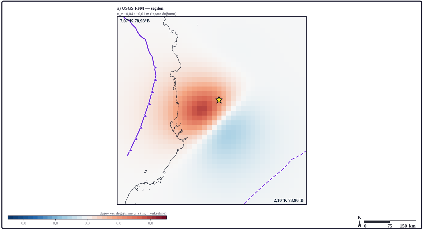
Şekil 13c. Panel kayma modelinden hesaplanan kosismik düşey yer değıştirmedir ( u_z , + yükselme): USGS NEIC us6000tj12 (ürün tarihi 14.08.2026) (seçilen); model ileri hesabı yamaların Okada (1985) yüzey çözümüyle toplamıdır: homojen elastik yarı uzay (katmanlı ortam değil); bütün model değerleri model çıktısıdır; renk ölçeği seçilen modelin tepesine göre \pm 0,05 m'de doyar; panel kendi uçlarını (kaba ızgara düğümünde) yazar (model: kurum ürünü: USGS NEIC sonlu fay modeli us6000tj12 [U.S. Geological Survey, 2017]; yöntem: Okada, 1985; kıyı çizgisi [0 m eğrisi]: GMRT v4.5.0 [Ryan vd., 2009; CC BY 4.0; çok-ışınlı olmayan hücrelerde GEBCO] + Mapzen / AWS Terrain Tiles kara yükseltisi [SRTM [USGS], GMTED2010 [USGS]]).
