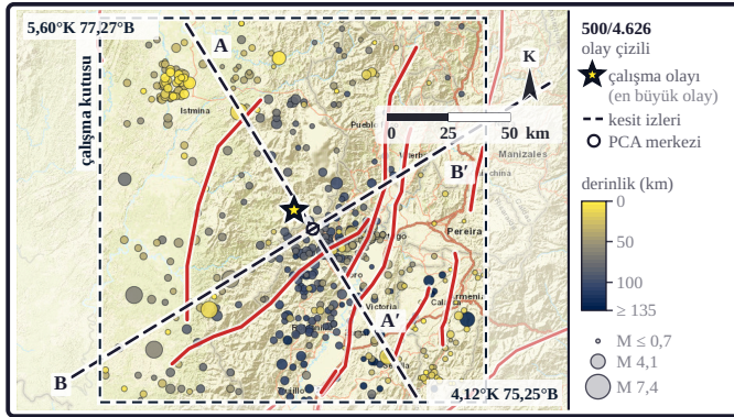
Şekil 3c. Derinlik renkli harita 4.626 olaylık katalogdan 500 olayı gösterir. Daire rengi odak derinliğini, çapı büyüklüğü verir. Sarı yıldız çalışma olayıdır; kesikli A–A' ve B–B' doğruları kesitlerin harita izleridir (kesikli dikdörtgen çalışma kutusudur; kutunun dışı sorgulanmamıştır; oradaki fay izleri bağlam içindir).
