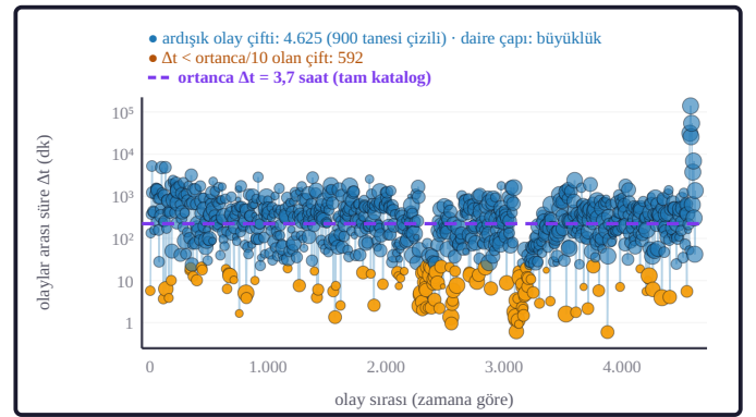
Şekil 5d. Düşey eksen bir önceki olaydan geçen süredir (dakika, logaritmik). Mor çizgi ortalanca süredir; turuncu daireler ortalancanın onda birinden kısa aralıklardır. Daire çapı büyüklükle artar (seri: tekilleştirilmiş tam katalog).
