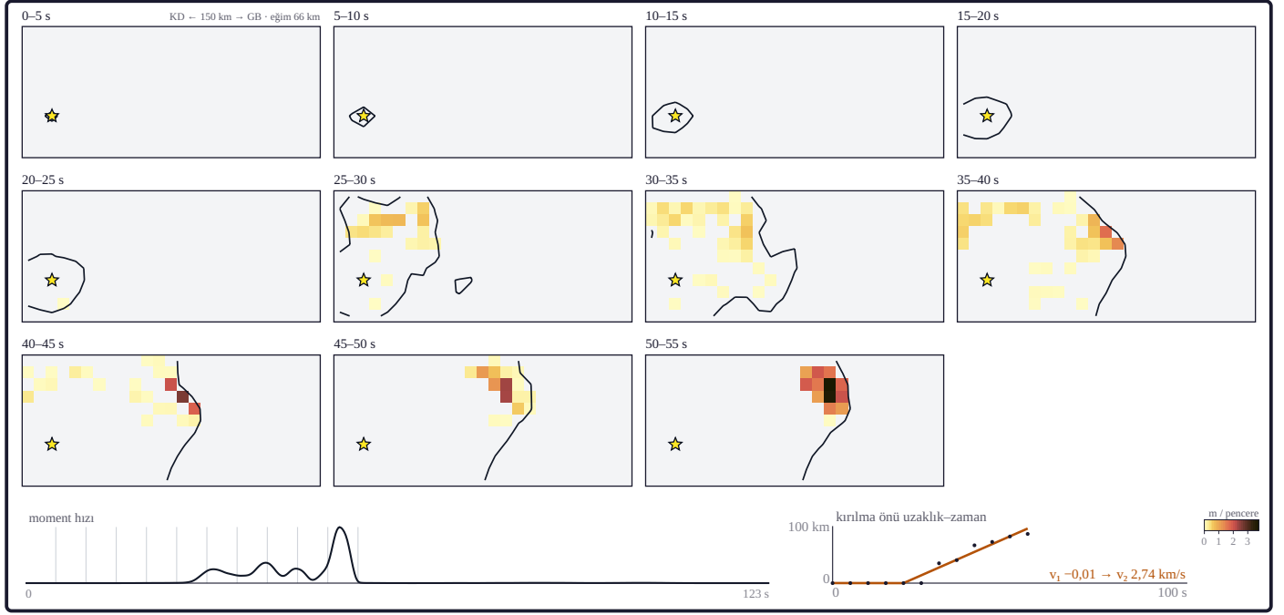
Şekil 9. Kırılma anlık görüntüleri: USGS NEIC us6000tjl2 (ürün tarihi 14.08.2026) kayma modelinin açılmış fay düzleminde (yatay doğrultu boyunca, düşey eğim aşağı) 11 ardışık 5 s'lik pencerede açığa çıkan kayma; renk pencere içindeki kaymadır (ortak ölçek 0–3,8 m; model çıktısı); 55 s'den sonra toplam kaymanın %1,7'si (momentin %1,7'si) açığa çıkar; panolardaki kayma ile bu kalan pay toplam kaymayı verir (fark %0,0); kaynak zaman işlevi yama başına yükselme ve düşme süreli asimetrik kosinüstür (modelin kendi parametreleri); siyah eğri pencere sonu kırılma önu; küçük pano kırılma önu uzaklık-zaman: v_1 -0,01 \rightarrow v_2 2,74 \text{ km/s} (model: kurum ürünü: USGS NEIC sonlu fay modeli us6000tjl2 [U.S. Geological Survey, 2017]; yöntem: bu çalışma [açılmış düzlem, pencere integrali]; renk: lajolla [Crameri, 2018]).
