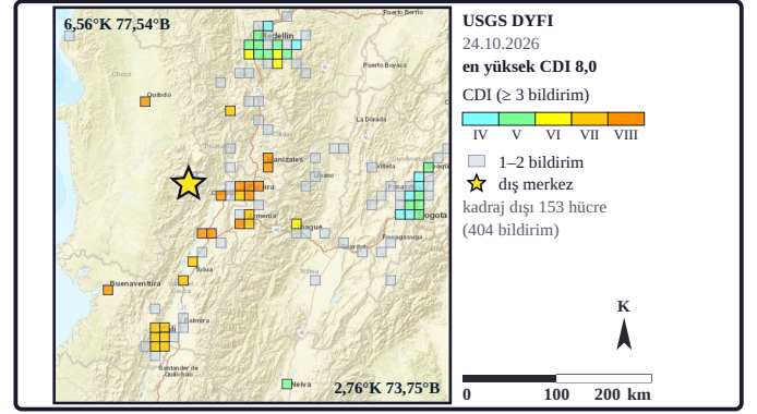
Şekil 14b. Harita USGS “Did You Feel It?” (DYFI) ürününün (24.10.2026) 10 km'lik hücrelerindeki topluluk şiddetini (CDI) gösterir; CDI hücresindeki bildirimlerden hesaplanan gözlem değeridir; ürünün 1.253 bildiriminin 1.230'u 260 hücrededir; renkli hücreler en az 3 bildirimli 79 hücredir ve rengi CDI değerinin en yakın tam şiddet düzeyidir; bunlarda en yüksek CDI 8,0 (Dosquebradas, 41 bildirim, hücre merkezi dış merkeze 64 km); kadraj dışında 153 hücre (31'i renkli, 16'sı şüpheli; 404 bildirim) kalır; dış merkeze en uzak renkli hücre 1.213 km uzaktadır; gri hücreler 1–2 bildirimlidir ve renklendirilmemiştir; yıldız çalışma olayının dış merkezidir; altlık: Sources: Esri, HERE, Garmin, © OpenStreetMap contributors, and the GIS user community (veri: USGS “Did You Feel It?” [DYFI]; yöntem: Wald vd., 2011; eşik: Atkinson ve Wald, 2007; yer adları: GeoNames [geonames.org], CC BY 4.0, erişim 26.10.2026).
