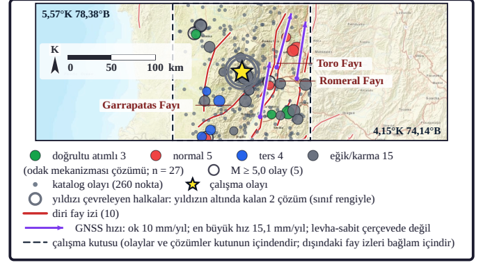
Şekil 13b. Haritada odak mekanizması çözümleri, diri fay izleri ve GNSS hız vektörleri birlikte gösterilmiştir. Renkli dairelerde renk mekanizma sınıfını, çap büyüklüğü kodlar. Kırmızı çizgiler haritalanmış diri fay izleridir; dış merkeze en yakın adlı faylar harita üzerinde adlandırılmıştır. Mor oklar GNSS istasyonlarının yatay hız vektörleridir (başvuru oku ve en büyük hız lejjantıdır). İçi boş halkalar M \geq 5,0 olayları, küçük gri noktalar katalog sismisitesini, sarı yıldız çalışma olayının dış merkezini gösterir (GCMT mekanizmaları; GNSS: Nevada Geodetic Laboratory [NGL] MIDAS hızları, Blewitt vd., 2016, 2018; hızlar levha-sabit çerçevede değildir, levha-görelî hareket olarak okunamaz; faylar: GEM Global Active Faults [Styron ve Pagani, 2020] — CC BY-SA 4.0).
