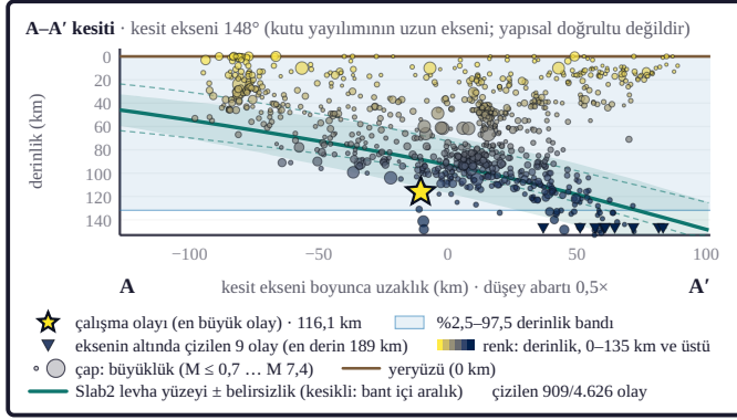
Şekil 3a. Olayların %95'i 0,0–131,8 km derinlik bandındadır; ortalama derinlik 56,0 km'dir (sabit atamalar dışlanınca 61,0 km). A–A' kesiti olayları kesit eksenini (kutu yayılımının uzun eksenini) boyunca uzanan düşey düzleme izdüşürür. Sarı yıldız çalışma olayıdır; daire rengi derinliği, çapı büyüklüğü verir. Alt kenardaki üçgenler derinlik ekseninin altında kalan olaylardır. Kesikli yatay çizgi kurumların varsayılan olarak atadığı sabit derinliktir. A–A' ve B–B' kesitleri aynı yatay açıklık ve aynı derinlik eksenine çizilmiştir (izdüşüm: çalışma kutusundaki olayların çizim örneği; derinlikler katalog hiposantrlarıdır; levha yüzeyi: Slab2 [Hayes, 2018], Seismo Lab hesabı).
