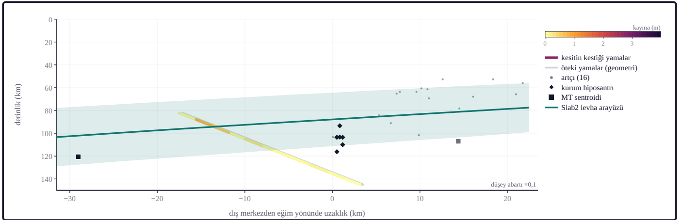
Şekil 8b. Kesit dış merkezden geçen ve USGS NEIC us6000tjl2 (ürün tarihi 14.08.2026) modelinin temsili doğrultusuna ( 226^\circ ) dik düşey düzlemdir; yatay eksen eğim yönünde ( 316^\circ ) uzaklıktır, eksi değerler eğim yukarıdır; şerit modelin doğrultu boyunca kapladığı 150 km'dir; renkli doğru parçaları modelin kesit düzleminin kestiği 11 yamasıdır (doğrultu boyunca dış merkezden uzaklığı yama yarı boyundan küçük olanlar; renk kayma, 0–4,0 m; model çıktısı); açık gri parçalar şeritteki öteki 264 yamanın eğim yönündeki izdüşümüdür (yalnız geometri); noktalar artçılar (16); elmaslar kurum hiposantr derinlikleri (içi boş: sabit / bağımlı) (model: kurum ürünü: USGS NEIC sonlu fay modeli us6000tjl2 [U.S. Geological Survey, 2017]; artçılar: USGS NEIC [ComCat] [U.S. Geological Survey, 2017]; levha yüzeyi: Slab2 [Hayes, 2018], Seismo Lab hesabı).
