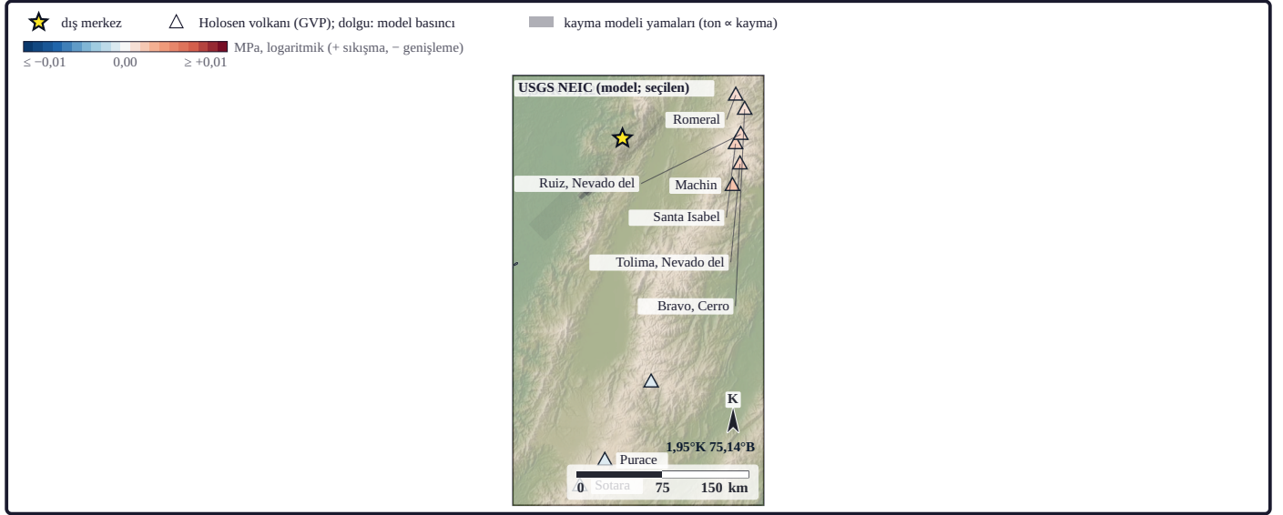
Şekil 11. 9 Holosen volkanı (GVP; min(dış merkez, kırılma izi) ≤ 300 km; aday kümesi USGS NEIC kırılma iziyle kurulmuştur). Üçgen dolgu volkanın altında 2–10 km derinlikteki eşismik kaya basıncı değişiminin ortalamasıdır ( P = -(\sigma_1 + \sigma_2 + \sigma_3)/3 ; + sıkışma, - genişleme; renk işaretli logaritmik ölçekte ( \pm 0,01 MPa'ya dek doğrusala yakın), \pm 0,01 MPa'da doyun); basınç MODEL çıktısıdır: USGS NEIC, kamu malı (USGS) kayma modelleriyle ( \mu = 30 GPa, \nu = 0,25 ). Basınç homojen elastik yarı uzay varsayımıyla Okada (1992) çözümünden hesaplanmıştır; topoğrafya ve katmanlı ortam yoktur. Gri tonlu dörtgenler panel modelinin yamalarının yüzey izdüşümüdür (ton kaymayla orantılı). Zemin GMRT gölgeli kabartmasıdır (oleron: mavi tonlar deniz, yeşil-kahve tonlar kara); ince koyu çizgi aynı ızgaranın 0 m eğrisidir (gelgit kıyı çizgisi değildir) (volkanlar ve püskürmeler: Global Volcanism Program, Smithsonian Institution; basınç: bu çalışma [model; Okada, 1992]; model: kurum ürünü: USGS NEIC sonlu fay modeli us6000tjl2 [U.S. Geological Survey, 2017]; altlık ve kıyı çizgisi: GMRT v4.5.0 [Ryan vd., 2009; CC BY 4.0; çok-ışınlı olmayan hücrelerde GEBCO] + Mapzen / AWS Terrain Tiles kara yükseltisi [SRTM [USGS], GMTED2010 [USGS]]; renk: oleron [Cramer, 2018a, 2018b]).
