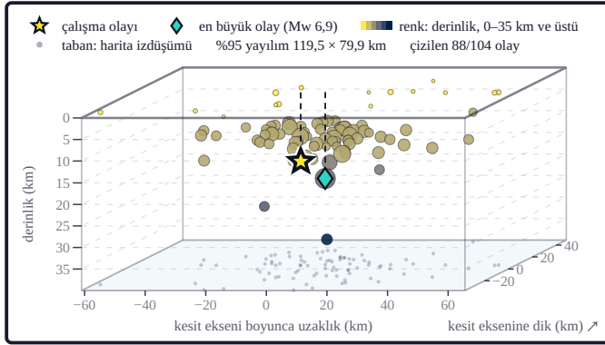
Şekil 3c. Yatay eksen kesit eksenini (kutu yayılımının uzun eksenini) boyunca, sağ üste kaçan eksen ona dik uzaklığı, düşey eksen derinliği verir. Derinlik eksenini kesitlerle ayırır. Yıldızdan ve elmaştan üst yüze çıkan kesikli çizgiler olayların yüzeydeki izdüşümünü gösterir (kabinet izdüşümü; üç eksen ayrı ölçeklidir; blok kenarları %95 yayılımını 1,06 katır).
