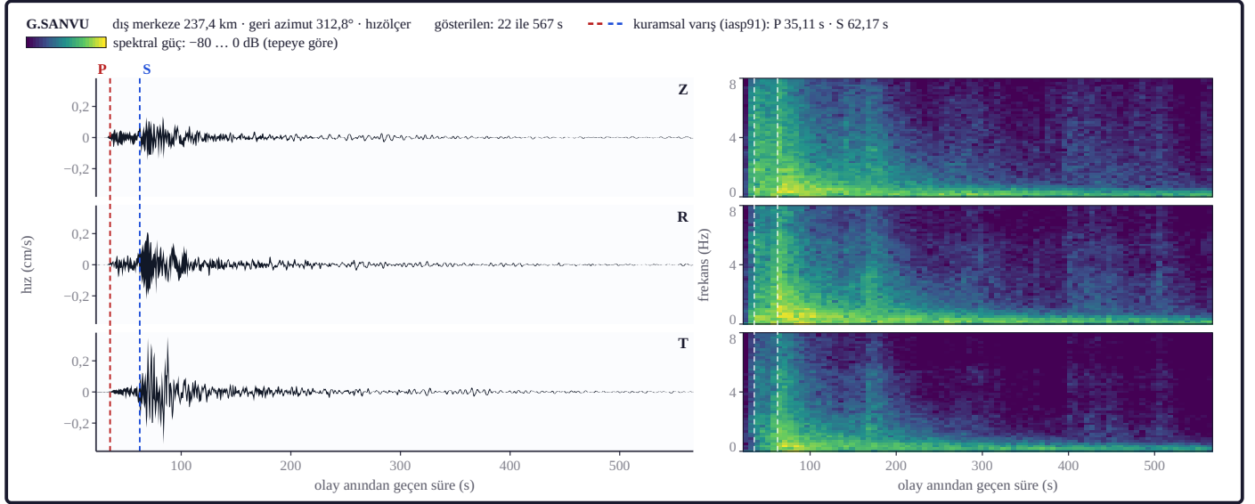
Şekil 8a. Solda dalga formu, sağda Hann pencereli kısa zamanlı Fourier spektrogramı (pencere 12,80 s, %50 örtüşme) verilir; P ve S varışları işaretlidir. Şekil kaydın sinyal taşıyan bölümünü gösterir; aralık lejantıdır. Dalga formunda yatay eksen olay anından geçen süre (s), dikey eksen cm/s birimindedir ve bileşenler ortak ölçektedir; spektrogramda dikey eksen frekans (Hz), renk tepeye göre dB'dir ve üç bileşen ortak renk ölçeğindedir. Yatay bileşenler geri azimuta göre ırsal (R) ve teğetsel (T) bileşene döndürülmüştür. Genlikler cihaz yanıtı giderilerek fiziksel birime çevrilmiştir. Kesikli dikey çizgiler kuramsal P ve S varışlarını gösterir (kayıt: G ağı, EarthScope veri merkezi, FDSN dataset; süzgeç: Butterworth bant geçiren, sıfır fazlı, 0,025–8,0 Hz).
