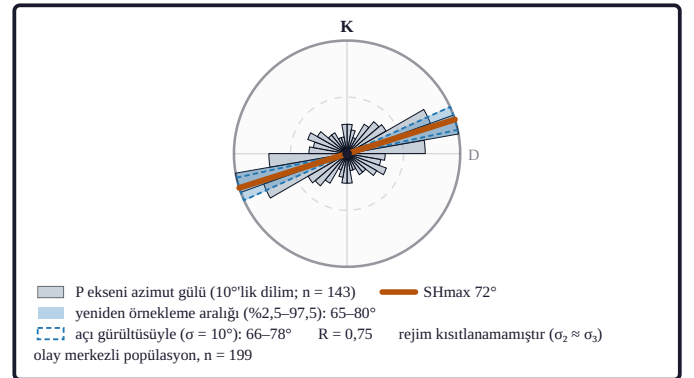
Şekil 6d. Çekinceli çözüm: SH_{max} = 72^\circ ; rejim sınıfı kısıtlanamamıştır ( R = 0,75 ; olay merkezli mekanizma popülasyonunun gerilme inversiyonu). Kuzeyi yukarıda olan gül diyagramında turuncu çift uçlu eksen gerilme inversiyonundan bulunan SH_{max} azimutunu, mavi yelpaze bu azimutun %2,5–97,5 yüzdelik aralığını (eksenel olduğundan karşı ucuyla birlikte) gösterir. Kesikli mavi sınır, her mekanizmanın doğrultu, eğim ve kayma açısına \sigma = 10^\circ 'lik rastgele gürültü de eklenerek yinelenen tersininin aynı yüzdelik aralığıdır (Vavryčuk, 2014). Gri sektörler bölgesel mekanizma kümesinin P eksen (kısılma) azimut gülüdür ( 10^\circ 'lik dilimler; yarıçap sayımın kareköküyle orantılı). İç kesikli çember yarı ölçek halkasıdır; şekil oranı R ve rejim sınıfı lejantta (SHmax yönü: Lund ve Townend, 2007; rejim sınıfı: Dünya Gerilme Haritası kuralı).
