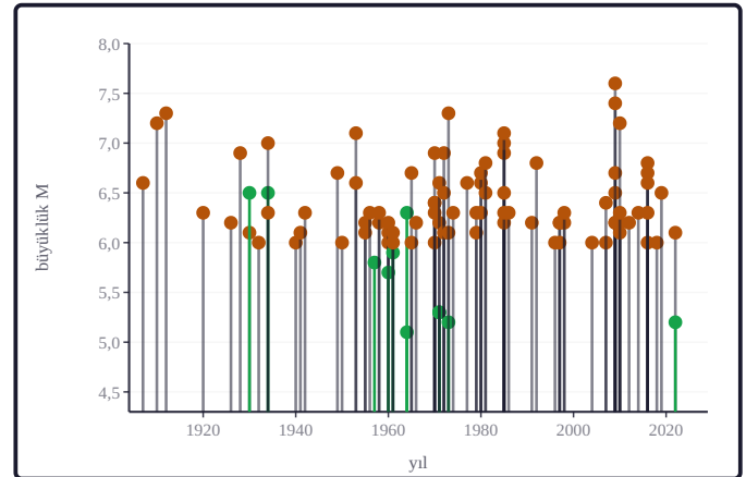
Şekil 13b. Tarihsel çişik üstü depremlerin büyüklükleri yıllara göre çizilmiştir; yeşil yakın kuşak, turuncu bölge kuşağıdır; sap rengi aynı ayrımı verir (yeşil sap yakın kuşak, gri sap bölge kuşağı) (birleşik katalog, 1900 sonrası; büyüklükler, varsa ISC-GEM Mw: International Seismological Centre, 2026; Di Giacomo vd., 2015, 2018).
