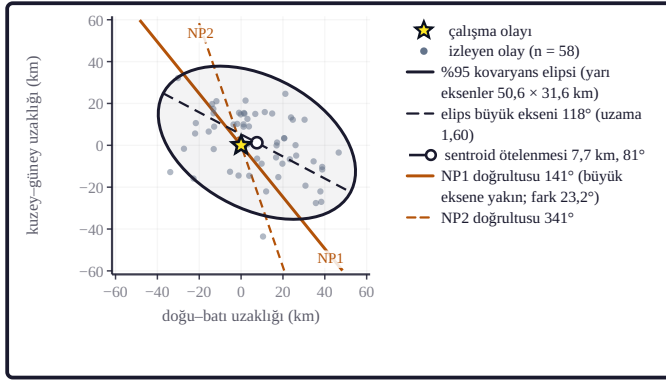
Şekil 6a. Çalışma olayına göre yerel yatay düzlemde (doğu ve kuzey artı, km; iki eksen aynı ölçekte) izleyen olay bulutu gri noktalarla, %95 kovaryans elipsi koyu çizgiyle gösterilmiştir; elips bulutun ağırlık merkezine oturur ve yıldız çalışma olayıdır. Kesikli koyu doğru elipsin büyük eksenidir; çalışma olayından çıkan ince çizgi ve içi boş daire izleyen olayların sentroidinin ötelenmesidir. Turuncu doğrular çalışma olayının düğüm düzlemlerinin doğrultularıdır; büyük eksene doğrultuca yakın olan düz, öteki kesikli çizilmiştir. Uzama oranı 1'e yaklaştıkça bulut izotroplaşır ve yön kestirimi zayıflar; elips ölçüleri lejantta (telesismik ikinci moment ölçüsünün izleyen olay konumlarına uyarlanmış vekili: McGuire vd., 2002).
