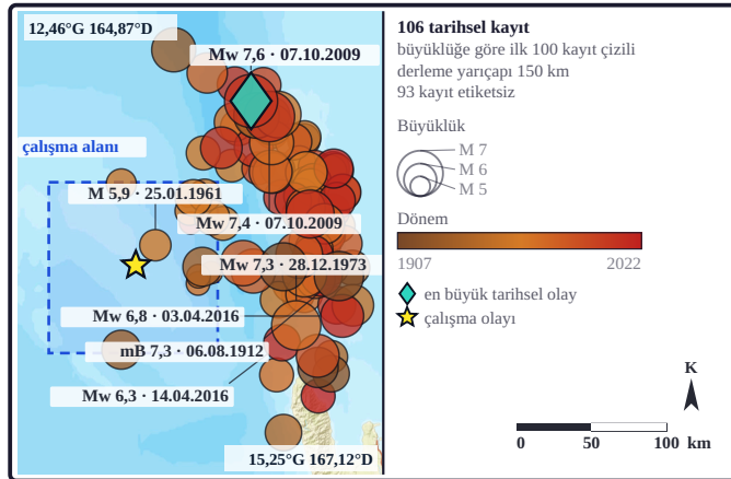
Şekil 13a. Çalışma olayından önceki eşik üstü kayıtlarda daire çapı büyüklüğü, dolgu rengi oluş dönemini gösterir. Turkvaz elmas derlemenin en büyük kaydı, sarı yıldız çalışma olayıdır. Kayıt eşiği yakın kuşakta M \geq 5 , bölge kuşağında M \geq 6 olarak alınmıştır. Mavi kesikli dikdörtgen çalışma alanıdır (birleşik katalog, 1900 sonrası; derleme yarıçapı 150 km, yakın kuşak 60 km).
