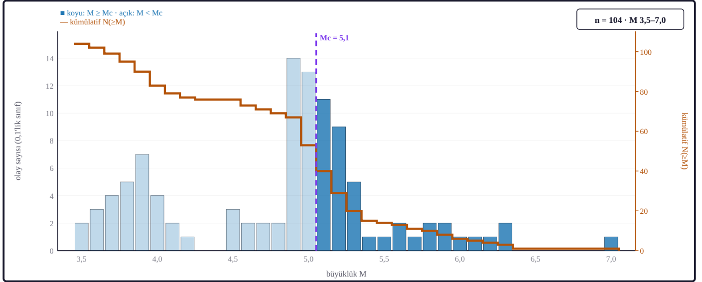
Şekil 12. Pencere kataloğunun tamamında tamlık büyüklüğü M_c = 5,1 olarak benimsenmiştir (azami eğrilik + 0,2 ölçütü); bu eşikte uyum iyiliği %84,9 düzeyindedir; pencerenin en büyük olayı M 7,0 büyüklüğündedir. Mavi çubuklar 0,1 genişliğindeki büyüklük sınıflarına düşen olay sayısıdır (sol eksen); turuncu eğri kümülatif N(\geq M) sayımıdır (sağ eksen). Mor kesikli çizgi pencere kataloğunun tamamının tamlık büyüklüğüdür; altındaki sınıflar açık dolgudur (tam katalog, n = 104 ).
