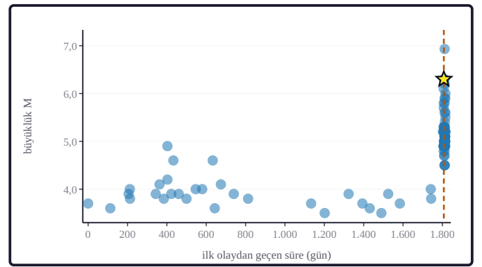
Şekil 2b. Pencere kataloğu 104 olaydır; en büyük olay Mw 6,9 büyüklüğündedir (24.10.2026); M_c = 5,1 üstünde 40 olay vardır. Büyüklük-zaman dağılımı: yatay eksen ilk olaydan geçen süre (gün), düşey eksen büyüklüktür. Her mavi daire bir olaydır ve daire çapı büyüklükle ölçeklidir; turuncu kesikli düşey çizgi ve yıldız çalışma olayını işaretler.
