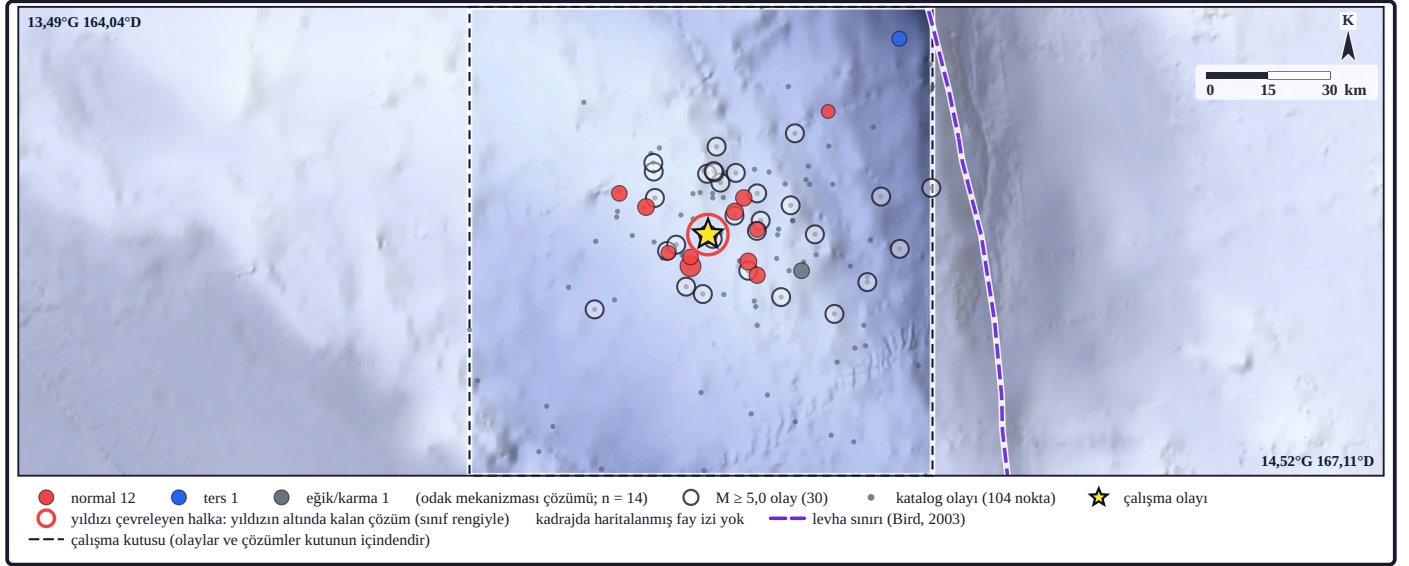
Şekil 10. Haritada odak mekanizması çözümleri gösterilmiştir. Renkli dairelerde renk mekanizma sınıfını, çap büyüklüğü kodlar. İçi boş halkalar M \geq 5,0 olayları, küçük gri noktalar katalog sismisitesini, sarı yıldız çalışma olayının dış merkezini gösterir; kesikli mor çizgiler Bird (2003) levha sınırlarıdır (GCMT mekanizmaları; levha sınırları: Bird, 2003).
