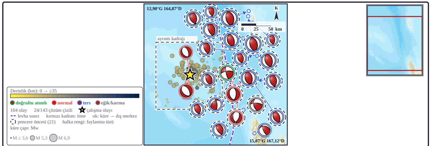
Şekil 13c. Bölgesel odak mekanizması çerçevesi: harita, çevrede yayımlanmış çözümlerin Mw sırasıyla en büyüklüklerini gösterir; ötelenen küreler okla konumlarına bağlıdır. Küreler alt yarıküre izdüşümünde odak mekanizmalarıdır; kırmızı kadrantlar P dalgasının ilk hareketinin itme olduğu bölgelerdir. Küreler künyesizdir. Küçük daireler pencere olayları, kesikli dikdörtgen ayrıntı haritasının kadrajıdır (mekanizma kümesi: bölgesel küme [ n = 143 ]; gerilme inversiyonu olay merkezli mekanizma popülasyonundandır [ n = 199 ]; haritalanmış fay izi yok; mor kesik: levha sınırı [Bird 2003]).
