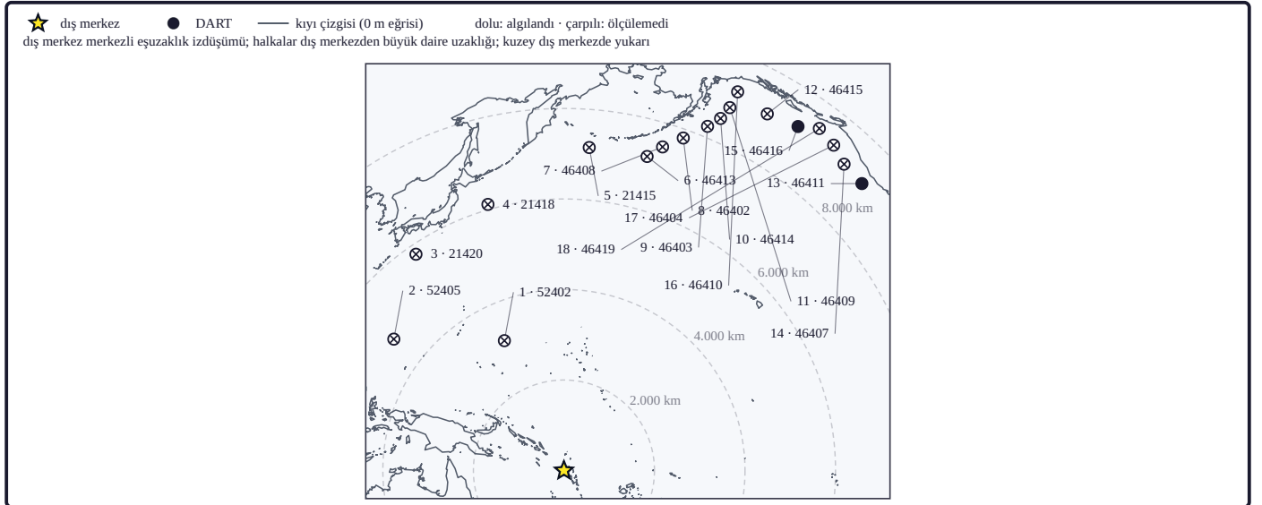
Şekil 8b. Tsunami gözlem istasyonlarının konumu: 18 DART (2 algıladı, 16 ölçülemedi); en uzak istasyon 9.432 km. Konumlar IOC SLSMF istasyon kaydındaki güncel konuşturmalarıdır (olay günündeki konum farklı olabilir). Ölçüm durumları bu çalışmanın ölçümüdür; DART kayıt kesiti ve DART çizelgesiyle aynı ölçümden gelir. DART etiketindeki ilk sayı dış merkez uzaklığına göre sıradır; DART kayıt kesitinde ve DART çizelgesinde aynı sıra kullanılır. Harita dış merkez merkezli eşuzaklık izdüşümüdür; halkalar dış merkezden büyük daire uzaklığıdır, yön yalnız dış merkezde geçerlidir; ince gri çizgi ETOPO 2022 ızgarasının ( \approx 7 km hücre) 0 m eğrisidir (kıyı; gelgit kıyı çizgisi değildir; hücreden küçük adalar çizilemez) (konum: IOC Sea Level Station Monitoring Facility istasyon kaydı; ölçüm: NOAA NDBC DART, işlem bu çalışma; kıyı çizgisi [0 m eğrisi]: ETOPO 2022 [60" ızgara, 4 hücrede bir, NOAA NCEI, doi:10.25921/fd45-gt74]).
