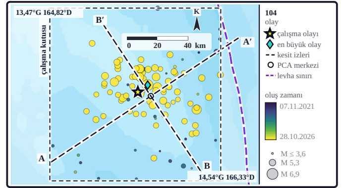
Şekil 11d. Daire rengi oluş zamanını (koyu mor en eski → sarı en yeni), çapı büyüklüğü verir. Öbür imler Şekil 4'teki gibidir (kesikli dikdörtgen çalışma kutusudur).
