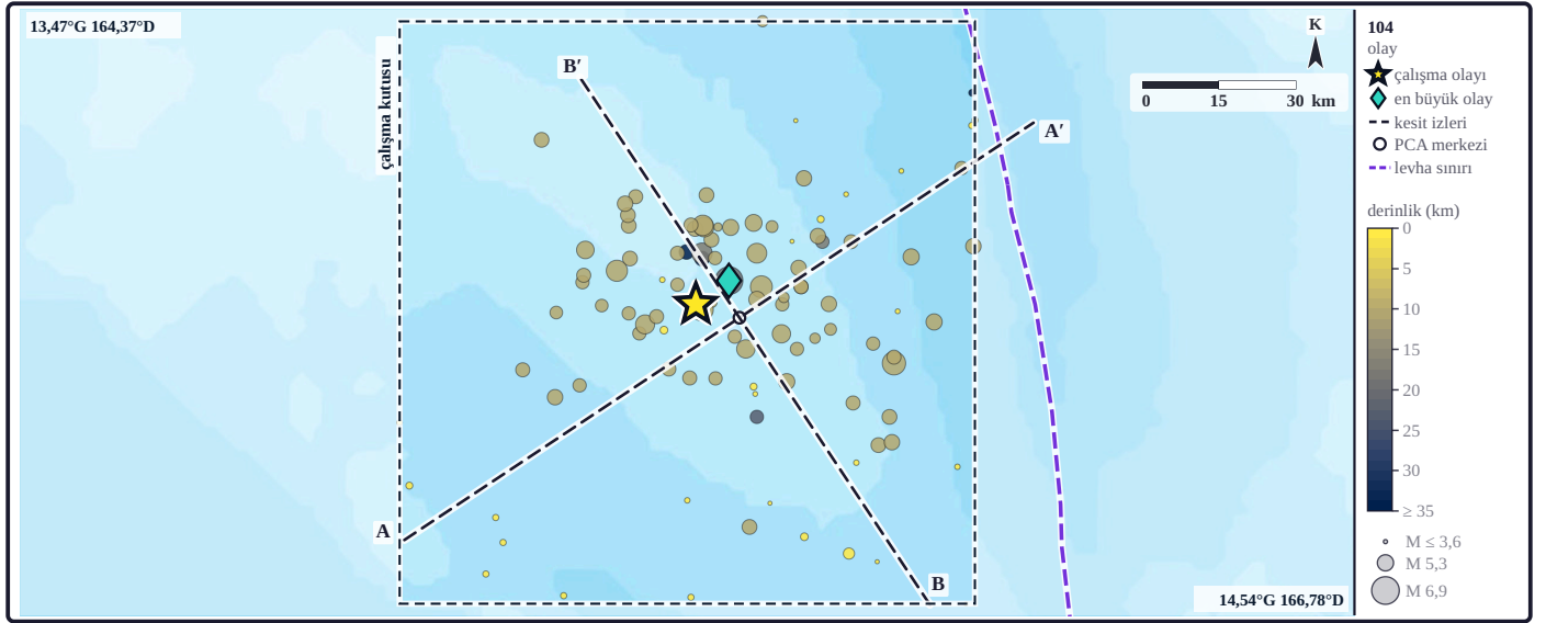
Şekil 4. Derinlik renkli harita 104 olaylık kataloğun tamamını gösterir. Daire rengi odak derinliğini, çapı büyüklüğü verir. Sarı yıldız çalışma olayıdır; kesikli A-A' ve B-B' doğruları kesitlerin harita izleridir (kesikli dikdörtgen çalışma kutusudur; kutunun dışı sorgulanmamıştır).
