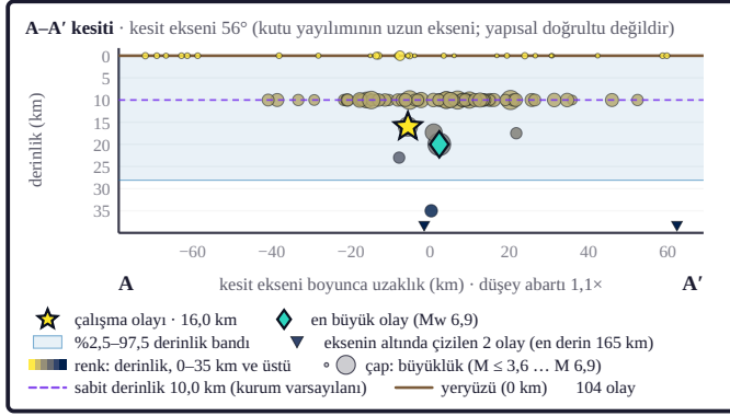
Şekil 3a. Olayların %95'i 0,0–28,1 km derinlik bandındadır; ortanca derinlik 10,0 km'dir (sabit atamalar dışlanınca 21,5 km). A–A' kesiti olayları kesit eksenini (kutu yayılımının uzun eksenini) boyunca uzanan düşey düzleme izdüşürür. Sarı yıldız çalışma olayıdır; daire rengi derinliği, çapı büyüklüğü verir. Alt kenardaki üçgenler derinlik ekseninin altında kalan olaylardır. Kesikli yatay çizgi kurumların varsayılan olarak atadığı sabit derinliktir. A–A' ve B–B' kesitleri aynı yatay açıklık ve aynı derinlik eksenine çizilmiştir (izdüşüm: çalışma kutusundaki bütün olaylar; derinlikler katalog hiposantrlarıdır).
