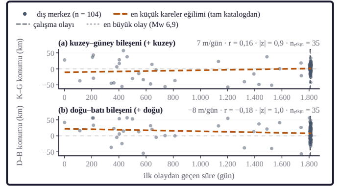
Şekil 3d. Dış merkez koordinatlarının zaman serisi iki şeritte verilmiştir: (a) kuzey–güney, (b) doğu–batı bileşeni. Düşey eksen pencere kutusunun merkezine uzaklıktır (km; kuzey ve doğu artı) ve iki şerit aynı ölçektedir; yatay eksen penceresinin ilk olayından geçen süredir (gün). Turuncu kesikli doğrular iki bileşenin en küçük kareler eğilimidir; eğim, Pearson korelasyon katsayısı ve etkin örneklem büyüklüğüyle hesaplanan Fisher z değeri şerit başlığındadır. Kesikli düşey çizgi çalışma olayının, noktali düşey çizgi pencerenin en büyük olayının anını işaretler.
