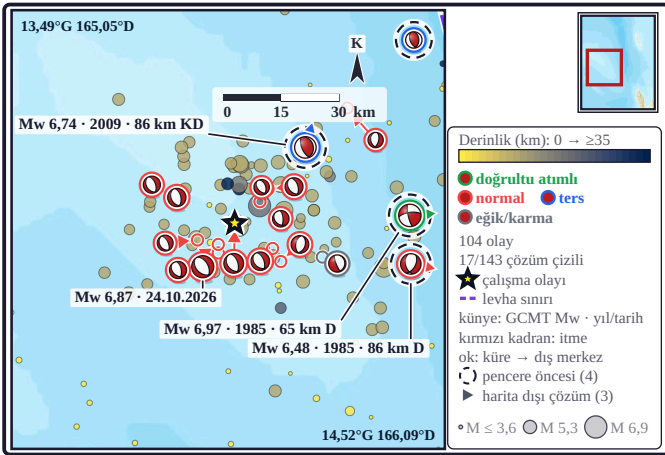
Şekil 1. Harita 104 olaylık kataloğun tamamını gösterir; odak mekanizmaları 143 çözümlük bölgesel mekanizma kümesindendir. Gerilme inversiyonu olay merkezli mekanizma popülasyonundandır ( n = 199 ). Daire rengi odak derinliğini, çapı büyüklüğü verir (haritalanmış fay izi yok; mor kesik: levha sınırı [Bird 2003]; mekanizmalar: bölgesel mekanizma kümesi; katalog: ISC · USGS · EMSC · GFZ; altlık: Batimetri: GMRT v4.5.0 [Global Multi-Resolution Topography] — Ryan, W.B.F. ve ark., 2009, Geochem. Geophys. Geosyst. 10, Q03014, doi:10.1029/2008GC002332 · Lamont-Doherty Earth Observatory / MGDS, CC-BY-4.0 · Renk skalası: oleron [bilimsel, sıfır-çapalı] — Crameri, F. [2018] Zenodo doi:10.5281/zenodo.1243862 · Crameri [2018] Geosci. Model Dev. 11, 2541–2562 · Crameri, Shephard & Heron [2020] Nature Communications 11, 5444 · Batimetri: GMRT v4.5.0 [Global Multi-Resolution Topography] — Ryan, W.B.F. ve ark., 2009, Geochem. Geophys. Geosyst. 10, Q03014, doi:10.1029/2008GC002332 · Lamont-Doherty Earth Observatory / MGDS, CC-BY-4.0 · Kabartma: AWS Terrain Tiles [Mapzen terrarium] — kaynak ve lisanslar: github.com/tilezen/joerd/blob/master/docs/attribution.md ).
