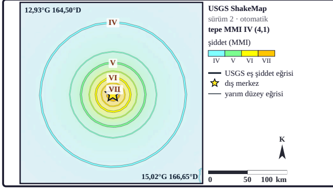
Şekil 7a. Harita USGS ShakeMap model kestiriminin (sürüm 2; otomatik ürün; 20.10.2026) eş şiddet (MMI) eğrilerini gösterir; ince eğriler yarım düzeylerdir; bu sürümde sismik istasyon kaydı yoktur; alan yalnız yer hareketi bağıntılarından kurulmuştur; USGS belirsizlik derecesi --; yıldız dış merkezdir; renkli zemin orta çözünürlüklü USGS ShakeMap şiddet ızgarasının her 2. hücresidir; zeminin en büyük değeri 7,2'dir (ürünün beyan ettiği tepe 4,1) (kurum ürünü: USGS ShakeMap; yöntem: Wald ve Worden, 2020; Worden vd., 2018).
