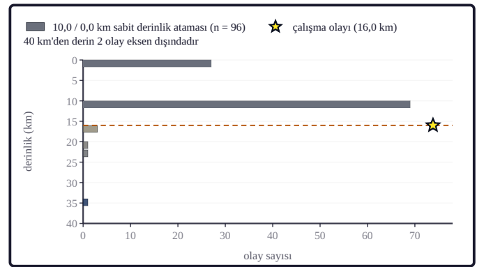
Şekil 2d. Tam katalogta derinlik değeri taşıyan 104 olayın %92'si \leq 10 km derinliktedir. Sabit derinlik atamaları (10,0 km) ölçülmüş derinlik taşımaz. Hiposantr derinlik histogramı (tam katalog): çubuk rengi derinliği gösterir (sığ sarı, derin lacivert); koyu kesim sabit derinlik atamalarıdır; yıldız ve kesikli çizgi çalışma olayının derinliğidir.
