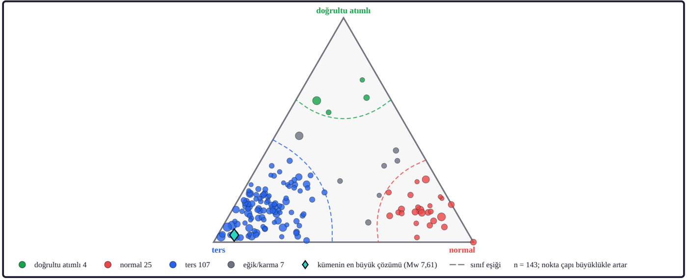
Şekil 7c. Çekinceli sayım: 143 çözümün %75'i ters sınıfındadır (%95 Wilson aralığı %62–84; 54 bağımsız küme). Alt uç %70 baskınlık eşliğinin altında kaldığından tek sınıflı niteleme yapılmamıştır. Bağımsız kümeler Gardner–Knopoff pencereleriyle ayrılmıştır. Frohlich üçgeninde her nokta bir odak mekanizması çözümünün P, T ve B eksenlerinin dalım açılarından gnomonik izdüşümle kurulan konumudur (köşeler: ters, normal, doğrultu atımlı). Renkli kesikli eğriler sınıf eşikleridir (B dalımı 60°, P dalımı 60°, T dalımı 50°); nokta rengi sınıfı, gri renk hiçbir eşiği aşmayan eğik/karma çözümleri, nokta çapı büyüklüğü, turkuaz elmas kümedeki en büyük çözümü gösterir; sınıf sayımları lejantadır (Frohlich, 1992 gnomonik üçgeni; Frohlich ve Apperson, 1992 eşikleri; çözümler: Global CMT, Ekström vd., 2012).
