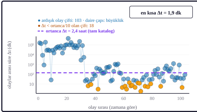
Şekil 11c. Düşey eksen bir önceki olaydan geçen süredir (dakika, logaritmik). Mor çizgi ortalanca süredir; turuncu daireler ortalancanın onda birinden kısa aralıklardır. Daire çapı büyüklükle artar (seri: tekilleştirilmiş tam katalog).
