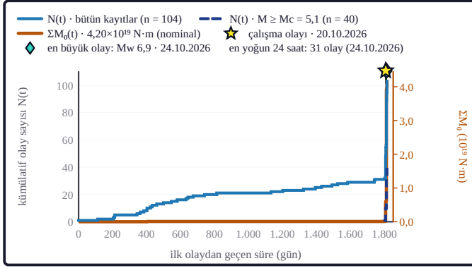
Şekil 11a. Mavi eğri kümülatif olay sayısı N(t) , turuncu eğri kümülatif sismik moment \Sigma M_0(t) değeridir. Sarı yıldız çalışma olayını, turkuaz elmas penceredeki en büyük olayı işaretler ( M_0 = 10^{(1,5 \cdot M + 9,1)} N·m; 9,1 sabiti Kanamori, 1977).
