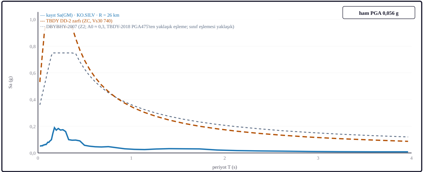
Şekil 8c. Yatay eksen periyot T (s), dikey eksen %5 sönümlü spektral ivme S_a (g), mavi eğri kayıt, turuncu kesikli eğri tasarım zarfıdır. Şekil kaydedilen yer hareketinin tepki spektrumunu tasarım zarfıyla karşılaştırır, mavi eğri en yakın ivme-ölçer istasyonunun iki yatay bileşeninin geometrik ortalaması S_a(T) , turuncu kesikli eğri aynı sahanın zemin sınıfı ve harita spektral ivme katsayılarıyla kurulan TBDY DD-2 tasarım spektrumu, gri noktalı eğri varsa 2007 deprem yönetmeliğinin (DBYBHY-2007) karşılığıdır; mavi eğrinin turuncu zarfı aştığı periyot bandı, o periyoda denk yapı stoğu için tasarım düzeyinin aşıldığı banttır ( S_a : Newmark- \beta SDOF çözümü, Newmark, 1959; TBDY 2018 tasarım spektrumu; gri eğri: DBYBHY-2007, Bayındırlık ve İskân Bakanlığı; kayıt: FDSN ham ivme).
