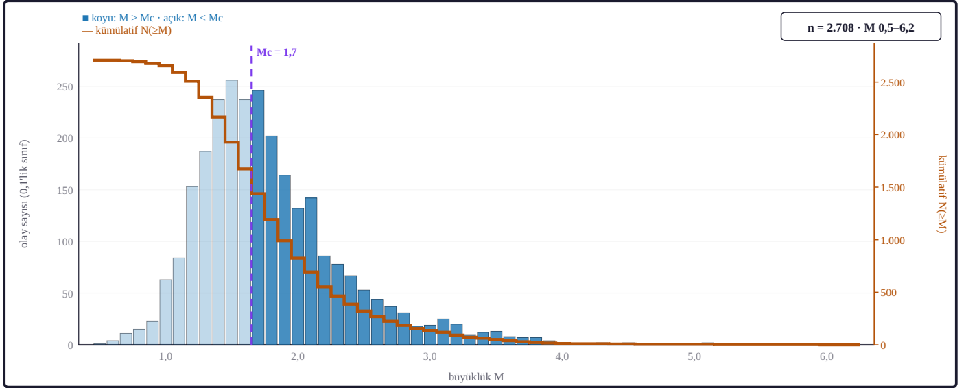
Şekil 12. Tamlık büyüklüğü M_c = 1,7 olarak benimsenmiştir (b-kararlılığı ölçütü); bu eşikte uyum iyiliği %98,4 düzeyindedir; pencerenin en büyük olayı çalışma olayıdır (Mw 6,2). Mavi çubuklar 0,1 genişliğindeki büyüklük sınıflarına düşen olay sayısıdır (sol eksen); turuncu eğri kümülatif N(\geq M) sayımıdır (sağ eksen). Mor kesikli çizgi tamlık büyüklüğüdür; altındaki sınıflar açık dolguludur ve b değeri kestirimine girmez (tam katalog, n = 2.708 ).
