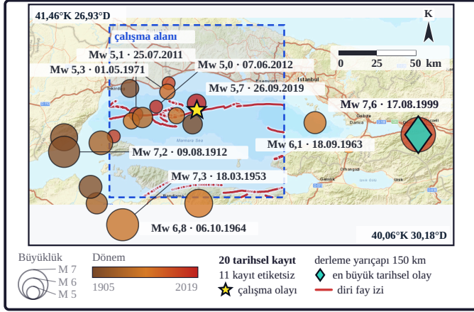
Şekil 13a. Çalışma olayından önceki eşik üstü kayıtlarda daire çapı büyüklüğü, dolgu rengi oluş dönemini gösterir. Turkuaz elmas derlemenin en büyük kaydı, sarı yıldız çalışma olayıdır. Kayıt eşiği yakın kuşakta M \geq 5 , bölge kuşağında M \geq 6 olarak alınmıştır. Mavi kesikli dikdörtgen çalışma alanıdır (birleşik katalog, 1900 sonrası; derleme yarıçapı 150 km, yakın kuşak 60 km).
