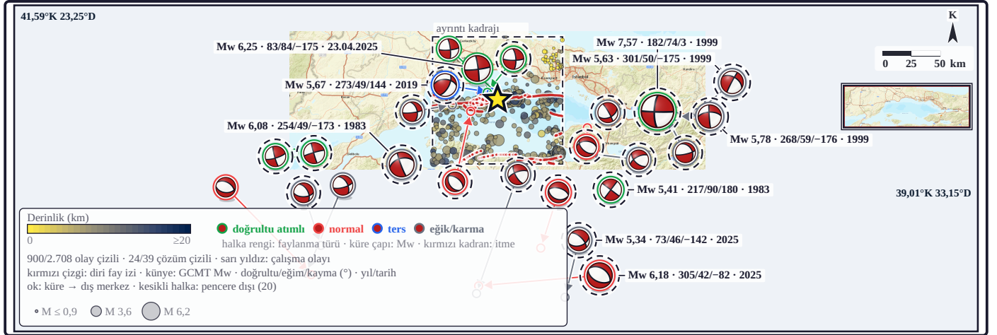
Şekil 13c. Bölgesel odak mekanizması çerçevesi: harita, çevrede yayımlanmış çözümlerin Mw sırasıyla en büyüklerini gösterir; ötelenen küreler okla konumlarına bağlıdır. Küreler alt yarıküre izdüşümünde odak mekanizmalarıdır; kırmızı kadrantlar P dalgasının ilk hareketinin itme olduğu bölgelerdir. Mw sırasıyla en büyük 9 çözüm künyelidir (öbür 15 küre künyesizdir); künye çözümün moment büyüklüğünü (GCMT Mw), bir düğüm düzleminin doğrultu, eğim ve kayma açısını ve yılını (çalışma penceresi içindeki çözümlerde tarihini) verir. Küçük daireler pencere olayları, kesikli dikdörtgen ayrıntı haritasının kadrājıdır (mekanizma kümesi: bölgesel küme [ n = 39 ]; gerilme inversiyonu olay merkezli mekanizma popülasyonundandır [ n = 15 ]; faylar: MTA TDFH-2026 [Elmacı vd., 2026]).
