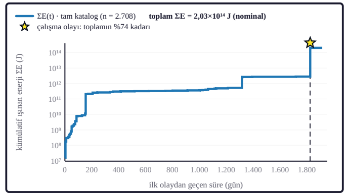
Şekil 9d. Mavi basamak eğrisi kümülatif ışınan sismik enerjidir ( \Sigma E , logaritmik eksen). Kesikli düşey çizgi çalışma olayını işaretler; en büyük tek katkı bu olaydır (Gutenberg ve Richter, 1956 enerji bağıntısı).
