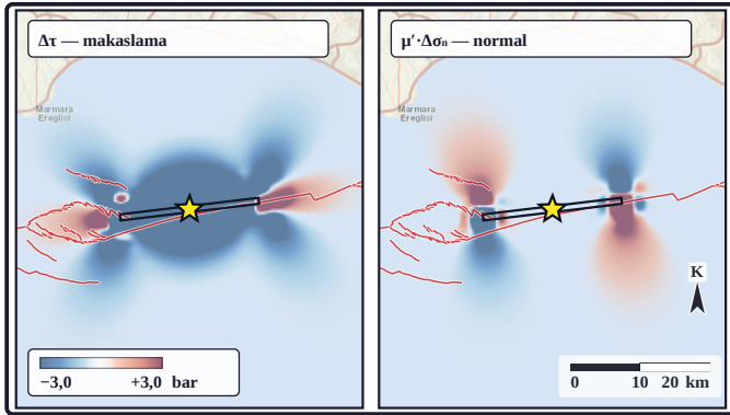
Şekil 5c. \Delta CFS 'in iki bileşeni ayrı panellerde gösterilmiştir: solda makaslama gerilmesi değişimi \Delta\tau , sağda fay düzlemine dik normal gerilme katkısı \mu'\Delta\sigma_n ( \Delta CFS = \Delta\tau + \mu'\Delta\sigma_n ; \Delta\sigma_n çekme artı, artı değer fayın ketetlenmesinin azalmasıdır). Kadraj kaynak çevresine yakınlaştırılmıştır; renk ölçeği ve kaynak geometrisi \Delta CFS haritasıyla aynıdır; yıldız dış merkezdir; ince dörtgen kaynağın yüzey izdüşümüdür (bileşen ayrışımı: Okada, 1992 analitik çözümü).
