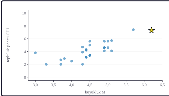
Şekil 7c. Bölgedeki depremlerin topluluk şiddeti (CDI) büyüklüklerine karşı çizilmiştir; yıldız çalışma olayının bildirim kaydını (veri: USGS "Did You Feel It?" [DYFI]; yöntem: Atkinson ve Wald, 2007).
