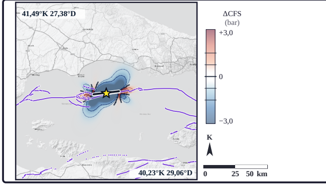
Şekil 5a. Harita statik Coulomb gerilme değişimini ( \Delta CFS ) gösterir (kırmızı artış, mavi azalma; \pm 3,0 bar). \Delta CFS Wells ve Coppersmith (1994) kaynağının kaynakla eş yönelimli alıcıda ( s/d/r = 83^\circ/84^\circ/-175^\circ ), 12,0 km derinlikte, \mu' = 0,40 ile hesaplanmıştır. Yıldız dış merkezdir; dörtgen kaynağın yüzey izdüşümüdür (kalın kenar üstte); çizgiler \Delta CFS konturlarıdır. Mor çizgiler diri fay izleridir; renk çubuğundaki çentikler kontur düzeyleridir; altlık gri tonludur, renkler yalnız \Delta CFS 'indir ( \Delta CFS : Okada, 1992; King vd., 1994; altlık [gri tonlu]: Esri, HERE, Garmin, © OpenStreetMap contributors, and the GIS user community; diri faylar: MTA TDFH-2026 [Elmacı vd., 2026]).
