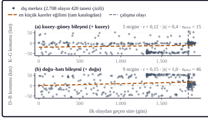
Şekil 9a. Dış merkez koordinatlarının zaman serisi iki şeritte verilmiştir: (a) kuzey-güney, (b) doğu-batı bileşeni. Düşey eksen pencere kutusunun merkezine uzaklıktır (km; kuzey ve doğu artı) ve iki şerit aynı ölçektedir; yatay eksen pencerenin ilk olayından geçen süredir (gün). Turuncu kesikli doğrular iki bileşenin en küçük kareler eğilimidir; eğim, Pearson korelasyon katsayısı ve etkin örneklem büyüklüğüyle hesaplanan Fisher z değeri şerit başlığındadır. Kesikli düşey çizgi çalışma olayının anını işaretler.
