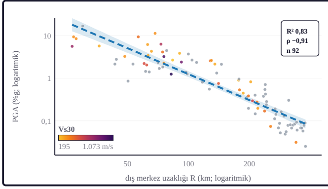
Şekil 8a. Her iki eksen de logaritmiktir, yatay eksen dış merkez uzaklığı R (km), dikey eksen PGA gösterir. Figür, kayıt istasyonlarında ölçülen en büyük yatay yer ivmesinin (PGA) dış merkez uzaklığıyla azalmasını verir ve PGA birimi eksen başlığında yazılmıştır. Küçük daireler gözlemdir; her biri bir kuvvetli yer hareketi kayıdır ve dolgu rengi o istasyonun Vs30 değerini kodlar — açık kehribar yumuşak zemin (düşük Vs30), koyu mor sağlam kaya (yüksek Vs30), gri ise Vs30 ölçümü olmayan istasyondur ve rampanın hiçbir ucuna atanmaz; renk ölçeği sol alttaki şeritte, uçlarındaki sayılar veri aralığının gerçek Vs30 sınırlarıdır. Kesikli mavi doğru modeldir: \log \text{PGA} = a + b \cdot \log R biçiminde en küçük karelerle oturtulan azalım bağıntısı; çevresindeki soluk mavi kuşak bu doğrunun %95 güven bandıdır ve çözümün döndürdüğü band dizisinden olduğu gibi çizilir, yeniden hesaplanmaz (Azalım regresyonu: log-log en küçük kareler + t-kuantili %95 güven bandı [Joyner ve Boore, 1981 geleneği] · sıra korelasyonu: Spearman, 1904 · Vs30/zemin sınıfı: TADAS-AFAD istasyon tablosu).
