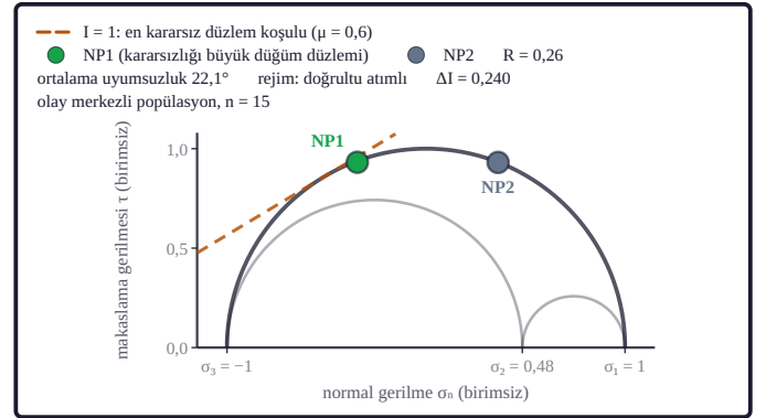
Şekil 5d. Gerilme inversiyonunun normalleştirilmiş Mohr diyagramında yatay eksen normal gerilme \sigma_n , düşey eksen makaslama gerilmesi \tau 'dur. Üç yarım çember asal gerilmelerle kurulan durumunu, turuncu kesikli doğru \mu sürtünme katsayısıyla tanımlı en kararsız düzlem koşulunu (kararsızlık indeksi I = 1 ) gösterir; iki nokta çalışma olayının iki düğüm düzleminin ( \sigma_n, \tau ) konumudur ve doğruya yakın olan düzlem bu gerilme alanında kaymaya daha yatkındır. Şekil oranı R , ortalama kayma yönü uyumsuzluğu ve iki düzlemin kararsızlık farkı \Delta I lejantıdır (Vavryčuk, 2014; kararsızlık ölçütü).
