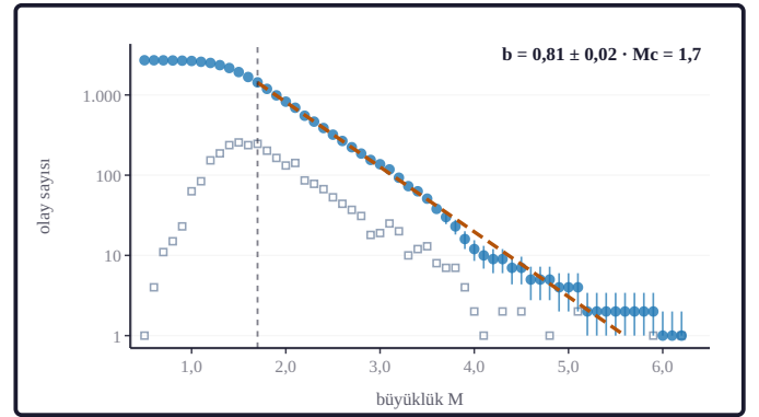
Şekil 2d. Mc = 1,7 (b-kararlılığı) üstündeki 1.437 olaydan b = 0,81 ± 0,02 kestirilmiştir. Gutenberg-Richter büyüklük-frekans dağılımı: dolu daireler kümülatif sayımı N(≥M), açık gri kareler her büyüklük aralığındaki artımsal sayımı verir; kesikli turuncu doğru, benimsenen eşiğin üstünde log 10 N = a - b·M ile çizilen uyum doğrusudur; gri kesikli dikey çizgi tamlık büyüklüğü Mc'dir; ince dikey çubuklar N ≤ 30 olan aralıklarda √N Poisson belirsizliğidir (dağılım: Gutenberg ve Richter, 1944).
