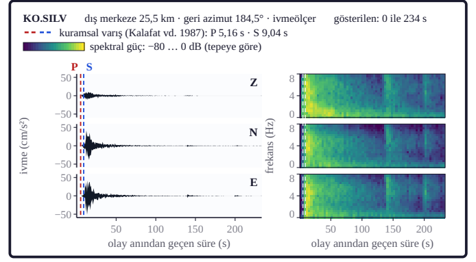
Şekil 8b. Solda dalga formu, sağda Hann pencereli kısa zamanlı Fourier spektrogramı (pencere 2,56 s, %50 örtüşme) verilir; P ve S varışları işaretlidir. Şekil kaydın sinyal taşıyan bölümünü gösterir; aralık lejantıdır. Dalga formunda yatay eksen olay anından geçen süre (s), dikey eksen \text{cm/s}^2 birimindedir ve bileşenler ortak ölçektedir; spektrogramda dikey eksen frekans (Hz), renk tepeye göre dB'dir ve üç bileşen ortak renk ölçeğindedir. Yatay bileşenlerin yönelimi bilinmediğinden döndürme yapılmamış, bileşenler kanal adlarıyla verilmiştir. Genlikler cihaz yanıtı giderilerek fiziksel birime çevrilmiştir. Kesikli dikey çizgiler kuramsal P ve S varışlarını gösterir (kayıt: KO ağı, KOERI veri merkezi, FDSN dataset; süzgeç: Butterworth bant geçiren, sıfır fazlı, 0,025–8,0 Hz).
