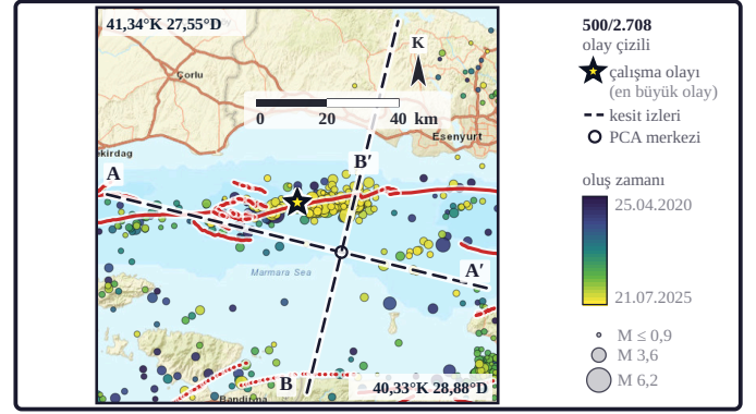
Şekil 10b. Daire rengi oluş zamanını (koyu mor en eski → sarı en yeni), çapı büyüklüğü verir. Öbür imler Şekil 4'teki gibidir.
