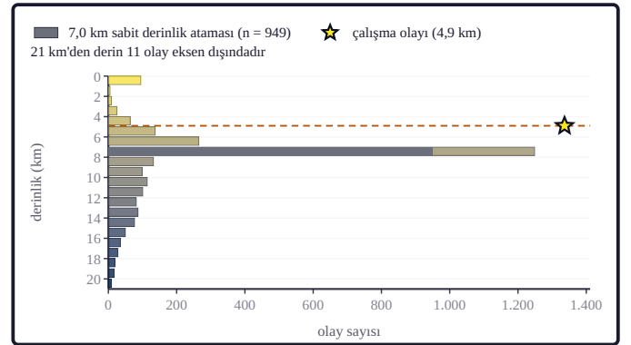
Şekil 3d. Tam katalogta derinlik değeri taşıyan 2.708 olayın %77'si ≤ 10 km derinliktedir. Sabit derinlik atamaları (7,0 km) ölçülmüş derinlik taşımaz. Hiposantr derinlik histogramı (tam katalog): çubuk rengi derinliği gösterir (sığ sarı, derin lacivert); koyu kesim sabit derinlik atamalarıdır; yıldız ve kesikli çizgi çalışma olayının derinliğidir.
