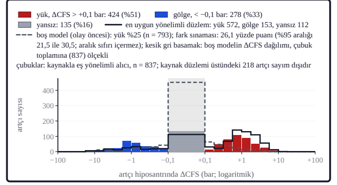
Şekil 5b. Coulomb nokta sınaması, artçıların kendi hiposantrlarında hesaplanan \Delta CFS değerlerinin dağılımını verir. Artçı konum belirsizliği sayılarına yansıtılmamıştır. Kırmızı çubuklar yük artışı, mavi çubuklar gerilme gölgesini, gri bant iki eşik arasındaki yansız aralığı gösterir; siyah çizgi en uygun yönelimli düzlem için aynı dağılımdır; kesik gri basamak, boş modelin çubuk toplamına (837) ölçekli çubuklar: kaynakla eş yönelimli alıcı, n = 837 ; kaynak düzlemi üstündeki 218 artçı sayım dışıdır
