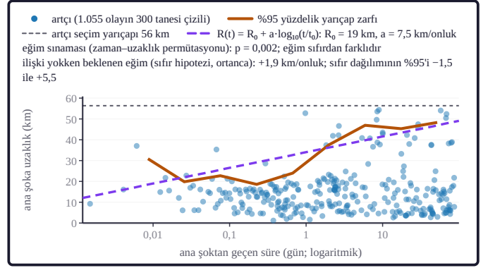
Şekil 9b. Mavi noktalar artçıların ana şoka uzaklığını ana şoktan geçen süreye karşı gösterir (yatay eksen logaritmiktir). Turuncu eğri logaritmik zaman kutularında hesaplanan %95 yüzdelik yarıçap zarfıdır. Kesikli yatay çizgi artçıların seçildiği yarıçaptır; uzaklıklar bu sınırı aşamaz. Mor kesikli doğru zarfa oturtulan R(t) = R_0 + a \cdot \log_{10}(t/t_0) modelidir; katsayılar ve eğim sınavının ölçüsü lejantta (logaritmik zamanda genişleme deseni; zarf %95 yüzdelik).
