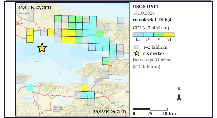
Şekil 7d. Harita USGS "Did You Feel It?" (DYFI) ürününün (14.10.2026) 10 km'lik hücrelerindeki topluluk şiddetini (CDI) gösterir; CDI hücredeki bildirimlerden hesaplanan gözlem değeridir; ürünün 938 bildiriminin 874'ü 140 hücrededir; renkli hücreler en az 3 bildirimli 54 hücredir ve rengi CDI değerinin en yakın tam şiddet düzeyidir; bunlarda en yüksek CDI 6,4 (Gürpınar, 39 bildirim, hücre merkezi dış merkeze 39,7 km); kadraj dışında 81 hücre (21'i renkli, 10'u şüpheli; 215 bildirim) kalır; dış merkeze en uzak renkli hücre 441 km uzaktadır; gri hücreler 1-2 bildirimlidir ve renklendirilmemiştir; yıldız çalışma olayının dış merkezidir; altlık: Sources: Esri, HERE, Garmin, © OpenStreetMap contributors, and the GIS user community (veri: USGS "Did You Feel It?" [DYFI]; yöntem: Wald vd., 2011; eşik: Atkinson ve Wald, 2007; yer adları: GeoNames [geonames.org], CC BY 4.0, erişim 26.10.2026).
