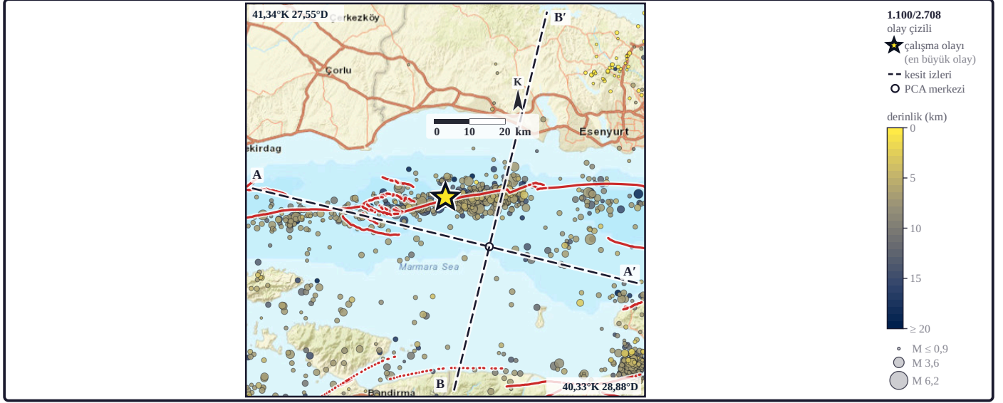
Şekil 4. Derinlik renkli harita 2.708 olaylık katalogdan 1.100 olayı gösterir. Daire rengi odak derinliğini, çapı büyüklüğü verir. Sarı yıldız çalışma olayıdır; kesikli A–A' ve B–B' doğruları kesitlerin harita izleridir.
