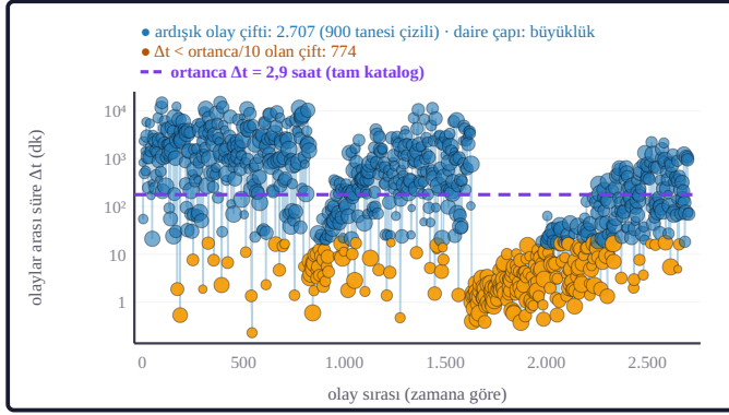
Şekil 10a. Düşey eksen bir önceki olaydan geçen süredir (dakika, logaritmik). Mor çizgi ortalama süredir; turuncu daireler ortalama sürenin onda birinden kısa aralıklardır. Daire çapı büyüklükle artar (seri: tekilleştirilmiş tam katalog).
