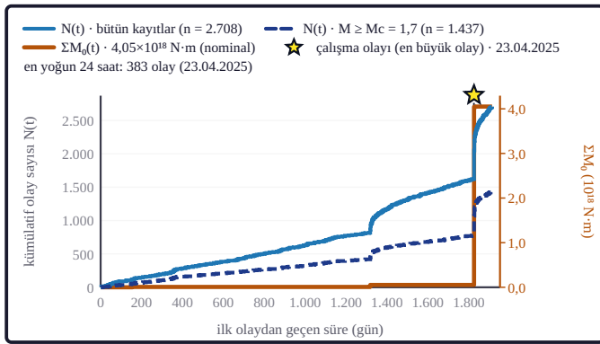
Şekil 9c. Mavi eğri kümülatif olay sayısı N(t) , turuncu eğri kümülatif sismik moment \Sigma M_0(t) değeridir. Sarı yıldız çalışma olayıdır; penceredeki en büyük olay da odur ( M_0 = 10^{[1,5 \cdot M + 9,1]} N\text{-m} ; 9,1 sabiti Kanamori, 1977).
