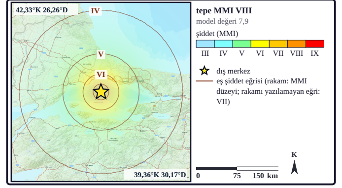
Şekil 7b. Harita modellenmiş makrosismik şiddet (MMI) alanını gösterir; yıldız dış merkezdir (şiddet-azalım bağıntısı: Allen vd., 2012).
