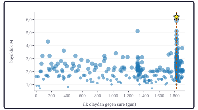
Şekil 2b. Pencere kataloğu 2.708 olaydır (320 olay çizilidir); en büyük olay çalışma olayıdır (Mw 6,2); Mc = 1,7 üstünde 1.437 olay vardır. Büyüklük-zaman dağılımı: yatay eksen ilk olaydan geçen süre (gün), dikey eksen büyüklüktür. Her mavi daire bir olaydır ve daire çapı büyüklükle ölçeklidir; turuncu kesikli dikey çizgi ve yıldız çalışma olayını işaretler (seyreltme eşit adımlıdır; en büyük 10 olay her durumda çizilmiştir).
