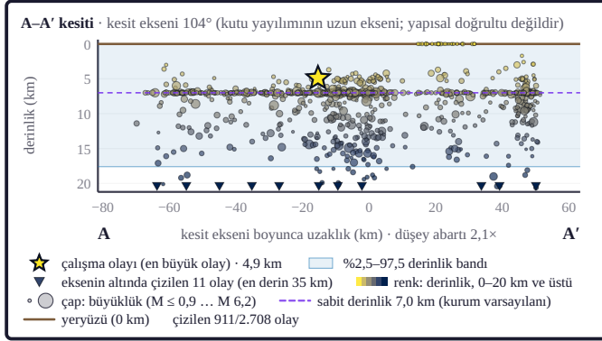
Şekil 3a. Olayların %95'i 0,0–17,6 km derinlik bandındadır; ortalama derinlik 7,0 km'dir (sabit atamalar dışlanınca 8,2 km). A–A' kesiti olayları kesit eksenini (kutu yayılımının uzun eksenini) boyunca uzanan düşey düzleme izdüşürür. Sarı yıldız çalışma olayıdır; daire rengi derinliği, çapı büyüklüğü verir. Alt kenardaki üçgenler derinlik ekseninin altında kalan olaylardır. Kesikli yatay çizgi kurumların varsayılan olarak atadığı sabit derinliktir. A–A' ve B–B' kesitleri aynı yatay açıklık ve aynı derinlik ekseniniyle çizilmiştir (izdüşüm: çalışma kutusundaki olayların çizim örnekleme; derinlikler katalog hiposantrlarıdır).
