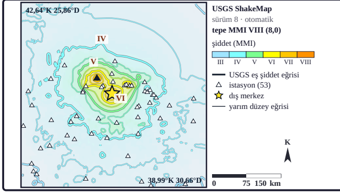
Şekil 7a. Harita USGS ShakeMap model kestiriminin (sürüm 8; otomatik ürün; 20.06.2025) eş şiddet (MMI) eğrilerini gösterir; ince eğriler yarım düzeylerdir; bu sürümde 81 sismik istasyon kaydı ve 516 şiddet gözleminin işaretlenmeyen 73'ü yer hareketi bağıntılarıyla birlikte kullanılmıştır; USGS belirsizlik derecesi A; üçgenler ShakeMap listesindeki 81 sismik istasyondan kadraj içinde kalan 53'ünü gösterir (dolu üçgen: en yüksek PGA); yıldız çalışma olayının dış merkezidir; ShakeMap'in girdi kökeni yıldızdan 2,4 km uzaktadır; renkli zemin orta çözünürlüklü USGS ShakeMap şiddet ızgarasının her 3. hücrelidir; zeminin en büyük değeri 7,7'dir (ürünün beyan ettiği tepe 8,0) (kurum ürünü: USGS ShakeMap; yöntem: Wald ve Worden, 2020; Worden vd., 2018).
