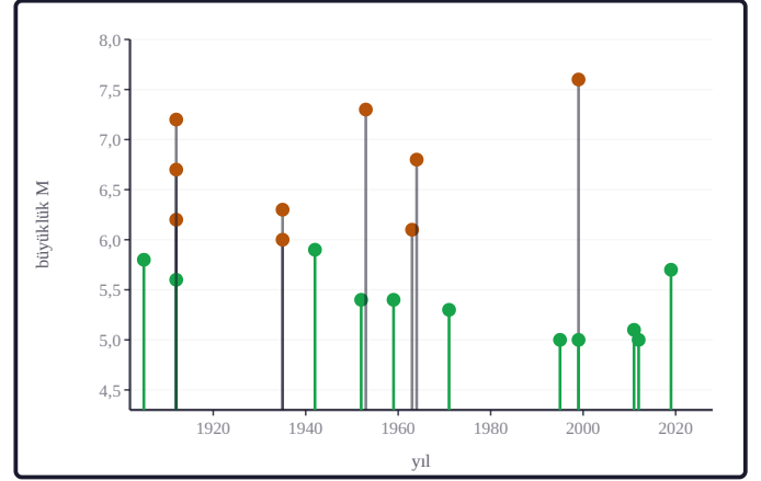
Şekil 13b. Tarihsel eşik üstü depremlerin büyüklükleri yıllara göre çizilmiştir; yeşil yakın kuşak, turuncu bölge kuşağıdır; sap rengi aynı ayrımı verir (yeşil sap yakın kuşak, gri sap bölge kuşağı) (birleşik katalog, 1900 sonrası; büyüklükler, varsa ISC-GEM Mw: International Seismological Centre, 2026; Di Giacomo vd., 2015, 2018).
