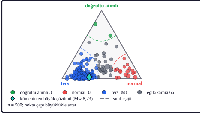
Şekil 8c. 500 çözümün %80'i ters sınıfındadır (%95 Wilson aralığı %73–85; 155 bağımsız küme). Alt uç %70 baskınlık eşliğinin üzerinde kaldığından bu sınıf baskın sayılmıştır. Bağımsız kümeler Gardner–Knopoff pencereleriyle ayrılmıştır. Frohlich üçgeninde her nokta bir odak mekanizması çözümünün P, T ve B eksenlerinin dalım açılarından gnomonik izdüşümle kurulan konumudur (köşeler: ters, normal, doğrultu atımlı). Renkli kesikli eğriler sınıf eşikleridir (B dalımı 60^\circ , P dalımı 60^\circ , T dalımı 50^\circ ); nokta rengi sınıfı, gri renk hiçbir eşığı aşmayan eğik/karma çözümleri, nokta çapı büyüklüğü, turkuaz elmas kümedeki en büyük çözümü gösterir; sınıf sayımları lejantıdır (Frohlich, 1992 gnomonik üçgeni; Frohlich ve Apperson, 1992 eşikleri; çözümler: Global CMT, Ekström vd., 2012).
