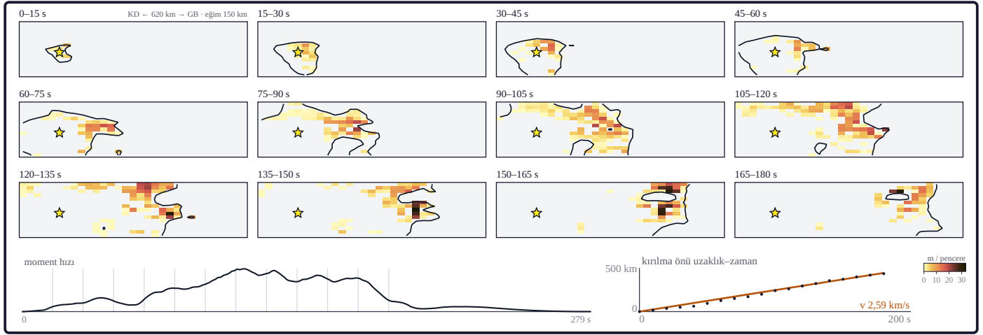
Şekil 20. Kırılma anlık görüntüleri: USGS NEIC us6000qw60 (ürün tarihi 19.11.2025) kayma modelinin açılmış fay düzleminde (yatay doğrultu boyunca, düşey eğim aşağı) 12 ardışık 15 s'lik pencerede açığa çıkan kayma; renk pencere içindeki kaymadır (ortak ölçek 0–33,1 m; model çıktısı); 180 s'den sonra toplam kaymanın %8,2'si (momentin %6,3'ü) açığa çıkar; panolardaki kayma ile bu kalan pay toplam kaymayı verir (fark %0,0); kaynak zaman işlevi yama başına yükselme ve düşme süreli asimetrik kosinüstür (modelin kendi parametreleri); siyah eğri pencere sonu kırılma önu; küçük pano kırılma önu uzaklık-zaman: v = 2,59 \text{ km/s} (model: kurum ürünü: USGS NEIC sonlu fay modeli us6000qw60 [U.S. Geological Survey, 2017]; yöntem: bu çalışma [açılmış düzlem, pencere integrali]; renk: lajolla [Cramer, 2018]).
