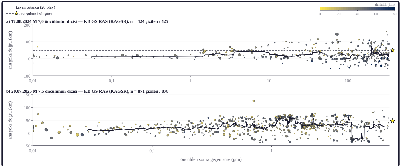
Şekil 5b. Her pano bir büyük öncül dizisidir: yatay eksen öncülünden sonra geçen süre (gün, logaritmik), düşey eksen olayın öncülünden ana şoka uzanan doğrultuya izdüşümüdür (km; artı yön ana şoka doğru); daireler seçilen katalogun raporlarıdır (renk derinlik, ortak 0–80 km ölçeği; 15 olay daha derin, en koyu renkte; boyut büyüklük); koyu çizgi 20 olaylık kayan ortanca, kesikli yatay çizgi ve sarı yıldız ana şokun izdüşümüdür; katalog her dizide bu çalışmanın kuralıyla seçildi: iki katalogun tamlık büyüklüğünün (azami eğrilik + 0,2) büyüğü ortak eşik alındı, bu eşğin üstünde olay sayısı büyük olan katalog kullanıldı — a) KB GS RAS (KAGSR) (Mc 4,6; USGS NEIC (ComCat) 39, KB GS RAS (KAGSR) 50 olay); b) KB GS RAS (KAGSR) (Mc 4,4; USGS NEIC (ComCat) 193, KB GS RAS (KAGSR) 276 olay); pano yalnız öncülünden 15 s sonrası ile pencere sonu arasındaki kayıtları çizer (öncülün kendi raporları dışarıda); başlıktaki n çizilen sayıdır, pencere sayımı ondan büyüktür (424 / 425; 871 / 878) (katalog: KB GS RAS [KAGSR]; katalog seçimi, izdüşüm ve kayan ortanca: bu çalışma).
