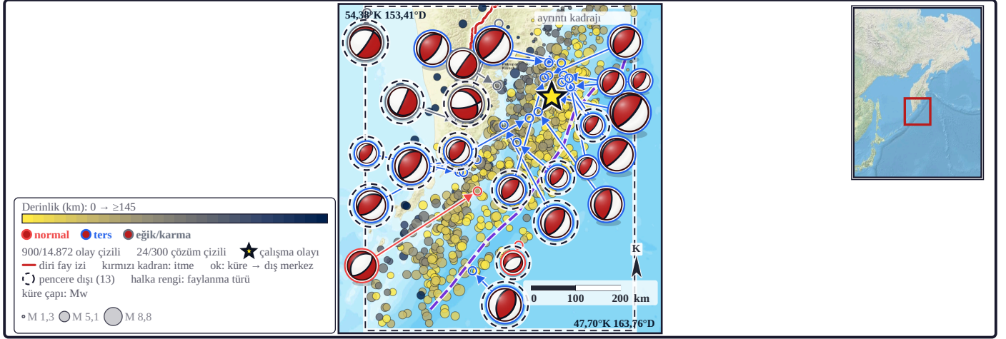
Şekil 36c. Bölgesel odak mekanizması çerçevesi: harita, çevrede yayımlanmış çözümlerin Mw sırasıyla en büyüklerini gösterir; ötelenen küreler okla konumlarına bağlıdır. Küreler alt yarıküre izdüşümünde odak mekanizmalarıdır; kırmızı kadranslar P dalgasının ilk hareketinin itme olduğu bölgelerdir. Küreler künyesizdir. Küçük daireler pencere olayları, kesikli dikdörtgen ayrıntı haritasının kadranıdır (mekanizma kümesi: bölgesel küme [ n = 300 ]; gerilme inversiyonu olay merkezli mekanizma popülasyonundandır [ n = 467 ]; faylar: GEM Global Active Faults [Styron ve Pagani, 2020] — CC BY-SA 4.0).
