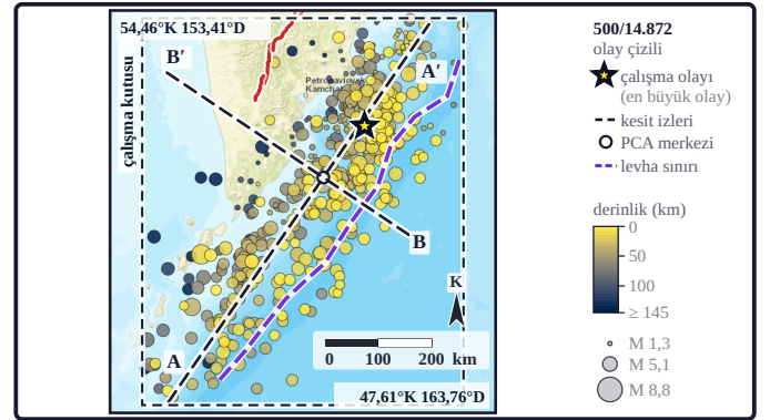
Şekil 3d. Derinlik renkli harita 14.872 olaylık katalogdan 500 olayı gösterir. Daire rengi odak derinliğini, çapı büyüklüğü verir. Sarı yıldız çalışma olayıdır; kesikli A-A' ve B-B' doğruları kesitlerin harita izleridir (kesikli dikdörtgen çalışma kutusudur; kutunun dışı sorgulanmamıştır, oradaki fay izleri bağlam içindir).
