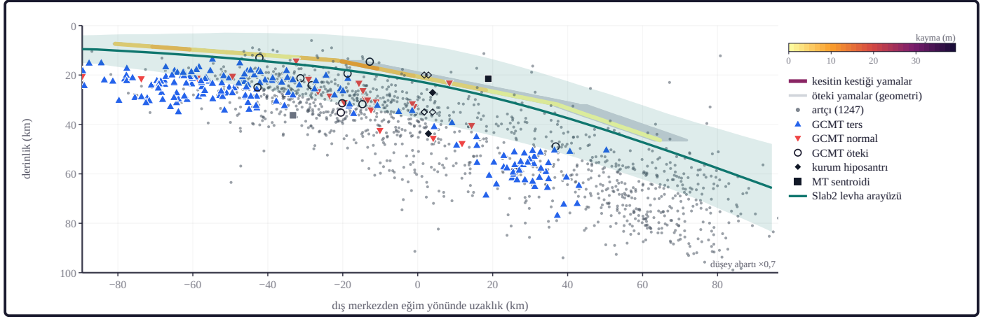
Şekil 15. Kesit dış merkezden geçen ve USGS NEIC us6000qw60 (ürün tarihi 19.11.2025) modelinin temsili doğrultusuna (217°) dik düşey düzlemdir; yatay eksen eğim yönünde (307°) uzaklıktır, eksi değerler eğim yukarıdır; şerit modelin doğrultu boyunca kapladığı 625 km'dir; renkli parçalar USGS FFM modelinin kesitin kestiği 15 yaması (kayma 0–39,3 m; model), açık gri öteki yamalar (geometri); noktalar artçıları (1.247; sabit derinlikli 1.677 çizilmedi); imler GCMT artçıları, sentroid derinliği; sabit 19 çizilmedi; elmaslar kurum hiposantr derinlikleri (içi boş: sabit / bağımlı) (model: kurum ürünü: USGS NEIC sonlu fay modeli us6000qw60 [U.S. Geological Survey, 2017]; artçıları: USGS NEIC [ComCat] [U.S. Geological Survey, 2017]; GCMT: Dziewonski vd., 1981; levha yüzeyi: Slab2 [Hayes, 2018], Seismo Lab hesabı).
