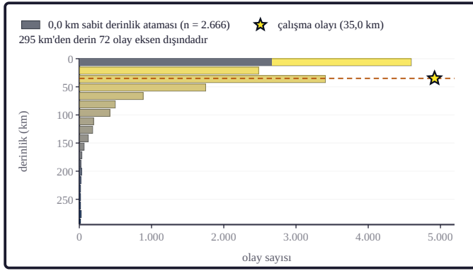
Şekil 4a. Tam katalogda derinlik değeri taşıyan 14.872 olayın %29'u \leq 10 km derinliktedir. Sabit derinlik atamaları (0,0 km) ölçülmüş derinlik taşımaz. Hiposantr derinlik histogramı (tam katalog): çubuk rengi derinliği gösterir (sıfır sarı, derin lacivert); koyu kesim sabit derinlik atamalarıdır; yıldız ve kesikli çizgi çalışma olayının derinliğidir.
