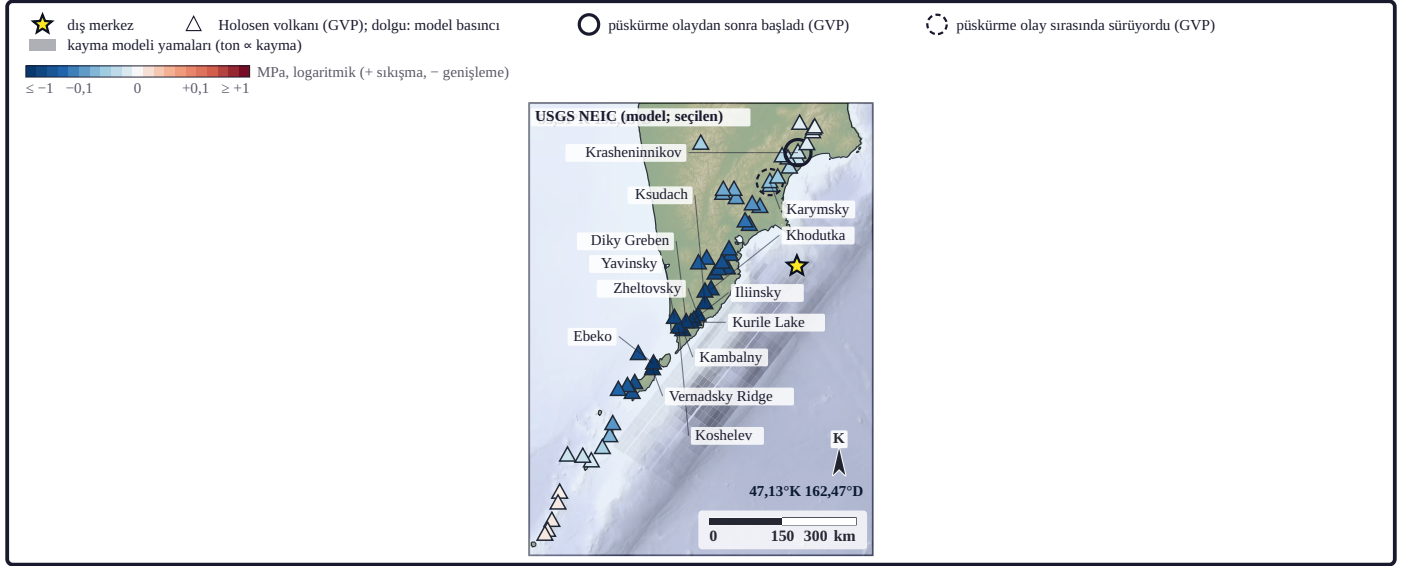
Şekil 22. 58 Holosen volkanı (GVP; min(dış merkez, kırılma izi) \leq 300 km; aday kümesi USGS NEIC kırılma iziyle kurulmuştur). Üçgen dolgu volkanın altında 2–10 km derinlikteki eşsismik kaya basıncı değişiminin ortalamasıdır ( P = -(\sigma_1 + \sigma_2 + \sigma_3)/3 ; + sıkışma, - genişleme; renk işaretli logaritmik ölçekte ( \pm 0,01 MPa'ya dek doğrusala yakın), \pm 1 MPa'da doygun); basınç MODEL çıkışıdır: USGS NEIC, kamu malı (USGS) kayma modelleriyle ( \mu = 30 GPa, \nu = 0,25 ). Basınç homojen elastik yarı uzay varsayımıyla Okada (1992) çözümünden hesaplanmıştır; topoğrafya ve katmanlı ortam yoktur. Gri tonlu dörtgenler panel modelinin yamalarının yüzey izdüşümüdür (ton kaymayla orantılı). Halka GVP'ye göre olay penceresindeki püskürme durumudur (Krashennikov: olaydan sonra başladı, 3 gün sonra; Karymsky: olay sırasında sürüyordu; gün farkı volkanın nominal yerel takvim günüyle (GVP tarihleri saat taşımaz; \pm 1 gün). Öbür imler Şekil 6'deki gibidir. Zemin ETOPO 2022 gölgeli kabartmasıdır (oleron: mavi tonlar deniz, yeşil-kahve tonlar kara); ince koyu çizgi aynı ızgaranın 0 m eğrisidir (gelgit kıyı çizgisi değildir) (volkanlar ve püskürmeler: Global Volcanism Program, Smithsonian Institution; basınç: bu çalışma [model; Okada, 1992]; model: kurum ürünü: USGS NEIC sonlu fay modeli us6000qw60 [U.S. Geological Survey, 2017]; altlık ve kıyı çizgisi: ETOPO 2022 [30" ızgara, NOAA NCEI, doi:10.25921/fd45-gt74]; renk: oleron [Cramer, 2018a, 2018b]).
