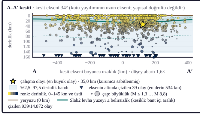
Şekil 3a. Olayların %95'i 0,0-142,6 km derinlik bandındadır; ortanca derinlik 31,6 km'dir (sabit atamalar dışlanınca 40,7 km). A-A' kesiti olayları kesit eksenini (kutu yayılımının uzun eksenine) boyunca uzanan düşey düzleme izdüşürür. Sarı yıldız çalışma olayıdır; daire rengi derinliği, çapı büyüklüğü verir. Alt kenardaki üçgenler derinlik ekseninin altında kalan olaylardır. Kesikli yatay çizgi kurumların varsayılan olarak atadığı sabit derinliktir. A-A' ve B-B' kesitleri aynı yatay açıklık ve aynı derinlik eksenine çizilmiştir (izdüşüm: çalışma kutusundaki olayların çizim örneği; derinlikler katalog hiposantrlarıdır; levha yüzeyi: Slab2 [Hayes, 2018], Seismo Lab hesabı).
