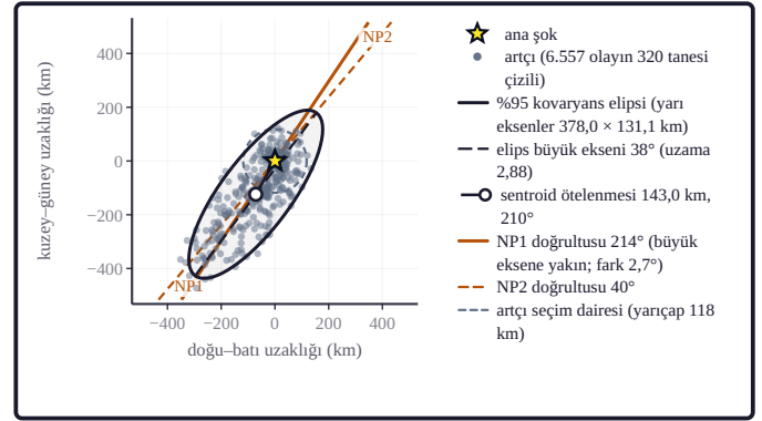
Şekil 9b. Ana şoka göre yerel yatay düzlemde (doğu ve kuzey artı, km; iki eksen aynı ölçekte) artçı bulutu gri noktalarla, %95 kovaryans elipsi koyu çizgiyle gösterilmiştir; elips bulutun ağırlık merkezine oturur ve yıldız ana şoktur. Elips, artçı konumlarının kovaryansından Gauss dağılımı varsayımıyla kurulan bir yayılım ölçüsüdür; artçıların %95'ini içeren bir sınır değildir. Kesikli koyu doğru elipsin büyük eksenidir; ana şoktan çıkan ince çizgi ve içi boş daire artçı sentroidinin ötelenmesidir; gri kesikli çember artçıların seçildiği dairedir. Bulut bu daireye dayandığından uzama oranı seçim yarıçapıyla sınırlıdır (gerçek değer için alt sınır) ve sentroid dış merkeze doğru yanlıdır. Turuncu doğrular ana şokun düğüm düzlemlerinin doğrultularıdır; büyük eksene doğrultuca yakın olan düz, öteki kesikli çizilmiştir. Uzama oranı 1'e yaklaştıkça bulut izotroplaşır ve yön kestirimi zayıflar; elips ölçüleri lejantıdır (telesismik ikinci moment ölçüsünün artçı konumlarına uyarlanmış vekili: McGuire vd., 2002).
