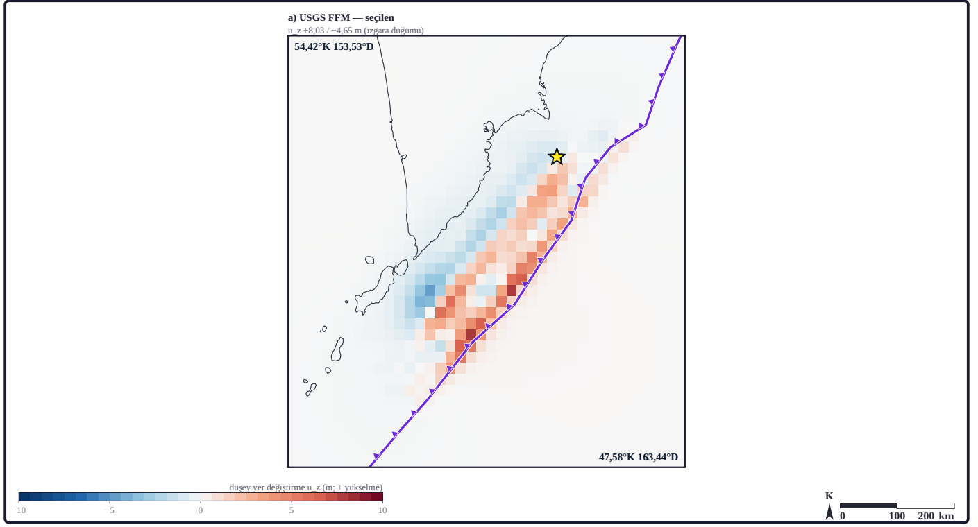
Şekil 28. Panel kayma modelinden hesaplanan kosmik düşey yer değiştirmedir ( u_z , + yükselme): USGS NEIC us6000qw60 (ürün tarihi 19.11.2025) (seçilen); model ileri hesabı yamaların Okada (1985) yüzey çözümüyle toplamıdır: homojen elastik yarı uzay (katmanlı ortam değil); bütün model değerleri model çıktısıdır; renk ölçeği seçilen modelin tepesine göre \pm 10 m'de doyar; panel kendi uçlarını (kaba ızgara düğümünde) yazar; PB2002 hendek izi, ETOPO 2022 batimetrisindeki hendek ekseninden ortanca \approx 10 km kara (üst levha) yönündedir (iz boyunca 10 km arayla 84 dik kesitte en derin nokta; %10–90 aralığı 5 ile 30 km); iz yayımlandığı gibi çizilmiştir (model: kurum ürünü: USGS NEIC sonlu fay modeli us6000qw60 [U.S. Geological Survey, 2017]; yöntem: Okada, 1985; kıyı çizgisi [0 m eğrisi]: ETOPO 2022 [30" ızgara, NOAA NCEI, doi:10.25921/fd45-gt74]).
