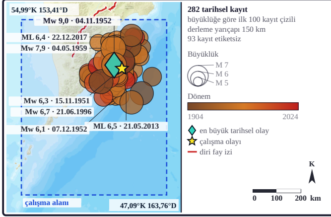
Şekil 36a. Çalışma olayından önceki eşik üstü kayıtlarda daire çapı büyüklüğü, dolgu rengi oluş dönemini gösterir. Turkuaz elmas derlemenin en büyük kaydı, sarı yıldız çalışma olayıdır. Kayıt eşiği yakın kuşakta M \geq 5 , bölge kuşağında M \geq 6 olarak alınmıştır. Mavi kesikli dikdörtgen çalışma alanıdır (birleşik katalog, 1900 sonrası; derleme yarıçapı 150 km, yakın kuşak 60 km).
