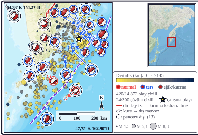
Şekil 1. Harita 14.872 olaylık katalogdan 420 olayı gösterir; odak mekanizmaları 300 çözümlük bölgesel mekanizma kümesindedir. Gerilme inversiyonu olay merkezli mekanizma popülasyonundandır ( n = 467 ). Daire rengi odak derinliğini, çapı büyüklüğü verir; kadranlı küreler odak mekanizması çözümleridir; kırmızı kadranlar P dalgasının ilk hareketinin itme olduğu bölgelerdir. Sarı yıldız çalışma olayı, kırmızı çizgiler diri fay izleridir. Küreler küyesizdir. Ok küreyi çözümün dış merkezine bağlar. Kesikli halkalı kürelerin tarihi çalışma penceresinin dışındadır (faylar: GEM Global Active Faults [Styron ve Pagani, 2020] — CC BY-SA 4.0; mekanizmalar: bölgesel mekanizma kümesi; katalog: ISC · GSRAS · USGS · KAGSR · EMSC · GFZ; altlık: Esri, HERE, Garmin, OSM katkıları).
