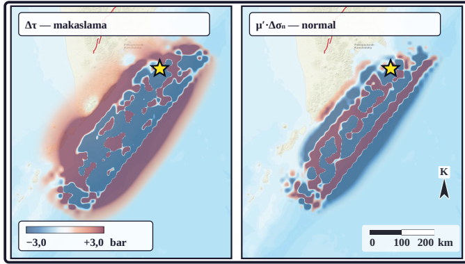
Şekil 9a. ΔCFS'in iki bileşeni ayrı panellerde gösterilmiştir: solda makaslama gerilmesi değişimi \Delta\tau , sağda fay düzlemine dik normal gerilme katkısı \mu' \cdot \Delta\sigma_n ( \Delta CFS = \Delta\tau + \mu' \cdot \Delta\sigma_n ; \Delta\sigma_n çekme artı, artı değer fayın kenetlenmesinin azalmasıdır). Kadraj kaynak çevresine yakınlaştırılmıştır; renk ölçeği ve kaynak geometrisi ΔCFS haritasıyla aynıdır; yıldız dış merkezdir (bileşen ayrışımı: Okada, 1992 analitik çözümü; kurum ürünü: USGS NEIC sonlu fay modeli us6000qw60 [U.S. Geological Survey, 2017]).
