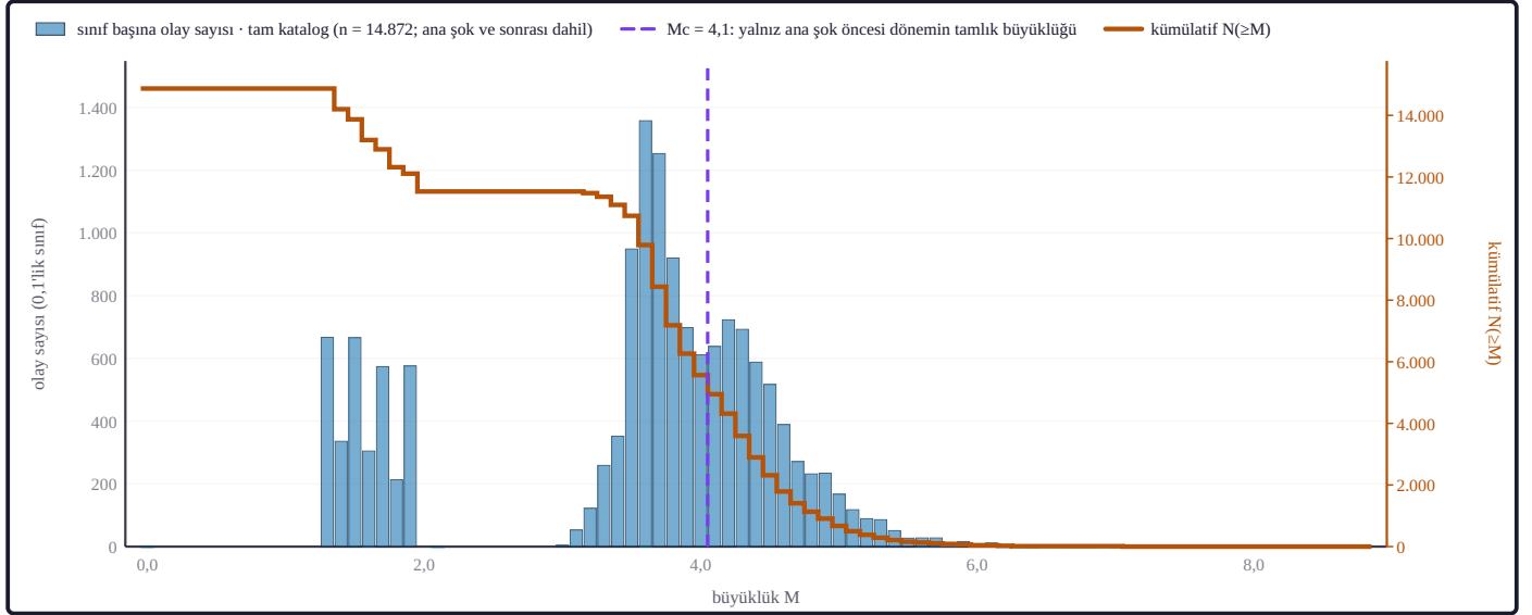
Şekil 35. Tamlik büyüklüğü (ana şok öncesi dönem) M_c = 4,1 olarak benimsenmiştir (b-kararlılığı ölçütü); bu eşikte uyum iyiliği %97,6 düzeyindedir; pencerenin en büyük olayı çalışma olayıdır (Mw 8,8). Mavi çubuklar 0,1 genişliğindeki büyüklük sınıflarına düşen olay sayısıdır (sol eksen); ana şok ve sonrası dahil tam katalog; turuncu eğri kümülatif N(\geq M) sayımıdır (sağ eksen). Mor kesikli çizgi yalnız ana şok öncesi dönemin tamlik büyüklüğüdür (tam katalog, n = 14.872 ).
