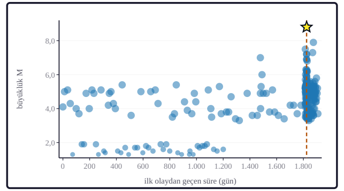
Şekil 2b. Pencere kataloğu 14.872 olaydır (320 olay çizilidir); en büyük olay çalışma olayıdır (Mw 8,8); ana şok öncesi dönemde M_c = 4,1 üstünde 1.476 olay vardır. Büyüklük-zaman dağılımı: yatay eksen ilk olaydan geçen süre (gün), dikey eksen büyüklüktür. Her mavi daire bir olaydır ve daire çapı büyüklükle ölçektir; turuncu kesikli dikey çizgi ve yıldız çalışma olayını işaretler (seyreltme eşit adımlıdır); en büyük 10 olay her durumda çizilmiştir).
