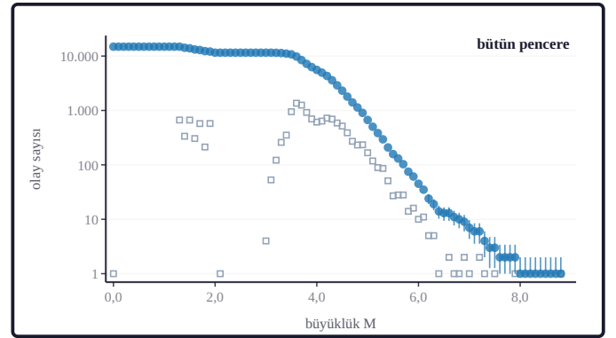
Şekil 2d. Ana şok öncesi dönemde M_c = 4,1 (b-kararlılığı) üstündeki 1.476 olaydan b = 1,12 \pm 0,06 kestirilmiştir. Gutenberg-Richter büyüklük-frekans dağılımı: dolu daireler kümülatif sayımı N(\geq M) , açık gri kareler her büyüklük aralığındaki artımsal sayımı verir; ince dikey çubuklar N \leq 30 olan aralıklarda \sqrt{N} Poisson belirsizliğidir. Çizilen dağılım bütün pencereye aittir; ana şok öncesi dönemin uyum doğrusu bu nedenle çizilmemiştir (dağılım: Gutenberg ve Richter, 1944).
