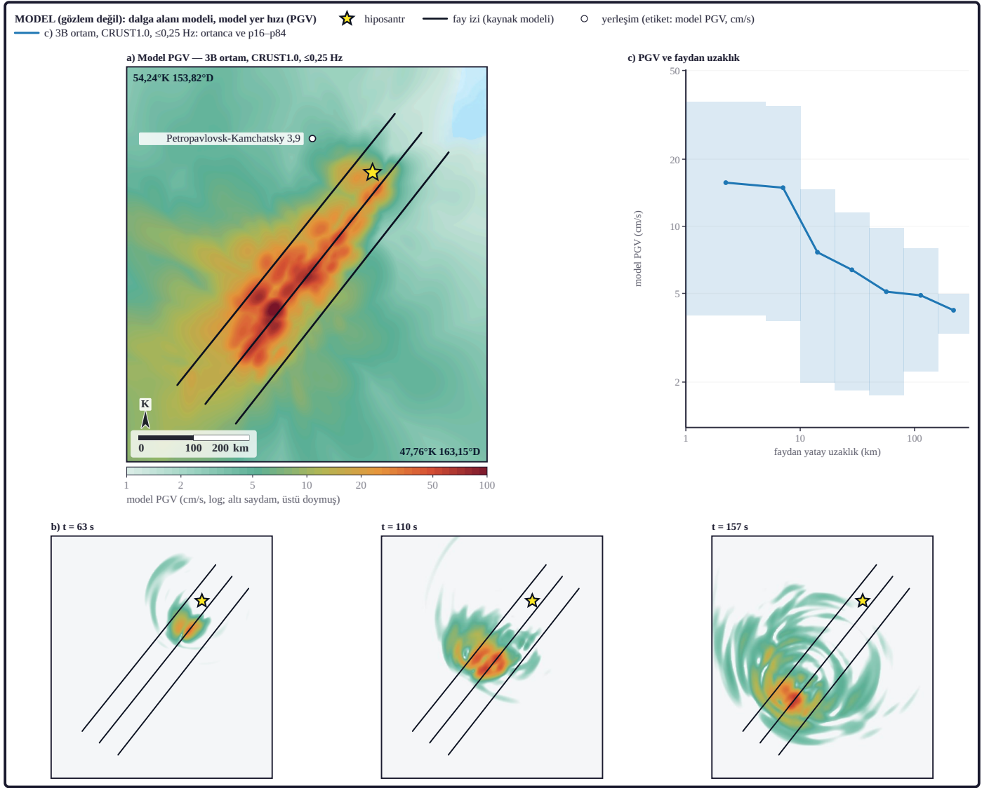
Şekil 34. Dalga alanı modeli, MODEL — gözlem değil: a) 3B ortam, CRUST1.0 çözümünde \leq 0,25 Hz model yer hızı (PGV); renk ölçeği logaritmik, 1–100 cm/s, alt sınırın altı saydam, üst sınırın üstü doymuş; b) aynı çözümün t = 63, 110 ve 157 s anlarındaki hız büyüklüğü |v| , aynı renk ölçeğiyle; c) PGV ile faydan yatay uzaklık, model başına kuşak ortalancası (çizgi) ve p16–p84 aralığı (bant), iki eksen logaritmik; kinematik kaynak: us6000qw60; kırılma süresi 271 s; havza büyütmesi ve yerel zemin etkisi hesapta yoktur; 3B ortamda kayma dalgası hızı tabanı 2,571 km/s (model: Seismo Lab dalga alanı hesabı — 3B ortam: Seismo Lab kendi sonlu farklar çözücüsü yz-sf3b/2 [Virieux, 1986; Graves, 1996, Q sönümü: Day, 1998], CRUST1.0, Laske vd., 2013; kaynak: us6000qw60).
