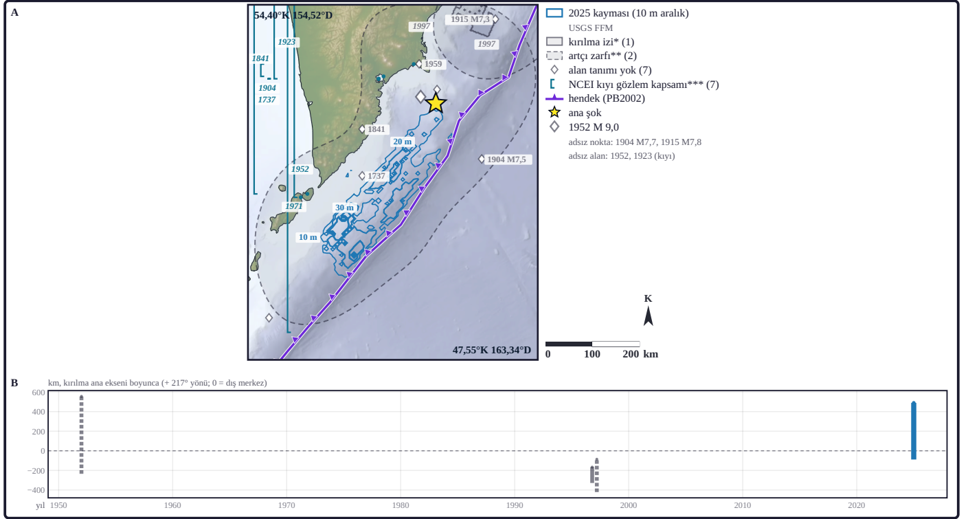
Şekil 11. Tarihsel büyük depremler: kırılma alanları ve uzay-zaman dağılımı: (A) mavi eğriler USGS NEIC us6000qw60 (ürün tarihi 19.11.2025) kayması (10 m aralıklı; model); gri düz çizgili alanlar 1997 sonlu fay modeli izleri (kayma \geq 0,1 \times tepe); gri kesikli alanlar 1952, 1997 katalog artçı zarfı (kırılma alanı değil); açık eşkenar dörtgenler 1737, 1841, 1904, 1915, 1959 dış merkezleri (1737, 1841 temsili, NCEI) (sayısal alan tanımı yok, çizilmedi); *** köşeli çizgiler NCEI kıyı gözlem kapsamı (1737: 5, 1841: 3, 1904: 1, 1923: 6, 1923: 2, 1952: 42, 1971: 2 nokta; kırılma alanı değil); ara / derin odaklı 3 olay çizilmedi (1957 148 km, 2008 633 km, 2013 607 km); (B) gri çubuklar tarihsel kırılma alanlarının 217° eksenine izdüşümü, mavi çubuk bu deprem (kayma modeli: kurum ürünü: USGS NEIC sonlu fay modeli us6000qw60 [U.S. Geological Survey, 2017]; kırılma izleri: USGS NEIC sonlu fay modelleri usp0008btk [U.S. Geological Survey, 2017]; artçı zarfları: bu çalışma [katalogdan]; dış merkezler: International Seismological Centre, 2026; National Geophysical Data Center / World Data Service, t.y.; kıyı gözlemleri: National Geophysical Data Center / World Data Service, t.y.; uzay-zaman: kırılma ana eksenine 217° [seçilen kayma modelinin kırılma eksenine, bu çalışmanın ölçüsü]; alanların eksene en yakın uzaklığı en çok 2 km; alan tanımı olmayan 14 kayıt izdüşüme girmez; levha sınırı: Bird, 2003 [iz, ETOPO 2022 hendek ekseninden ortalca \approx 11 km kara yönünde]; altlık ve kıyı çizgisi: ETOPO 2022 [30" ızgara, NOAA NCEI, doi:10.25921/fd45-gt74]; renk: oleron [Cramer, 2018a, 2018b]).
