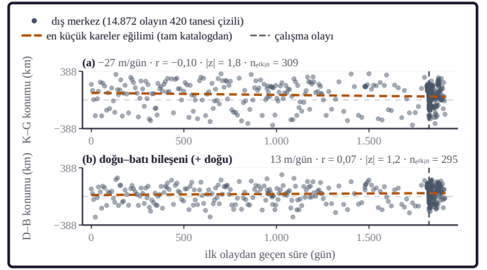
Şekil 4b. Dış merkez koordinatlarının zaman serisi iki şeritte verilmiştir: (a) kuzey-güney, (b) doğu-batı bileşeni. Düşey eksen pencere kutusunun merkezine uzaklıktır (km; kuzey ve doğu artı) ve iki şerit aynı ölçektedir; yatay eksen pencerenin ilk olayından geçen süredir (gün). Turuncu kesikli doğrular iki bileşenin en küçük kareler eğilimidir; eğim, Pearson korelasyon katsayısı ve etkin örneklem büyüklüğüyle hesaplanan Fisher z değeri şerit başlığındadır. Kesikli düşey çizgi çalışma olayının anını işaretler.
