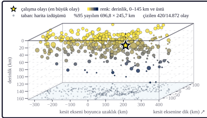
Şekil 3c. Yatay eksen kesit eksenini (kutu yayılımının uzun eksenine) boyunca, sağ üste kaçan eksen ona dik uzaklığı, düşey eksen derinliği verir. Derinlik eksenini kesitlerle ayırır. Yıldızdan üst yüzeye çıkan kesikli çizgi olayın yüzeydeki izdüşümünü gösterir (kabinet izdüşümü; üç eksen ayrı ölçeklidir; blok kenarları %95 yayılımın 1,06 katıdır).
