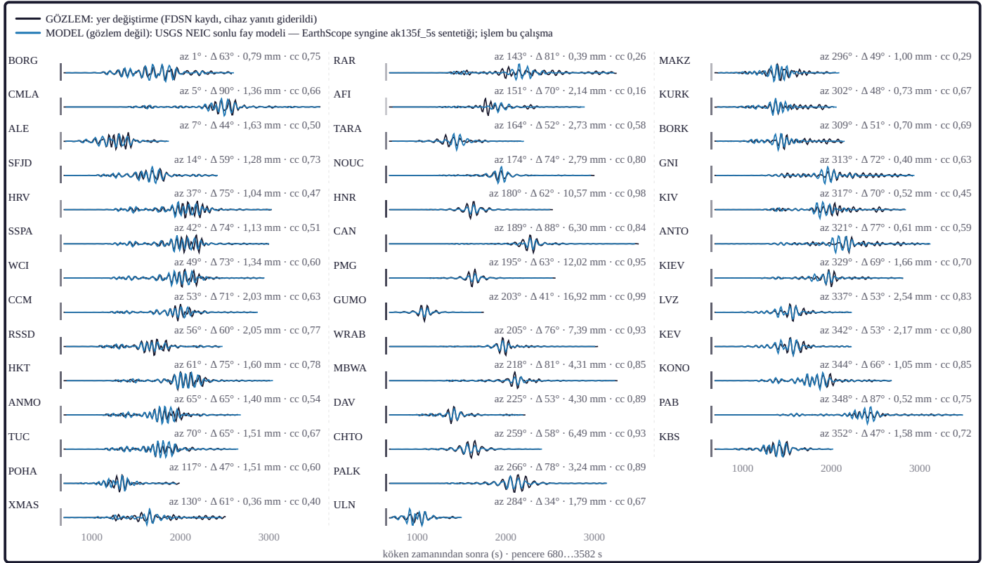
Şekil 18. 40 telesismik istasyonda (30–90°; açılar G , GE , II , IU ) Love dalgası enine ( T ; yataylar istasyondan kaynağa azimutla döndürüldü) bileşen yer değiştirmesi: siyah GÖZLEM (EarthScope veri hizmetleri), mavi MODEL — USGS NEIC sonlu fay modeli için EarthScope syngine ak135f_5s sentetiği (sentetik syngine hizmetinde hesaplandı; işlem bu çalışma). Love sentetiği, kurum ürünü kayma modelinin yamalarının syngine sonlu fay yoluyla toplanmasıdır. Love kayıtları cihaz yanıtı giderilip 50–100 s bandında (Butterworth, sıfır fazlı) süzüldü. Love izlerinin zaman eksenini köken zamanına göre (680...3582 s); sentetik, ilintiyi en büyük yapan zaman ötelemesiyle ( \pm 40 s içinde) kaydırılarak çizildi. Love izlerinde solda istasyon kodu, sağ üstte azimut, uzaklık ( ^\circ ), gözlemin tepe genliği (mm; bu çalışmanın süzgeciyle) ve ilinti katsayısı (cc); izin solundaki ince çubuk cc arttıkça açık griden koyu griye döner. Uyum (40 iz): kaydırılmış sentetik ile ilinti ortancası 0,70 (çeyrekler 0,58–0,83), kaymasız -0,11 ; varyans azalımı ortancası 0,35; genlik oranı (gözlem / sentetik, RMS) ortancası 1,07; 6 izde kayma arama sınırına dayandı. Öteki kaynakların ilinti ortancası (çizilmedi): GCMT C202507292324B nokta kaynak 0,49; USGS W-fazı ( M_{ww} ) nokta kaynak 0,54 (veri: EarthScope Consortium veri hizmetleri [eski IRIS DMC] [FDSN dataset]; cihaz yanıtı: EarthScope FDSN station hizmeti; açılar G [doi:10.18715/GEOSCOPE.G], GE [doi:10.14470/TR560404], II [doi:10.7914/SN/II], IU [doi:10.7914/SN/IU]; sentetik: EarthScope syngine [doi:10.17611/DP/SYNGINE.1]; Krischer vd., 2017; Nissen-Meyer vd., 2014; van Driel vd. 2015], ak135f_5s [ak135: Kennett vd., 1995; yoğunluk ve Q : Montagner ve Kennett, 1996]; kurum ürünü: USGS NEIC sonlu fay modeli us6000qw60 [U.S. Geological Survey, 2017]; varış: IASP91 [Kennett ve Engdahl 1991]; işlem: bu çalışma).
