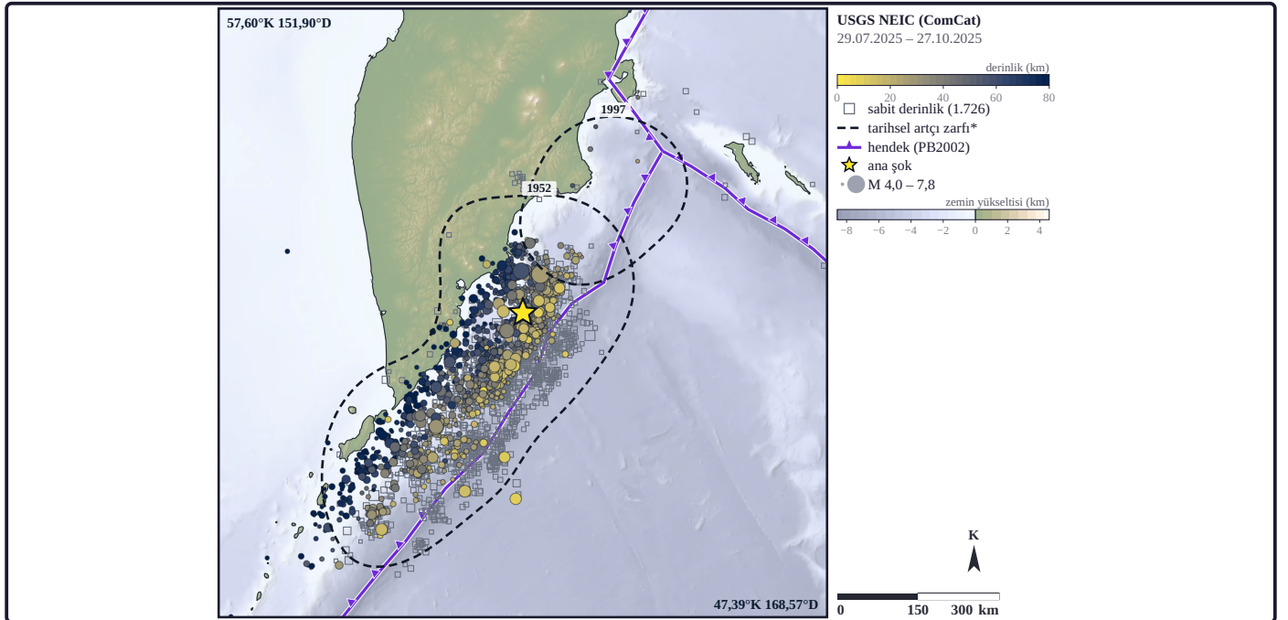
Şekil 4c. Noktalar USGS NEIC (ComCat) kataloğunun kendi raporlarıdır; ana şoktan sonraki 90 gün (29.07.2025 – 27.10.2025), dış merkezin artçı yarıçapı kutusu, n = 3.017 ; boyut büyüklüğüne göre; renk derinliktir (0–80 km; 103 olay daha derin, en koyu renkte); içi boş gri kareler kurumun sabit derinlik değerlerindeki raporlardır (10 / 35 km; 1.726 olay, %57) — bu derinlikler ölçülmüş değildir; kesikli çizgiler 1952, 1997 depremlerinin ilk 30 gündeki artçılarından katalogdan türetilmiş zarflardır; yayımlanmış kırılma poligonları değildir (katalog: USGS NEIC [ComCat] [U.S. Geological Survey, 2017]; artçı zarfları: bu çalışma [katalogdan]; levha sınırı: Bird, 2003 [iz, ETOPO 2022 hendek ekseninden ortalca \approx 10 km kara yönünde]; altlık ve kıyı çizgisi: ETOPO 2022 [30" ızgara, NOAA NCEI, doi:10.25921/fd45-gt74]; renk: oleron [Crameri, 2018a, 2018b]).
