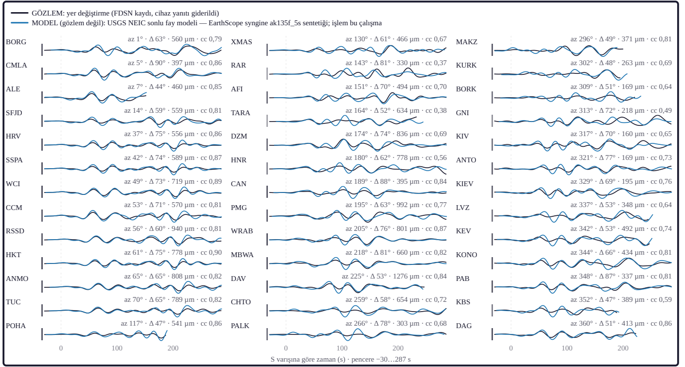
Şekil 17. 39 telesismik istasyonda (30–90°; ağırlar G, GE, II, IU) SH dalgası enine (T; yataylar istasyondan kaynağa azimutla döndürüldü) bileşen yer değiştirmesi: siyah GÖZLEM (EarthScope veri hizmetleri), mavi MODEL — USGS NEIC sonlu fay modeli için EarthScope syngine ak135f_5s sentetiği (sentetik syngine hizmetinde hesaplandı; işlem bu çalışma). SH sentetiği, kurum ürünü kayma modelinin yamalarının syngine sonlu fay yoluyla toplanmasıdır. SH kayıtları cihaz yanıtı giderilip 25–100 s bandında (Butterworth, sıfır fazlı) süzüldü; alt sınır, sentetiği kurulan sonlu fay modelinin alt fay boyutundan türetili ( \Delta 20 km; T \geq 4\Delta/\beta , \beta 3,75 km/s): sentetik her alt fayı tek nokta kaynakla temsil ettiğinden daha kısa periyotta yapay enerji taşır. SH penceresi, Love dalgası girmeden kesildi. SH izlerinin zaman eksenini IASP91 S varışına göre (-30...287 s); sentetik, ilintiyi en büyük yapan zaman ötelemesiyle ( \pm 15 s içinde) kaydırılarak çizildi. SH izlerinde solda istasyon kodu, sağ üstte azimut, uzaklık (°), gözlemin tepe genişliği ( \mu\text{m} ; bu çalışmanın süzgeciyle) ve ilinti katsayısı (cc); izin solundaki ince çubuk cc arttıkça açık griden koyu griye döner. Uyum (39 iz): kaydırılmış sentetik ile ilinti ortancası 0,81 (çeyrekler 0,68–0,84), kaymasız 0,62; varyans azalımı ortancası 0,08; genlik oranı (gözlem / sentetik, RMS) ortancası 0,69. Öteki kaynakların ilinti ortancası (çizilmedi): GCMT C202507292324B nokta kaynak \geq 0,31 (21 / 39 izde kayma \pm 15 s arama sınırına dayandı; değer alt sınırdır); USGS W-fazı (Mww) nokta kaynak 0,42 (veri: EarthScope Consortium veri hizmetleri [eski IRIS DMC] [FDSN dataset]; cihaz yanıtı: EarthScope FDSN station hizmeti; ağırlar G [doi:10.18715/GEOSCOPE.G], GE [doi:10.14470/TR560404], II [doi:10.7914/SN/II], IU [doi:10.7914/SN/IU]; sentetik: EarthScope syngine [doi:10.17611/DP/SYNGINE.1; Krischer vd., 2017; Nissen-Meyer vd., 2014; van Driel vd. 2015], ak135f_5s [ak135: Kennett vd., 1995; yoğunluk ve Q: Montagner ve Kennett, 1996]; kurum ürünü: USGS NEIC sonlu fay modeli us6000qw60 [U.S. Geological Survey, 2017]; varış: IASP91 [Kennett ve Engdahl 1991]; işlem: bu çalışma).
