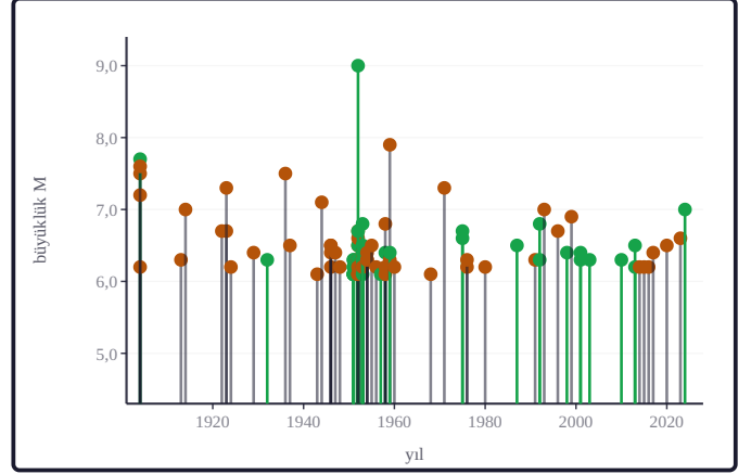
Şekil 36b. Tarihsel eşik üstü depremlerin büyüklükleri yıllara göre çizilmiştir; yeşil yakın kuşak, turuncu bölge kuşağıdır; sap rengi aynı ayrımı verir (yeşil sap yakın kuşak, gri sap bölge kuşağı) (birleşik katalog, 1900 sonrası; büyüklükler, varsa ISC-GEM Mw: International Seismological Centre, 2026; Di Giacomo vd., 2015, 2018).
