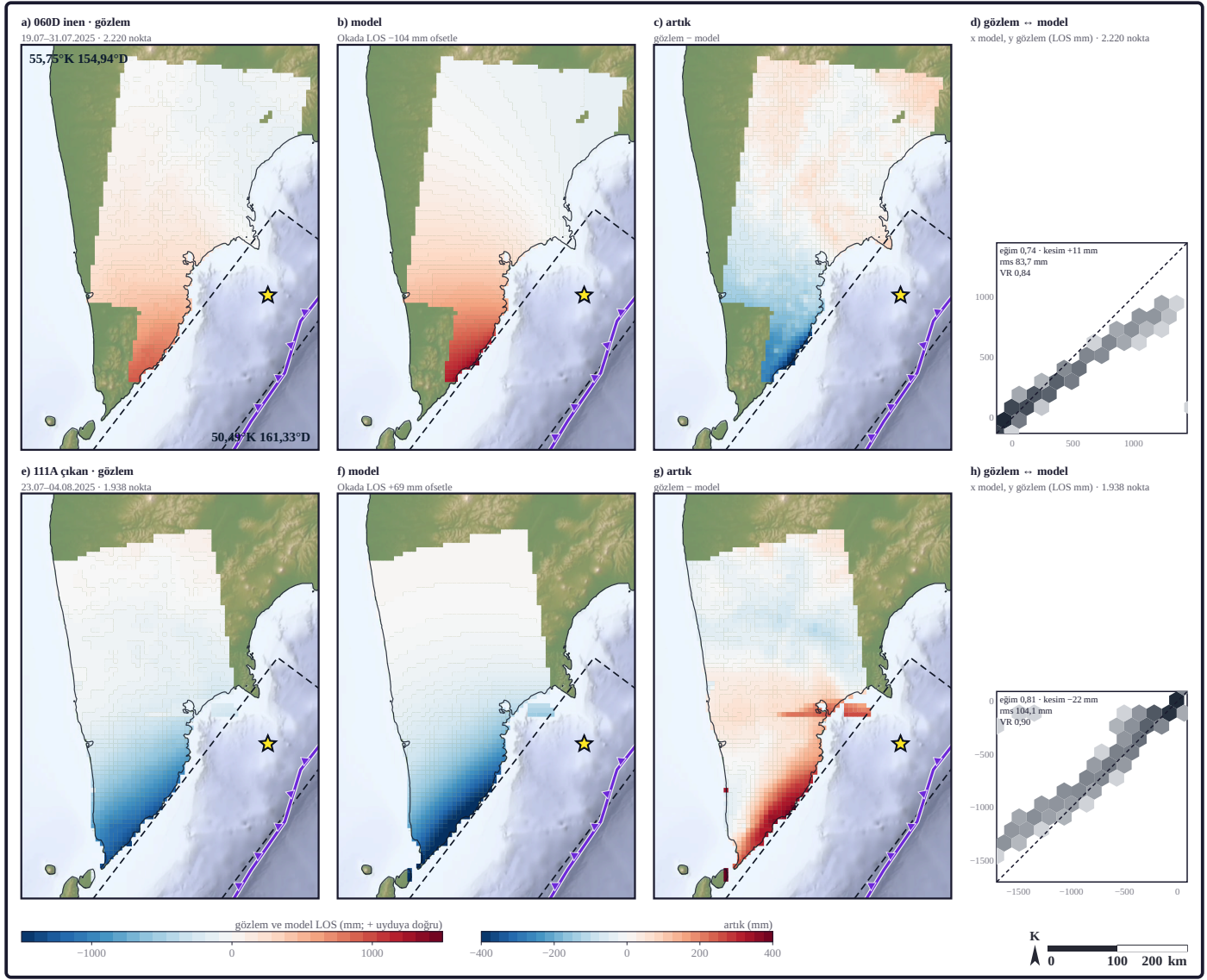
Şekil 26. a, e gözlem: Sentinel-1 LOS (COMET-LiCSAR; düzenli alt örnek): 060D 2.220, 111A 1.938 nokta; b, f model: USGS NEIC us6000qw60 (ürün tarihi 19.11.2025), Okada (1985) homojen yarı uzay LOS + iz başına sabit ötelenme (060D -104, 111A +69 mm; rampa ve katmanlı ortam yok); c, g artık: rms 060D 83,7, 111A 104,1 mm; gözlem ve model aynı ölçek ( \pm 1.500 mm; + uyduya doğru), artık ayrı \pm 400 mm; d, h gözlem ↔ model saçılımı (kesikli 1:1) (InSAR: LiCSAR contains modified Copernicus Sentinel data 2025 analysed by the Centre for the Observation and Modelling of Earthquakes, Volcanoes and Tectonics [COMET]. LiCSAR uses JASMIN, the UK's collaborative data analysis environment [http://jasmin.ac.uk]; Copernicus Sentinel-1 verisi [değiştirilmiş] [Lazecký vd., 2020]; model: kurum ürünü: USGS NEIC sonlu fay modeli us6000qw60 [U.S. Geological Survey, 2017]; ileri hesap, artık ve saçılım oturtması: bu çalışma; altlık ve kıyı çizgisi: ETOPO 2022 [30" ızgara, NOAA NCEI, doi:10.25921/fd45-gt74]; renk: oleron [Cramer, 2018a, 2018b]).
