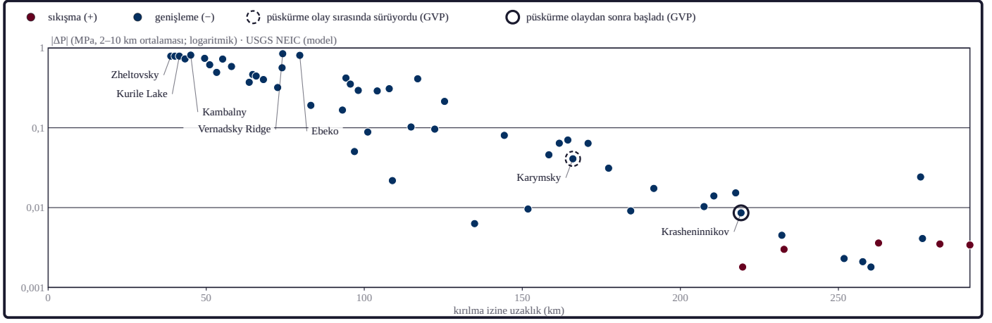
Şekil 23. 58 volkanın kırılma izine uzaklığına göre altındaki eşismik kaya basıncı değişiminin büyüklüğü ( |\Delta P| , 2–10 km derinlik ortalaması; logaritmik eksen); basınç MODEL çıktısıdır: USGS NEIC kayma modeliyle. Nokta rengi işareti verir: koyu kırmızı sıkışma (+), koyu mavi genişleme (-). İnce yatay çizgiler logaritmik |\Delta P| ekseninin onluk ızgarasıdır; eşik ya da başvuru değeri değildir. Dolu daire olay penceresinde püskürme kaydı olmayan volkanlar; halka GVP püskürme durumudur (düz halka olaydan sonra başlayan, kesikli halka olay sırasında süren). Adı yazılanlar |\Delta P| 'si en büyük 5 volkan ve püskürme kaydı olan 2 volkan. Öbür imler Şekil 6d ve 22'deki gibidir (volkanlar ve püskürmeler: Global Volcanism Program, Smithsonian Institution; basınç: bu çalışma [model; Okada, 1992]; model: kurum ürünü: USGS NEIC sonlu fay modeli us6000qw60 [U.S. Geological Survey, 2017]).
