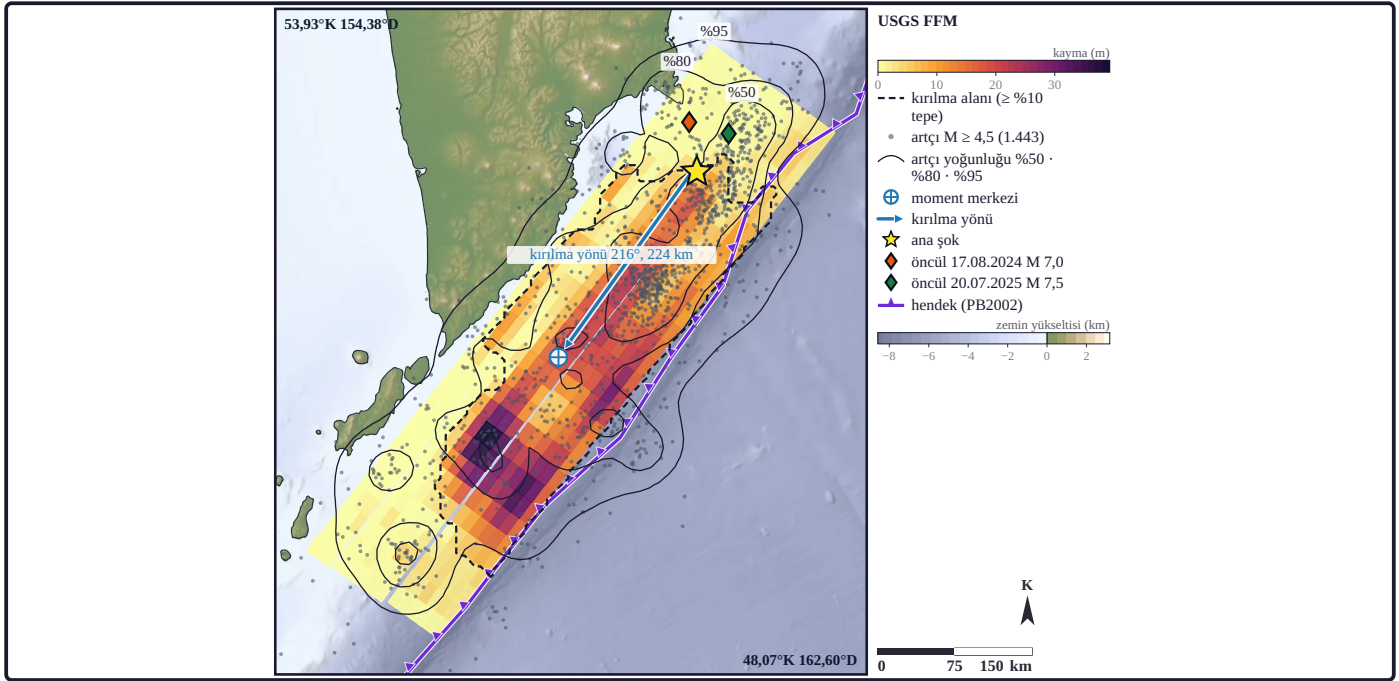
Şekil 13. Renkli dörtgenler USGS NEIC us6000qw60 (ürün tarihi 19.11.2025) yamaları (kayma 0–39,3 m; model çıktısı); kesikli siyah çizgi kırılma alanı (kayma \geq 3,9 m); gri noktalar M \geq 4,5 artçılar ( n = 1.443 ); ince siyah eğriler yoğunluğun %50, %80 ve %95 kütle sınırları; mavi artılı daire moment merkezi, mavi ok kırılma yönü 216^\circ , 224 km; sarı yıldız ana şok, elmaslar büyük öncüller (model: kurum ürünü: USGS NEIC sonlu fay modeli us6000qw60 [U.S. Geological Survey, 2017]; artçılar: USGS NEIC [ComCat] [U.S. Geological Survey, 2017]; kırılma alanı, artçı yoğunluğu, moment merkezi: Seismo Lab hesabı; levha sınırı: Bird, 2003 [iz, ETOPO 2022 hendek ekseninden ortalama \approx 12 km kara yönünde]; altlık ve kıyı çizgisi: ETOPO 2022 [30" ızgara, NOAA NCEI, doi:10.25921/fd45-gt74]; renk: oleron [Crameri, 2018a, 2018b]).
