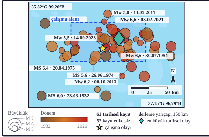
Şekil 8a. Çalışma olayından önceki eşik üstü kayıtlarda daire çapı büyüklüğü, dolgu rengi oluş dönemi gösterir. Turkuaz elmas derlemenin en büyük kaydı, sarı yıldız çalışmaya aittir. Kayıt eşiği yakın kuşakta M \geq 5 , bölge kuşağında M \geq 6 olarak alınmıştır. Mavi kesikli dikdörtgen çalışma alanıdır (birleşik katalog, 1900 sonrası; derleme yarıçapı 150 km, yakın kuşak 60 km).
