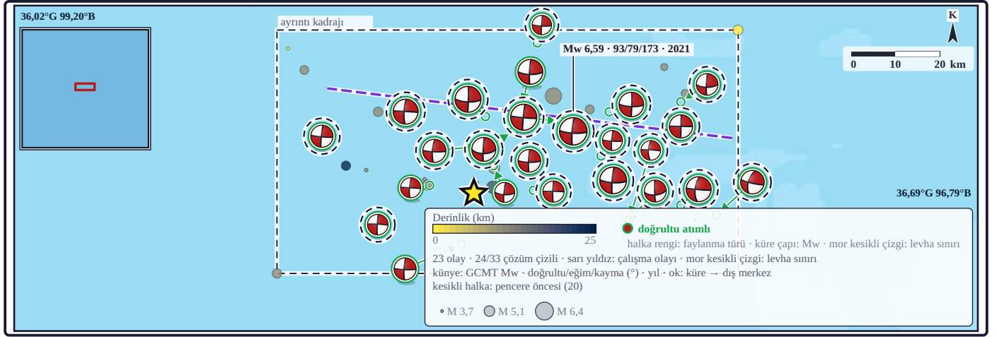
Şekil 8c. Bölgesel odak mekanizması çerçevesi: harita, çevrede yayımlanmış çözümlerin Mw sırasıyla en büyüklerini gösterir; ötelenen küreler okla konumlarına bağlıdır. Küreler alt yarıküre izdüşümünde odak mekanizmalarıdır; kırmızı kadrantlar P dalgasının ilk hareketinin itme olduğu bölgelerdir. Mw sırasıyla en büyük 1 çözüm künyelidir (öbür 23 küre künyesizdir); künye çözümün moment büyüklüğünü (GCMT Mw), bir düğüm düzleminin doğrultu, eğim ve kayma açısını ve yalını verir. Küçük daireler pencere olayları, kesikli dikdörtgen ayrıntı haritasının kadrantıdır (mekanizma kümesi: bölgesel küme [ n = 33 ]; gerilme inversiyonu olay merkezli mekanizma popülasyonundandır [ n = 80 ]; haritalanmış fay izi yok; mor kesik: levha sınırı [Bird 2003]).
