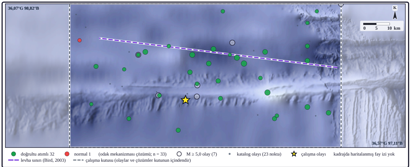
Şekil 5c. Haritada odak mekanizması çözümleri gösterilmiştir. Renkli dairelerde renk mekanizma sınıfını, çap büyüklüğü kodlar. İç boş halkalar M \geq 5,0 olayları, küçük gri noktalar katalog sismisitesini, sarı yıldız çalışma olayının dış merkezini gösterir; kesikli mor çizgiler Bird (2003) levha sınırlarıdır (GCMT mekanizmaları; levha sınırları: Bird, 2003).
