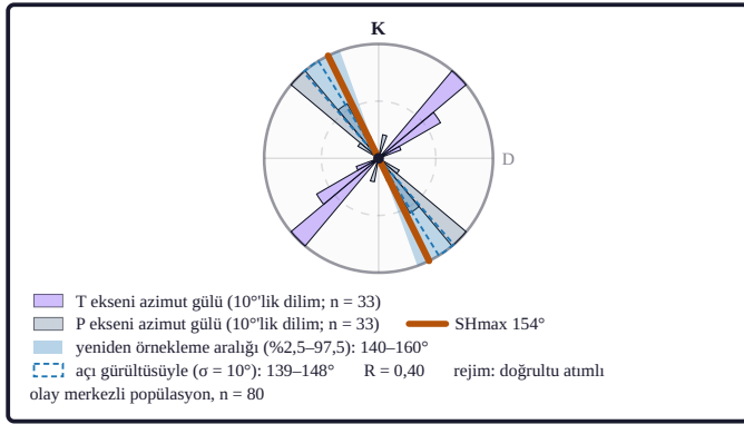
Şekil 5a. SHmax = 154° (yön iyi kısıtlı); rejim doğrultu atımlı faylanmadır (olay merkezli mekanizma popülasyonunun gerilme inversiyonu). Kuzeyi yukarıda olan gül diyagramında turuncu çift uçlu eksen gerilme inversiyonundan bulunan SHmax azimutunu, mavi yelpaze bu azimutun %2,5-97,5 yüzdelik aralığını (eksenel olduğundan karşı ucuyla birlikte) gösterir. Kesikli mavi sınır, her mekanizmanın doğrultu, eğim ve kayma açısına \sigma = 10^\circ 'lik rastgele gürültü de eklenerek yinelenen tersinin aynı yüzdelik aralığıdır (Vavryčuk, 2014). Gri sektörler bölgesel mekanizma kümesinin P eksenini (kısalma), mor sektörler T eksenini (uzama) azimut güllüdür (10°'lik dilimler; yarıçap sayının kareköküyle orantılı, iki gül ortak ölçekte). İç kesikli çember yarı ölçek halkasıdır; şekil oranı R ve rejim sınıfı lejantıdır (SHmax yönü: Lund ve Townend, 2007; rejim sınıfı: Dünya Gerilme Haritası kuralı).
