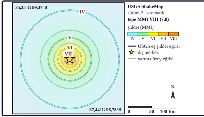
Şekil 6a. Harita USGS ShakeMap model kestiriminin (sürüm 2; otomatik ürün; 29.10.2026) eş şiddet (MMI) eğrilerini gösterir; ince eğriler yarım düzeylerdir; bu sürümde sismik istasyon kaydı yoktur; şiddet gözlemi de yoktur; alan yalnız yer hareketi bağıntılarından kurulmuştur; USGS belirsizlik derecesi --; yıldız dış merkezdir; renkli zemin orta çözünürlüklü USGS ShakeMap şiddet ılgarasının her 2. hücrelidir (kurum ürünü: USGS ShakeMap; yöntem: Wald ve Worden, 2020; Worden vd., 2018).
