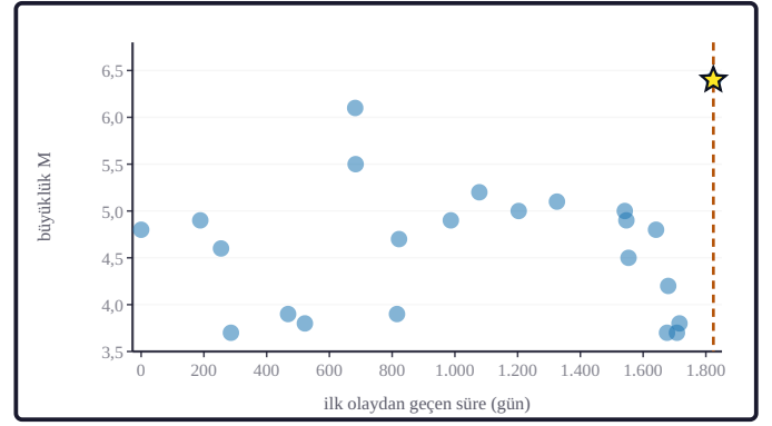
Şekil 2b. Pencere kataloğu 23 olaydır; en büyük olay çalışma olayıdır (Mw 6,4); M_c = 3,9 üstünde 18 olay vardır. Büyüklük–zaman dağılımı: yatay eksen ilk olaydan geçen süre (gün), dikey eksen büyüklüktür. Her mavi daire bir olaydır ve daire çapı büyüklükle ölçeklidir; turuncu kesikli dikey çizgi ve yıldız çalışma olayını işaretler.
