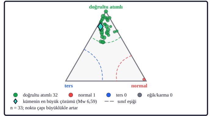
Şekil 5b. 33 çözümün %97'si doğrultu atımlı sınıfındadır (%95 Wilson aralığı %81-100; 23 bağımsız küme). Alt uç %70 baskınlık eşiklerinin üzerinde kaldığından bu sınıf baskın sayılmıştır. Bağımsız kümeler Gardner-Knopoff pencereleriyle ayrılmıştır. Frohlich üçgeninde her nokta bir odak mekanizması çözümünün P, T ve B eksenlerinin dalım açılarından gnomonik izdüşümle kurulan konumudur (köşeler: ters, normal, doğrultu atımlı). Renkli kesikli eğriler sınıf eşikleridir (B dalımı 60°, P dalımı 60°, T dalımı 50°); nokta rengi sınıfı, gri renk hiçbir eşik aşmayan eğik/karma çözümleri, nokta çapı büyüklüğü, turkuaz elmas kümedeki en büyük çözümü gösterir; sınıf sayımları lejantıdır (Frohlich, 1992 gnomonik üçgeni; Frohlich ve Apperson, 1992 eşikleri; çözümler: Global CMT, Ekström vd., 2012).
