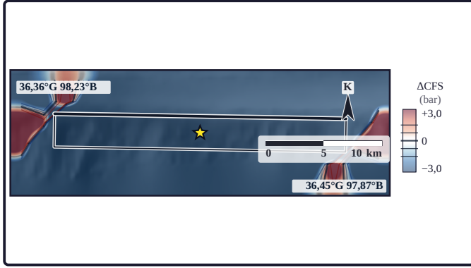
Şekil 4a. Harita statik Coulomb gerilme değişimini ( \Delta CFS ) gösterir (kırmızı artış, mavi azalma; \pm 3,0 bar). \Delta CFS Wells ve Coppersmith (1994) kaynağının kaynakla eş yönelimli alıcıda ( s/d/r = 91^\circ/72^\circ/173^\circ ), 10,0 km derinlikte, \mu' = 0,40 ile hesaplanmıştır. Yıldız dış merkezdir; dörtgen kaynağın yüzey izdüşümüdür (kalın kenar üstte); çizgiler \Delta CFS konturlarıdır. Mor çizgiler diri fay izleridir ( \Delta CFS : Okada, 1992; King vd., 1994; altlık [gri tonlu]: Batimetri: GMRT v4.5.0 [Global Multi-Resolution Topography] — Ryan, W.B.F. ve ark., 2009, Geochem. Geophys. Geosyst. 10, Q03014, doi:10.1029/2008GC002332 · Lamont-Doherty Earth Observatory / MGDS, CC-BY-4.0 · Renk skalası: oleron [bilimsel, sıfır-çapalı] — Crameri, F. [2018] Zenodo doi:10.5281/zenodo.1243862 · Crameri [2018] Geosci. Model Dev. 11, 2541–2562 · Crameri, Shephard & Heron [2020] Nature Communications 11, 5444 · Batimetri: GMRT v4.5.0 [Global Multi-Resolution Topography] — Ryan, W.B.F. ve ark., 2009, Geochem. Geophys. Geosyst. 10, Q03014, doi:10.1029/2008GC002332 · Lamont-Doherty Earth Observatory / MGDS, CC-BY-4.0 · Kabartma: AWS Terrain Tiles [Mapzen terrarium] — kaynak ve lisanslar: github.com/tilezen/joerd/blob/master/docs/attribution.md ).
