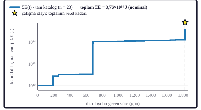
Şekil 3b. Mavi basamak eğrisi kümülatif ısıran sismik enerjidir ( \Sigma E , logaritmik eksen). Kesikli düşey çizgi çalışma olayını işaretler; en büyük tek katkı bu olaydır (Gutenberg ve Richter, 1956 enerji bağıntısı).
