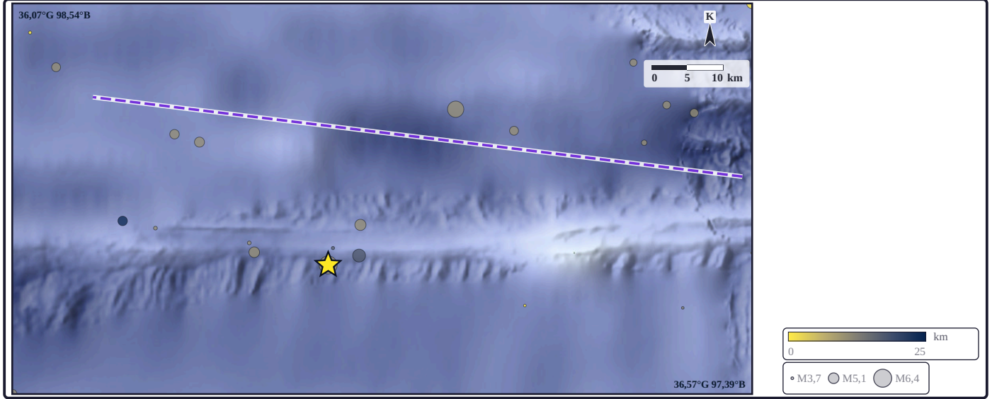
Şekil 7. Harita 23 olaylık kataloğun tamamını gösterir; en büyük olay çalışma olayıdır (Mw 6,4). Bölge haritası: yıldız çalışma olayının dış merkezidir; olaylar derinlikle renkli (sıfır sarı, derin lacivert), daire çapı büyüklükle ölçeklidir; çizgiler diri fay izleridir (haritalanmış fay izi yok; mor kesik: levha sınırı [Bird 2003]; mekanizmalar: bölgesel mekanizma kümesi; katalog: ISC · USGS · GFZ; altlık: Batimetri: GMRT v4.5.0 [Global Multi-Resolution Topography] — Ryan, W.B.F. ve ark., 2009, Geochem. Geophys. Geosyst. 10, Q03014, doi:10.1029/2008GC002332 · Lamont-Doherty Earth Observatory / MGDS, CC-BY-4.0 · Renk skalası: oleron [bilimsel, sıfır-çapalı] — Crameri, F. [2018] Zenodo doi:10.5281/zenodo.1243862 · Crameri [2018] Geosci. Model Dev. 11, 2541–2562 · Crameri, Shephard & Heron [2020] Nature Communications 11, 5444 · Batimetri: GMRT v4.5.0 [Global Multi-Resolution Topography] — Ryan, W.B.F. ve ark., 2009, Geochem. Geophys. Geosyst. 10, Q03014, doi:10.1029/2008GC002332 · Lamont-Doherty Earth Observatory / MGDS, CC-BY-4.0 · Kabartma: AWS Terrain Tiles [Mapzen terrarium] — kaynak ve lisanslar: github.com/tilezen/joerd/blob/master/docs/attribution.md ).
