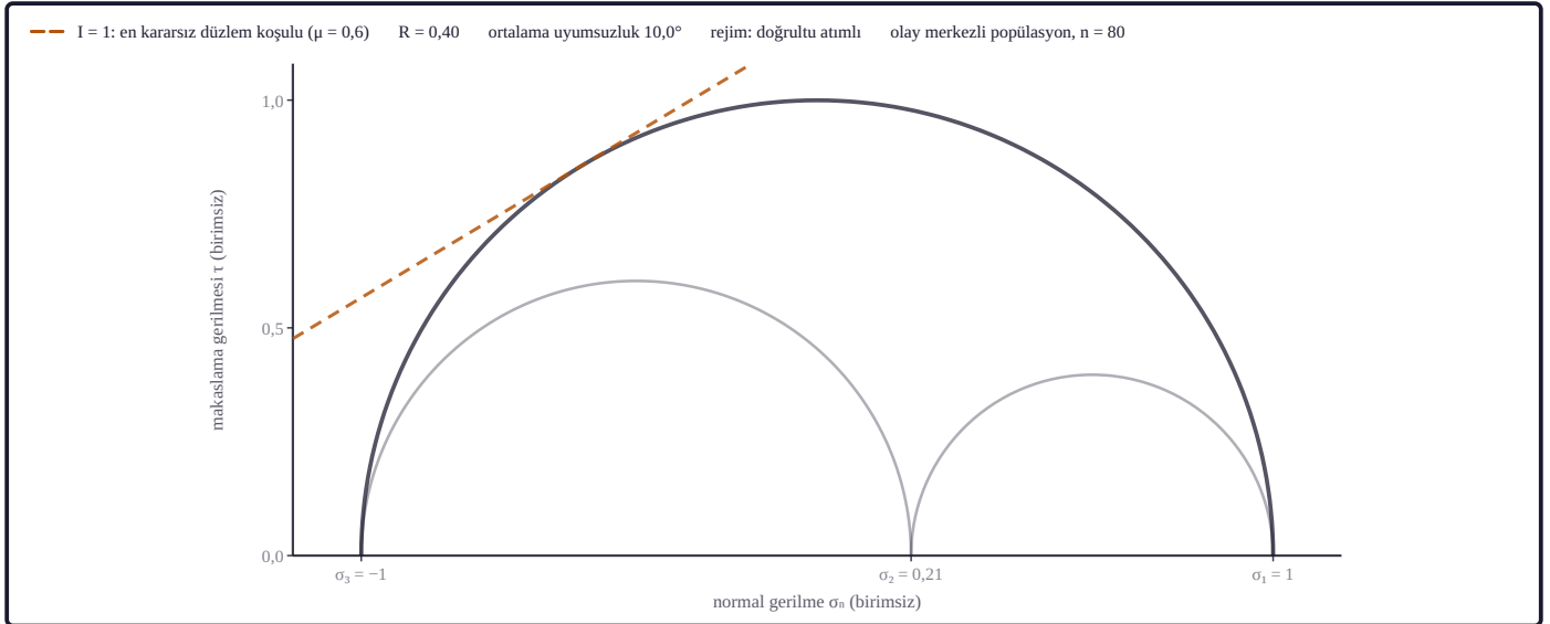
Şekil 4c. Gerilme inversiyonunun normalleştirilmiş Mohr diyagramında yatay eksen normal gerilme \sigma_n , dikey eksen makaslama gerilmesi \tau 'dur. Üç yarım çember asal gerilmelerle kurulan gerilme durumunu, turuncu kesikli doğru \mu sürtünme katsayısıyla tanımlı en kararsız düzlem koşulunu (kararsızlık indeksi I = 1 ) gösterir; çalışma olayının odak mekanizması çözümü bulunmadığından düğüm düzlemi noktaları çizilmemiştir. Şekil oranı R ve ortalama kayma yönü uyumsuzluğu lejjantıdır (Vavryčuk, 2014; kararsızlık ölçütü).
