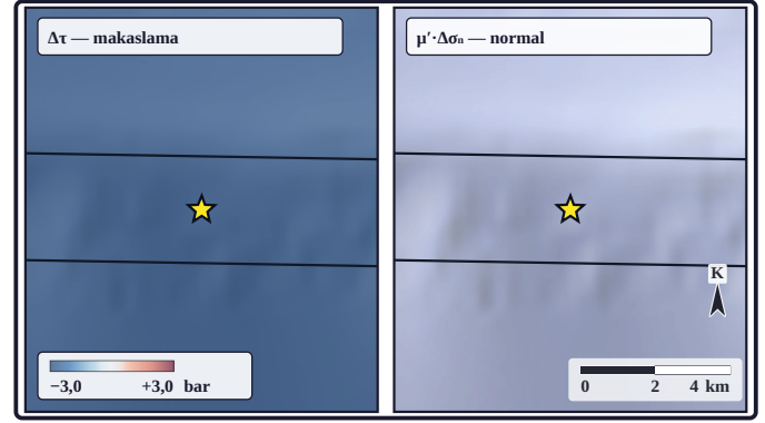
Şekil 4b. \Delta CFS 'in iki bileşeni ayrı panellerde gösterilmiştir: solda makaslama gerilmesi değişimi \Delta\tau , sağda fay düzlemine dik normal gerilme katkısı \mu'\Delta\sigma_n ( \Delta CFS = \Delta\tau + \mu'\Delta\sigma_n ; \Delta\sigma_n çekme artı, artı değer fayın kenetlenmesinin azalmasıdır). Kadraj kaynak çevresine yaklaştırılmıştır; renk ölçeği ve kaynak geometrisi \Delta CFS haritasıyla aynıdır; yıldız dış merkezdir; ince dörtgen kaynağın yüzey izdüşümüdür (bileşen ayrışımı: Okada, 1992 analitik çözümü).
