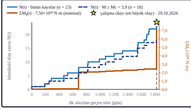
Şekil 3a. Mavi eğri kümülatif olay sayısı N(t) , turuncu eğri kümülatif sismik moment \Sigma M_0(t) değeridir. Sarı yıldız çalışma olayıdır; pencerede en büyük olay da odur ( M_0 = 10^{18}[1,5 \cdot M + 9,1] N·m; 9,1 sabiti Kanamori, 1977).
