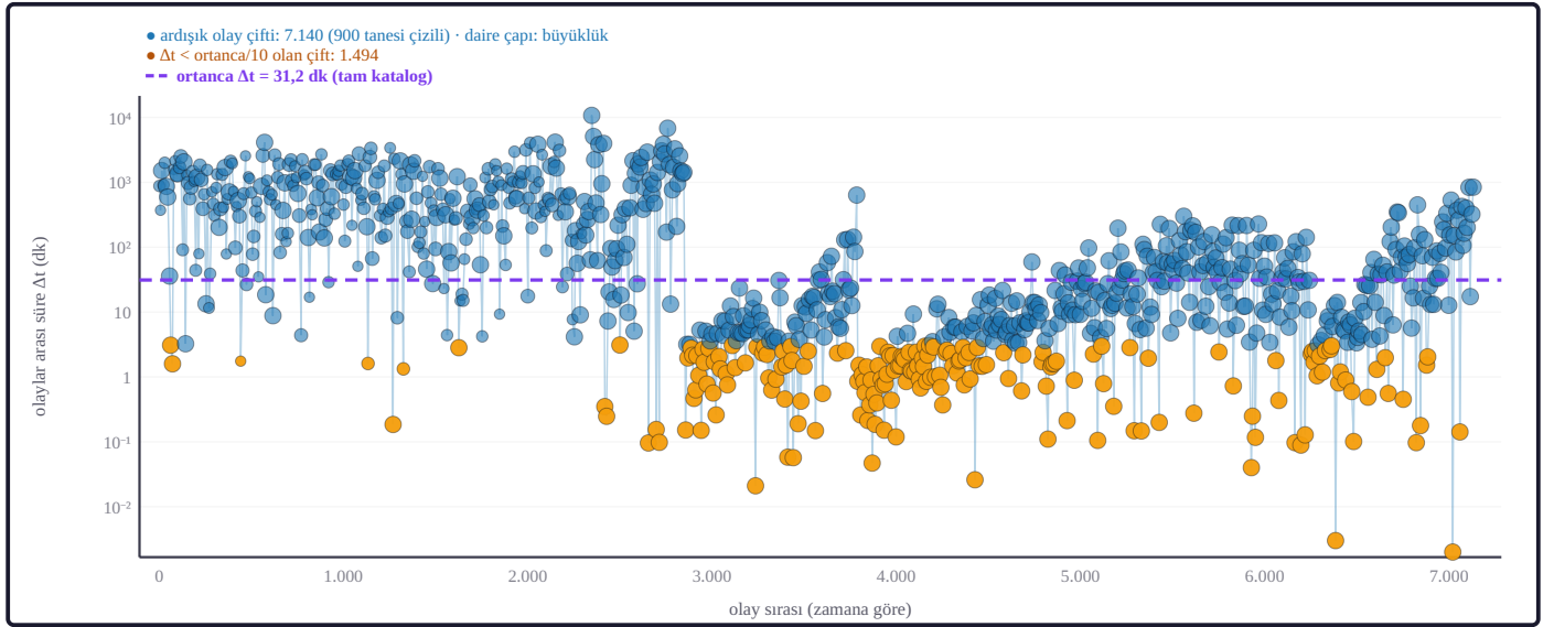
Şekil 6c. Düşey eksen bir önceki olaydan geçen süredir (dakika, logaritmik). Mor çizgi ortalama süredir; turuncu daireler ortancanın onda birinden kısa aralıklardır. Daire çapı büyüklükle artar (seri: tekilleştirilmiş tam katalog).
