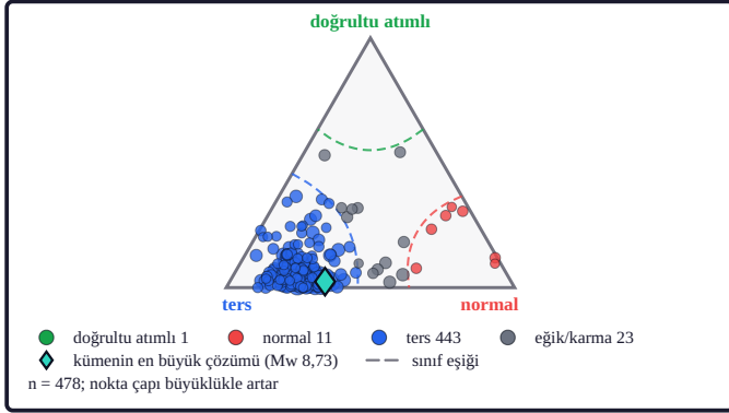
Şekil 8c. 478 çözümün %93'ü ters sınıfındadır (%95 Wilson aralığı %85–97; 84 bağımsız küme). Alt uç %70 baskınlık eşiğinin üzerinde kaldığından bu sınıf baskın sayılmıştır. Bağımsız kümeler Gardner–Knopoff pencereleriyle ayrılmıştır. Frohlich üçgeninde her nokta bir odak mekanizması çözümünün P, T ve B eksenlerinin dalım açılarından gnomonik izdüşümü kurulan konumudur (köşeler: ters, normal, doğrultu atımlı). Renkli kesikli eğriler sınıf eşikleridir (B dalımı 60°, P dalımı 60°, T dalımı 50°); nokta rengi sınıfı, gri renk hiçbir eşiği aşmayan eğik/karma çözümleri, nokta çapı büyüklüğü, turkuaz elmas kümedeki en büyük çözümü gösterir; sınıf sayımları lejantıdır (Frohlich, 1992 gnomonik üçgeni; Frohlich ve Apperson, 1992 eşikleri; çözümler: Global CMT, Ekström vd., 2012).
