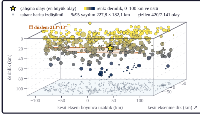
Şekil 4a. Yatay eksen kesit eksen (kutu yayılımının uzun eksenini) boyunca, sağ üste kaçan eksen ona dik uzaklığı, düşey eksen derinliği verir. Derinlik eksen kesitlerle aynıdır; turuncu levha oturtulan düzlemdir. Yıldızdan üst yüze çıkan kesikli çizgi olayın yüzeydeki izdüşümünü gösterir (kabinet izdüşümü; üç eksen ayrı ölçeklidir; blok kenarları %95 yayılımın 1,06 katıdır).
