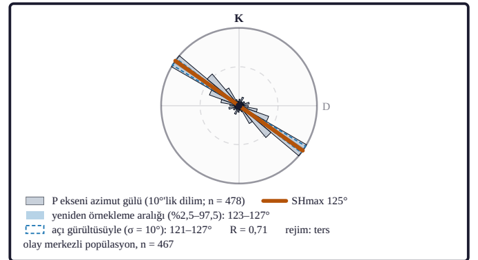
Şekil 7d. SH_{max} = 125^\circ (yön iyi kısıtlı); rejim ters faylanmadır (olay merkezli mekanizma popülasyonunun gerilme inversiyonu). Kuzeyi yukarıda olan gül diyagramında turuncu çift uçlu eksen gerilme inversiyonundan bulunan SH_{max} azimutunu, mavi yelpaze bu azimutun %2,5–97,5 yüzdelik aralığını (eksenel olduğundan karşı ucuyla birlikte) gösterir. Kesikli mavi sınır, her mekanizmanın doğrultu, eğim ve kayma açısına \sigma = 10^\circ 'lik rastgele gürültü de eklenerek yinelenen tersininin aynı yüzdelik aralığıdır (Vavryčuk, 2014). Gri sektörler bölgesel mekanizma kümesinin P eksen (kısalma) azimut güldür (10°'lik dilimler; yarıçap sayımın kareköküyle orantılı). İç kesikli çember yarı ölçek halkasıdır; şekil oranı R ve rejim sınıfı lejantıdır ( SH_{max} yönü: Lund ve Townend, 2007; rejim sınıfı: Dünya Gerilme Haritası kuralı).
