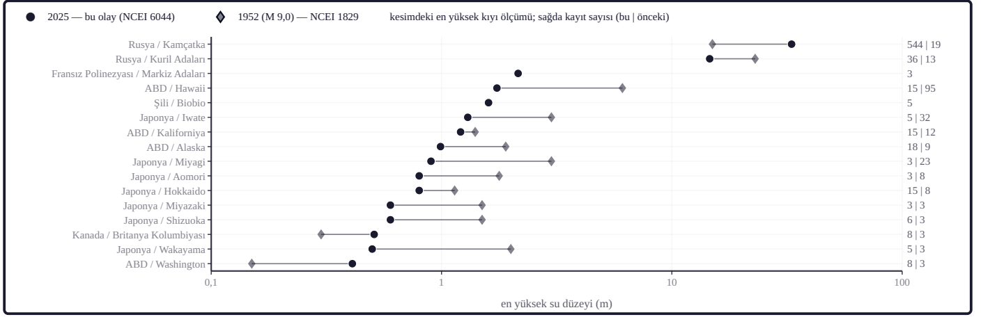
Şekil 31a. Ülke / bölge kesimlerinde NCEI'nin kıyı ölçümlerinin en yüksek değeri (logaritmik eksen); yalnız en az 3 ölçümü olan kesimler, şüpheli (doubtful) ve DART kayıtları hariç. Gri karo 1952 olayının (NCEI 1829, M 9,0) aynı kesimdeki değeridir ve yalnız iki olayda da en az 3 ölçümü olan 14 kesimde çizilir. Bu olayın en az 3 ölçümlü 28 kesiminden 16'sı gösterilmiştir (yükteki kesim listesi en yüksek değerli kesimlerle sınırlıdır). Sağdaki sayılar kesimdeki ölçüm sayısıdır; değerler gözlemdir, model değildir. Kesim değerleri tek tek kıyı gözlemlerinin en büyüğüdür; NCEI olay kaydının en büyük su yüksekliği alanı 17,0 m'dir (iki alan NCEI'nin ayrı tablolarıdır). Karolar kesimdeki en yüksek ölçümü NCEI ölçüm türü ayrılmadan gösterir; metindeki olaylar arası kesim sayımı ise aynı ölçüm türü kodlu kayıtlarla, iki olayda da en az 3 kaydı olan 7 kesimde yapılır (veri: NCEI/WDS Global Historical Tsunami Database [doi:10.7289/V5PN93H7]).
