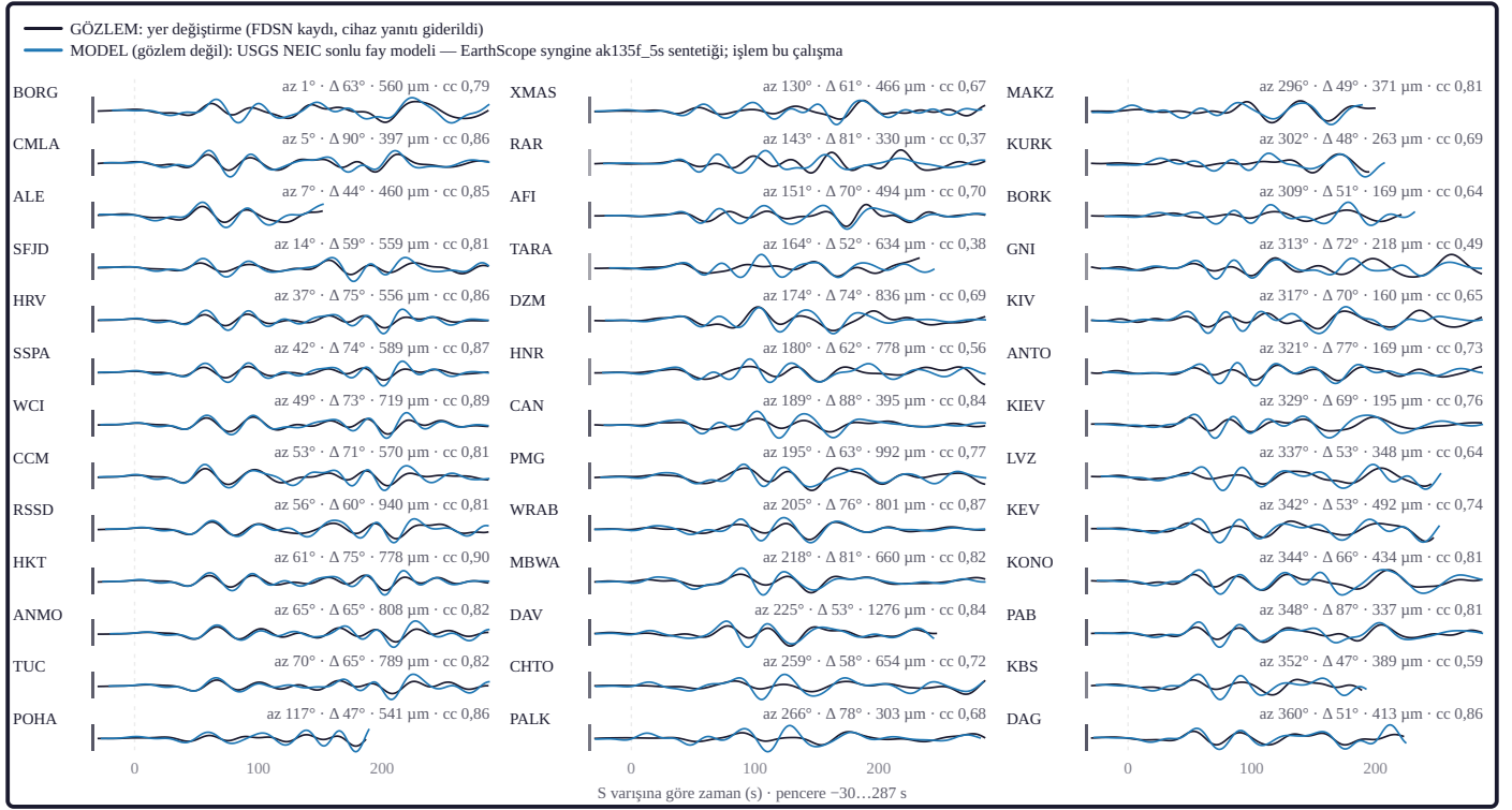
Şekil 17. 39 telesismik istasyonda (30–90°; açılar G , GE , II , IU ) SH dalgası enine ( T ; yataylar istasyondan kaynağa azimutla döndürüldü) bileşen yer değiştirmesi: siyah GÖZLEM (EarthScope veri hizmetleri), mavi MODEL — USGS NEIC sonlu fay modeli için EarthScope syngine ak135f_5s sentetiği (sentetik syngine hizmetinde hesaplandı; işlem bu çalışma). SH sentetiği, kurum ürünü kayma modelinin yamalarının syngine sonlu fay yoluyla toplanmasıdır. SH kayıtları cihaz yanıtı giderilip 25–100 s bandında (Butterworth, sıfır fazlı) süzüldü; alt sınır, sentetiği kurulan sonlu fay modelinin alt fay boyutundan türetili ( \Delta 20 km; T \geq 4 \cdot \Delta / \beta , \beta 3,75 km/s): sentetik her alt fayı tek nokta kaynakla temsil ettiğinden daha kısa periyotta yapay enerji taşır. SH penceresi, Love dalgası girmeden kesildi. SH izlerinin zaman eksenini IASP91 S varışına göre (-30...287 s); sentetik, ilintiyi en büyük yapan zaman ötelemesiyle ( \pm 15 s içinde) kaydırılarak çizildi. SH izlerinde solda istasyon kodu, sağ üstte azimut, uzaklık (°), gözlemin tepe genişliği ( \mu\text{m} ; bu çalışmanın süzgeciyle) ve ilinti katsayısı (cc); izin solundaki ince çubuk cc arttıkça açık griden koyu griye döner. Uyum (39 iz): kaydırılmış sentetik ile ilinti ortancası 0,81 (çeyrekler 0,68–0,84), kaymasız 0,62; varyans azalımı ortancası 0,08; genlik oranı (gözlem / sentetik, RMS) ortancası 0,69. Öteki kaynakların ilinti ortancası (çizilmedi): GCMT C202507292324B nokta kaynak \geq 0,31 (21 / 39 izde kayma \pm 15 s arama sınırına dayandı; değer alt sınırdır); USGS W-fazı (Mww) nokta kaynak 0,42 (veri: EarthScope Consortium veri hizmetleri [eski IRIS DMC] [FDSN dataset]; cihaz yanıtı: EarthScope FDSN station hizmeti; açılar G [doi:10.18715/GEOSCOPE.G], GE [doi:10.14470/TR560404], II [doi:10.7914/SN/II], IU [doi:10.7914/SN/IU]; sentetik: EarthScope syngine [doi:10.17611/DP/SYNGINE.1; Krischer vd., 2017; Nissen-Meyer vd., 2014; van Driel vd. 2015], ak135f_5s [ak135: Kennett vd., 1995; yoğunluk ve Q : Montagner ve Kennett, 1996]; kurum ürünü: USGS NEIC sonlu fay modeli us6000qw60 [U.S. Geological Survey, 2017]; varış: IASP91 [Kennett ve Engdahl 1991]; işlem: bu çalışma).
