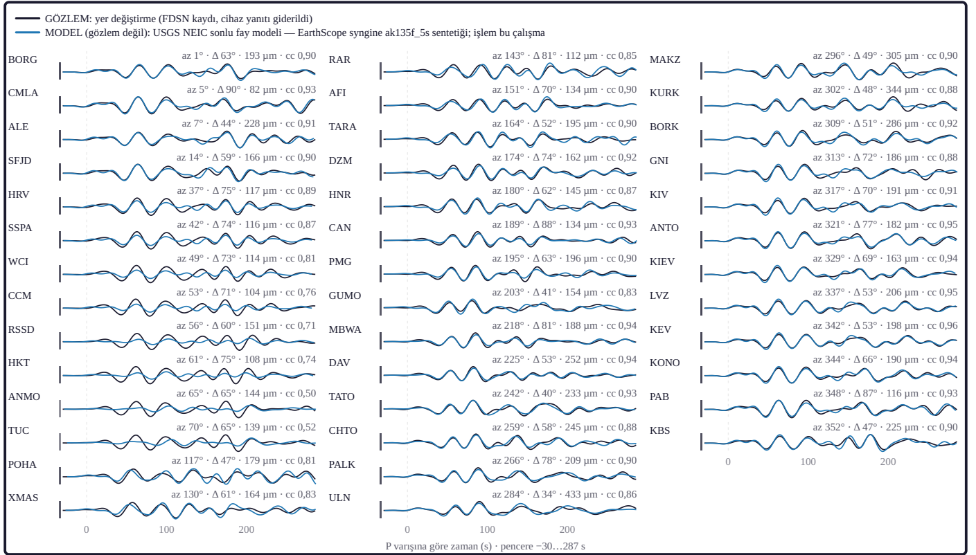
Şekil 16. 40 telesismik istasyonda (30–90°; açılar G, GE, II, IU) P dalgası düşey (Z) bileşen yer değiştirmesi: siyah GÖZLEM (EarthScope veri hizmetleri), mavi MODEL — USGS NEIC sonlu fay modeli için EarthScope syngine ak135f_5s sentetiği (sentetik syngine hizmetinde hesaplandı; işlem bu çalışmada). Sentetik, kurum ürünü kayma modelinin yamalarının syngine sonlu fay yoluyla toplanmasıdır (yama başına zaman kaydırmalı asimetrik kosinüs kayma hızı; Green işlevleri syngine veritabanının küresel yer modelindendir). P kayıtları cihaz yanıtı giderilip 25–100 s bandında (Butterworth, sıfır fazlı) süzülür; alt sınır, sentetiği kurulan sonlu fay modelinin alt fay boyutundan türetilir ( \Delta 20 km; T \geq 4 \cdot \Delta / \beta , \beta 3,75 km/s); sentetik her alt fayı tek nokta kaynakla temsil ettiğinden daha kısa periyotta yapay enerji taşır. P izlerinin zaman eksenini IASP91 P varışına göre (-30...287 s); sentetik, ilintiyi en büyük yapan zaman ötelemesiyle ( \pm 10 s içinde) kaydırılarak çizildi. P izlerinde solda istasyon kodu, sağ üstte azimut, uzaklık (°), gözlemin tepe genliği ( \mu\text{m} ; bu çalışmanın süzgeciyle) ve ilinti katsayısı (cc); izin solundaki ince çubuk cc arttıkça açık griden koyu griye döner. Uyum (40 iz): kaydırılmış sentetik ilinti ortancası 0,90 (çeyrekler 0,85–0,93), kaymasız 0,88; varyans azalımı ortancası 0,79; genlik oranı (gözlem / sentetik, RMS) ortancası 1,06. Öteki kaynakların ilinti ortancası (çizilmedi): GCMT C202507292324B nokta kaynak \geq 0,22 (26 / 40 izde kayma \pm 10 s arama sınırına dayandı; değer alt sınırdır); USGS W-fazı (Mww) nokta kaynak \geq 0,26 (39 / 40 izde kayma \pm 10 s arama sınırına dayandı; değer alt sınırdır) (veri: EarthScope Consortium veri hizmetleri [eski IRIS DMC] [FDSN dataset]; cihaz yanıtı: EarthScope FDSN station hizmeti; açılar G [doi:10.18715/GEOSCOPE.G], GE [doi:10.14470/TR560404], II [doi:10.7914/SN/II], IU [doi:10.7914/SN/IU]; sentetik: EarthScope syngine [doi:10.17611/DP/SYNGINE.1; Krischer vd., 2017; Nissen-Meyer vd., 2014; van Driel vd. 2015], ak135f_5s [ak135: Kennett vd., 1995; yoğunluk ve Q: Montagner ve Kennett, 1996]; kurum ürünü: USGS NEIC sonlu fay modeli us6000qw60 [U.S. Geological Survey, 2017]; varış: IASP91 [Kennett ve Engdahl 1991]; işlem: bu çalışma).
