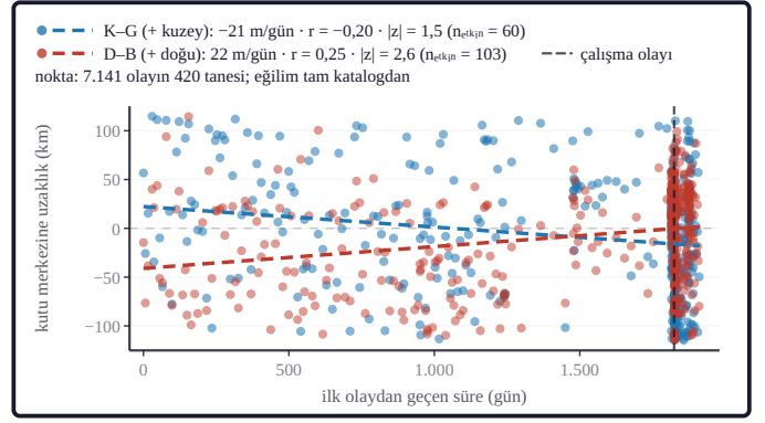
Şekil 4b. Dış merkez koordinatlarının zaman serisinde mavi noktalar kuzey-güney, kırmızı noktalar doğu-batı bileşenidir. Yatay eksen penceresinin ilk olayından geçen süre (gün), düşey eksen kutu merkezine uzaklıktır (km); iki bileşen aynı ölçekte olduğundan eğimleri doğrudan kıyaslanabilir. Kesikli doğrular her bileşenin en küçük kareler eğilimidir; eğim, Pearson korelasyon katsayısı ve etkin örneklem büyüklüğüyle hesaplanan Fisher z değeri lejantıdır. Düşey kesikli çizgi çalışma olayının anımı işaretler.
