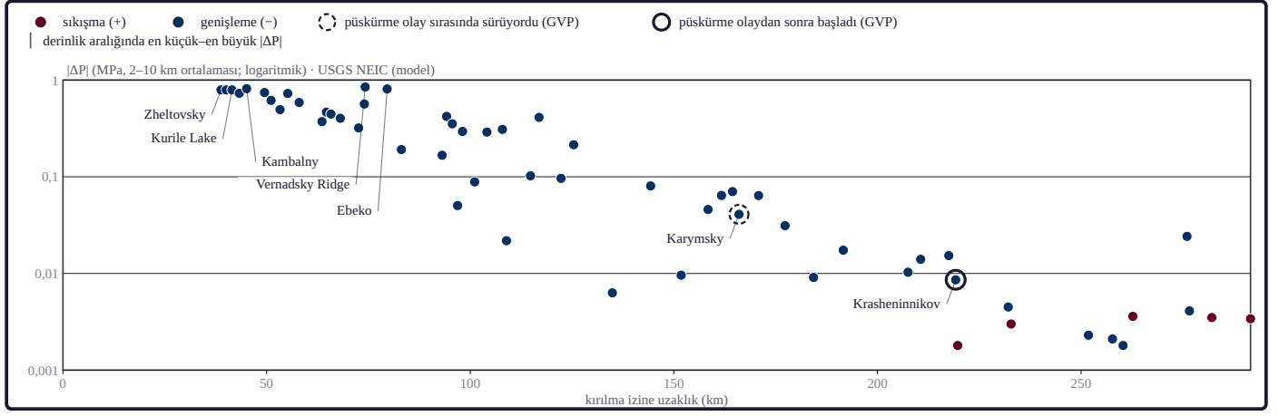
Şekil 23. 58 volkanın kırılma izine uzaklığına göre altındaki eşismik kaya basıncı değişiminin büyüklüğü ( \Delta P ), 2–10 km derinlik ortalaması; logaritmik eksen); basınç MODEL çıktısıdır; USGS NEIC kayma modeliyle. Nokta rengi işareti verir: koyu kırmızı sıkışma (+), koyu mavi genişleme (-). Dikey çizgi 2–10 km arasındaki derinliklerde en küçük ve en büyük \Delta P 'dir. Dolu daire olay penceresinde püskürme kaydı olmayan volkanlar; halka GVP püskürme durumudur (düz halka olaydan sonra başlayan, kesikli halka olay sırasında süren). Adı yazılanlar \Delta P 'si en büyük 5 volkan ve püskürme kaydı olan 2 volkan. Öbür imler Şekil 6d ve 22'deki gibidir (volkanlar ve püskürmeler: Global Volcanism Program, Smithsonian Institution; basınç; bu çalışma [model; Okada, 1992]; model: kurum ürünü: USGS NEIC sonlu fay modeli us6000qw60 [U.S. Geological Survey, 2017]).
