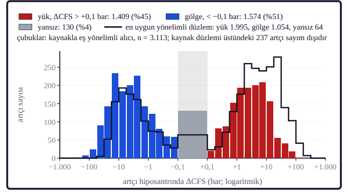
Şekil 8b. Coulomb nokta sınaması, artçıların kendi hiposantrlarında hesaplanan \Delta CFS değerlerinin dağılımını verir. Artçı konum belirsizliği sayımlara yansıtılmamıştır. Kırmızı çubuklar yük artışı, mavi çubuklar gerilme gölgesini, gri bant iki eşik arasındaki yansız aralığı gösterir; çizgi en uygun yönelimli düzlem için aynı dağılımdır (eşik 0,1 bar = 0,01 MPa: Hardebeck vd., 1998; kurum ürünü: USGS NEIC sonlu fay modeli us6000qw60 [U.S. Geological Survey, 2017]).
