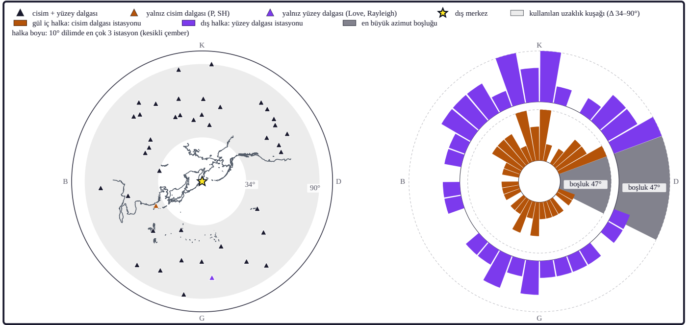
Şekil 12. Telesismik istasyonlar ve azimut kapsamı: solda dış merkezli azimutal eşuzaklık izdüşümünde 43 istasyon ve kullanılan uzaklık kuşağı (açık gri halka, \Delta 34–90°). Üçgenin rengi istasyonun kullanıldığı dalga grubudur (siyah: cisim ve yüzey dalgası, 40 istasyon; amber: yalnız cisim dalgası — P, SH, 2 istasyon; mor: yalnız yüzey dalgası — Love, Rayleigh, 1 istasyon). Sağdaki güldde 10°'lik azimut dilimlerinde istasyon sayısı: iç halka cisim dalgası (42 istasyon) ve dış halka yüzey dalgası (41 istasyon); gri kama grubun en büyük azimut boşluğudur. İstasyonlar G, GE, II, IU ağlarından her rolde azimut boşluğunu en aza indiren seçimle belirlendi (ölçüt: 30–90° uzaklık, iyi azimut kapsamı ve yüksek sinyal / gürültü); sinyal / gürültü oranı 3'ün altındaki, boşluklu ya da doygun kayıtlar elendi. En büyük azimut boşluğu cisim dalgasında 47° ve yüzey dalgasında 47° (rol başına P 47°, SH 47°, Love 47°, Rayleigh 47°). Kıyı çizgisi ETOPO 2022 ızgarasının 0 m eğrisidir; yalnız altlık ızgarasının kapsadığı kesimde çizildi (istasyon üstverisi: EarthScope FDSN station hizmeti; seçim, izdüşüm ve azimut kapsamı: bu çalışma; kıyı çizgisi [0 m eğrisi]: ETOPO 2022 [60" ızgara, 4 hücrede bir, NOAA NCEI, doi:10.25921/fd45-gt74]).
