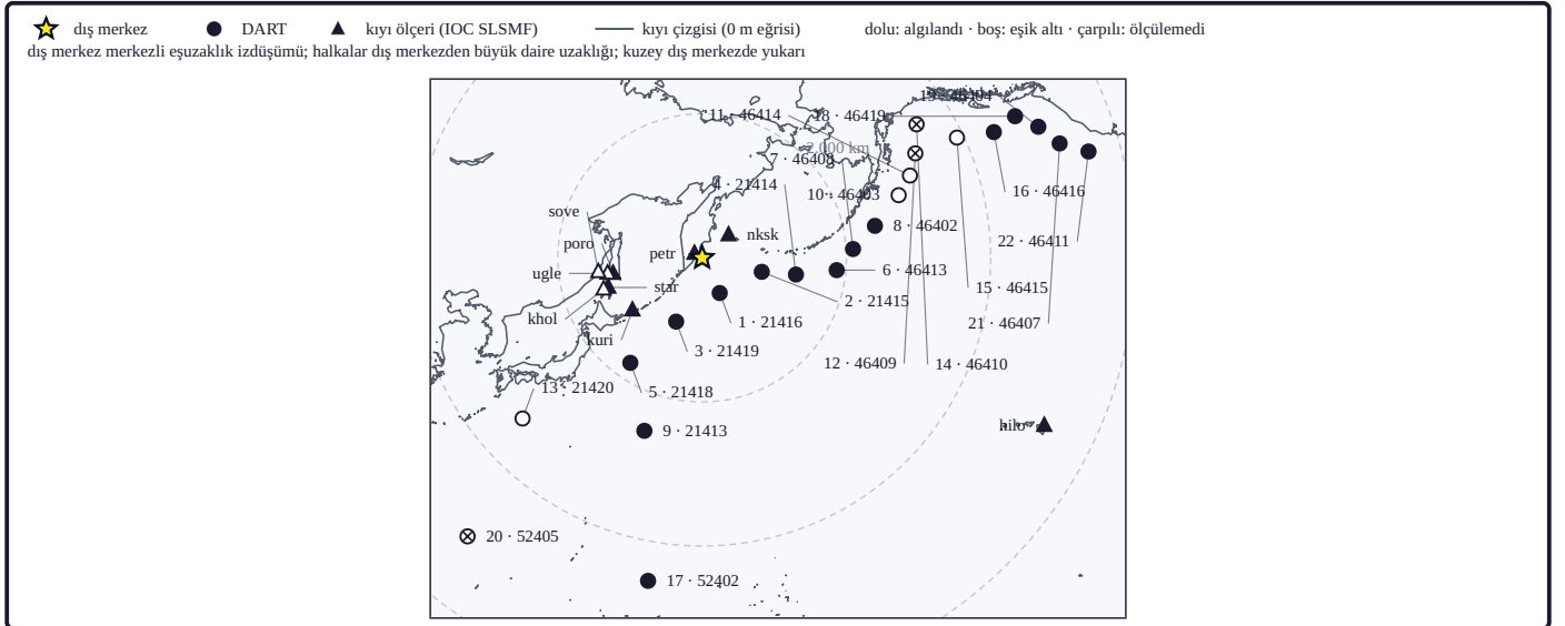
Şekil 30b. Tsunami gözlem istasyonlarının konumu: 22 DART (15 algıladı, 4 eşik altında kaldı, 3 ölçülemedi) ve 9 IOC kıyı ölçeri (6 algıladı, 3 eşik altında kaldı); en uzak istasyon 5.557 km. Konumlar IOC SLSMF istasyon kaydındaki güncel konuşlandırmadır (olay günündeki konum farklı olabilir); NCEI olay kaydındaki konumu 5 km'den farklı DART'lar: 21416 14 km (dış merkeze NCEI konumuyla 534 km, IOC kaydıyla 546 km); 21419 6 km (dış merkeze NCEI konumuyla 961 km, IOC kaydıyla 956 km); 46413 141 km (dış merkeze NCEI konumuyla 1.741 km, IOC kaydıyla 1.874 km); 52402 84 km (dış merkeze NCEI konumuyla 4.578 km, IOC kaydıyla 4.547 km). Ölçüm durumları bu çalışmanın ölçümüdür; DART kayıt kesiti ve DART çizelgesiyle aynı ölçümden gelir. DART etiketindeki ilk sayı dış merkez uzaklığına göre sıradır; DART kayıt kesitinde, tsunami modeli haritasında ve DART çizelgesinde aynı sıra kullanılır. Harita dış merkez merkezli eşuzaklık izdüşümüdür; halkalar dış merkezden büyük daire uzaklığıdır, yön yalnız dış merkezde geçerlidir; ince gri çizgi ETOPO 2022 ızgarasının (≈ 7 km hücre) 0 m eğrisidir (kıyı; gelgit kıyı çizgisi değildir; hücreden küçük adalar çizilemez) (konum: IOC Sea Level Station Monitoring Facility istasyon kaydı; ölçüm: NOAA NDBC DART / IOC SLSMF, işlem bu çalışmada; kıyı çizgisi [0 m eğrisi]: ETOPO 2022 [60" ızgara, 4 hücrede bir, NOAA NCEI, doi:10.25921/fd45-gt74]).
