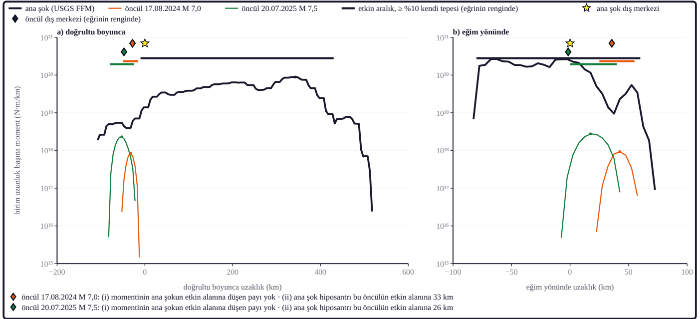
Şekil 14. Öncül ve ana şok kaymasının doğrultu ve eğim boyunca dağılımı: kalın siyah eğri ana şok (USGS FFM), renkli öncüller; 5 km kovada birim uzunluk başına moment (model çıktısı); a) 217° eksenli, b) eğim yönü; çubuklar etkin aralık; alt satırlar (i) moment örtüşme payı, (ii) en kısa uzaklık; Seismo Lab hesabı; "öncül" istatistik pencere anlamında (ana şok modeli: kurum ürünü: USGS NEIC sonlu fay modeli us6000qw60 [U.S. Geological Survey, 2017]; öncül modelleri: kurum ürünü: USGS NEIC sonlu fay modeli us7000n7n8 [U.S. Geological Survey, 2017]; kurum ürünü: USGS NEIC sonlu fay modeli us7000qdyd [U.S. Geological Survey, 2017]; profil ve örtüşme: Seismo Lab hesabı).
