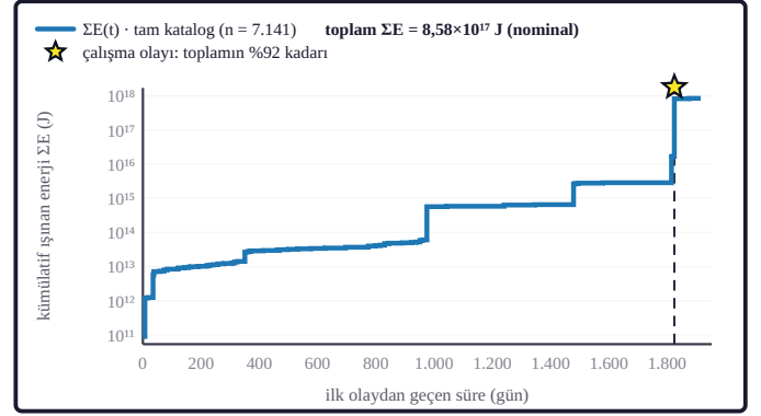
Şekil 6b. Mavi basamak eğrisi kümülatif ısıran sismik enerjidir ( \Sigma E , logaritmik eksen). Kesikli düşey çizgi çalışma olayını işaretler; en büyük tek katkı bu olaydır (Gutenberg ve Richter, 1956 enerji bağıntısı).
