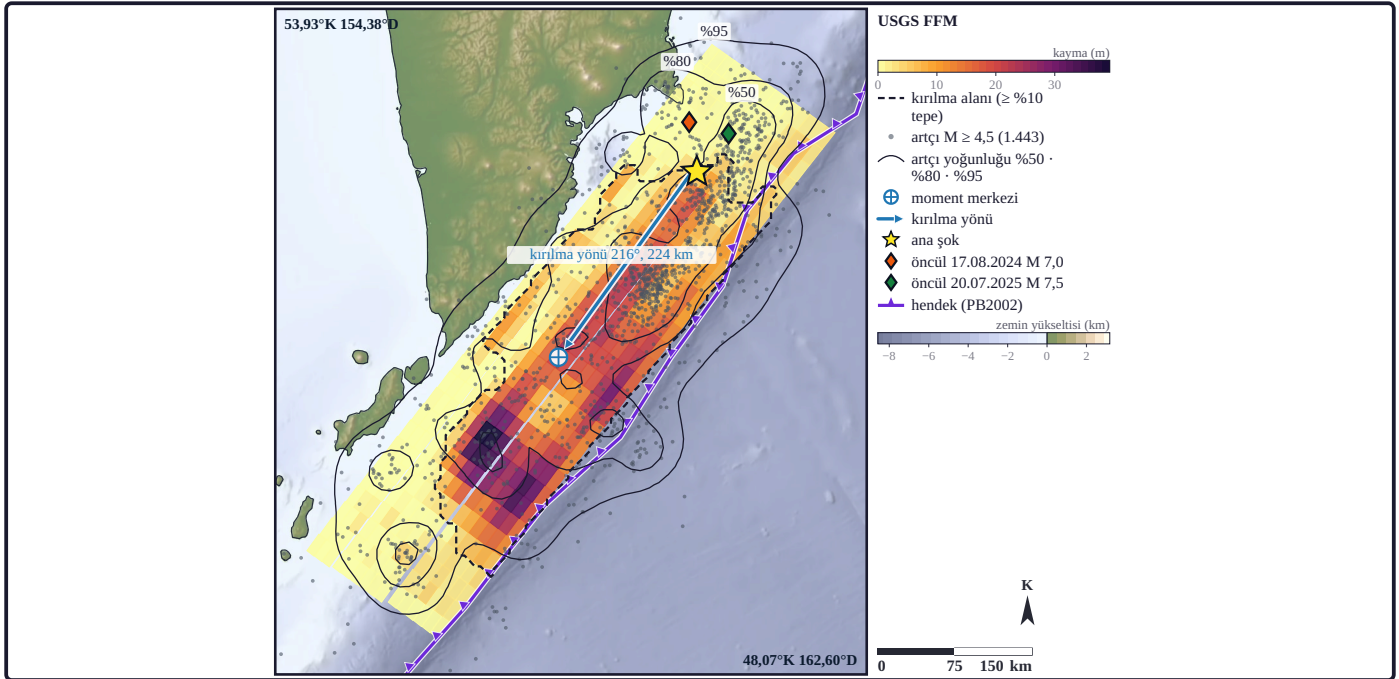
Şekil 13. Renkli dörtgenler USGS NEIC us6000qw60 (model 30) kayma modelinin 465 yamasının yatay izdüşümü; renk yama kaymasıdır (0–39,3 m, model çıktısı); kesikli siyah çizgi kırılma alanı (kayma \geq 3,9 m); gri noktalar M \geq 4,5 artçılar ( n = 1.443 ); ince siyah eğriler yoğunluğun %50, %80 ve %95 kütle sınırları; mavi artılı daire moment merkezi, mavi ok kırılma yönü 216^\circ , 224 km; sarı yıldız ana şok, elmaslar büyük öncüller (model: kurum ürünü: USGS NEIC sonlu fay modeli us6000qw60 [U.S. Geological Survey, 2017]; artçılar: USGS NEIC [ComCat] [U.S. Geological Survey, 2017]; kırılma alanı, artçı yoğunluğu, moment merkezi: Seismo Lab hesabı; levha sınırı: Bird, 2003 [iz, ETOPO 2022 hendek ekseninden ortalca \approx 12 km kara yönünde]; altlık ve kıyı çizgisi: ETOPO 2022 [30" ızgara, NOAA NCEI, doi:10.25921/fd45-gt74]; renk: oleron [Crameri, 2018]).
