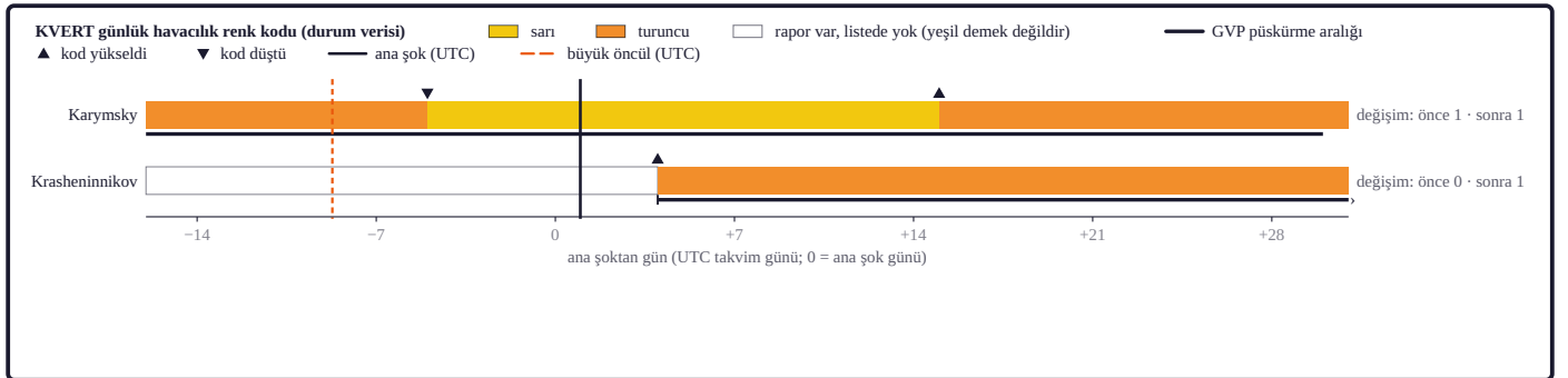
Şekil 6d. 13.07.2025–28.08.2025 (47 gün) penceresinde KVERT'in (IVS FEB RAS) günlük havacılık renk kodu, ana şoktan gün ekseninde (0 = ana şokun UTC günü; dikey düz çizgi ana şok, kesikli çizgi büyük öncül); aynı durumdaki ardışık günler tek parçadır; KVERT görseli değil, durum verisinden bu çalışmanın çizimidir. Satırlar volkanın kırılma izine uzaklığına göre sıralıdır (en yakın üstte). KVERT yalnız sarı ve üstündeki volkanları listeler: boş çerçeveli parça o günlerde rapor alındığını ama volkanın listede olmadığını gösterir ve "yeşil" anlamına gelmez (47 / 47 gün rapor var). Yukarı bakan üçgen kodun bir önceki raporlu güne göre yükseldiği, aşağı bakan üçgen düştüğü gündür; sağdaki sayım pencere içindeki değişimlerin ana şoktan önce ve sonra kaç kez olduğunu verir. Pencere büyük öncülü (20.07.2025 06:49:04 UTC, M 7,5) kapsayacak biçimde kurulmuştur (başlangıç = min(olay günü - 7 g, olaydan önceki 30 g içindeki en erken büyük öncülün günü - 7 g); bitiş = olay günü + 30 g). Çubuğun altındaki ince çizgi GVP püskürme aralığıdır (Krashennnikov 2025-08-02 → 2026-03-25 (sürüyor); Karymsky 2025-04-29 → 2025-08-27); kesikli çizgi gün hassasiyetinde olmayan başlangıçtır; GVP tarihleri volkanın yerel takvim günüdür ve UTC eksenine \pm 1 gün belirsizlikle yerleştirilmiştir. Deprem ile püskürme arasındaki zamansal yakınlık tek başına nedensellik kanıtlamaz. KB GS RAS vmon arşivi 19.10.2026 tarihinden başladığı için bu pencerede vmon verisi yoktur (çekilmedi; "rapor yok" anlamında değildir) (veri: KVERT [Kamchatkan Volcanic Eruption Response Team, IVS FEB RAS] günlük raporları; Global Volcanism Program, Smithsonian Institution).
