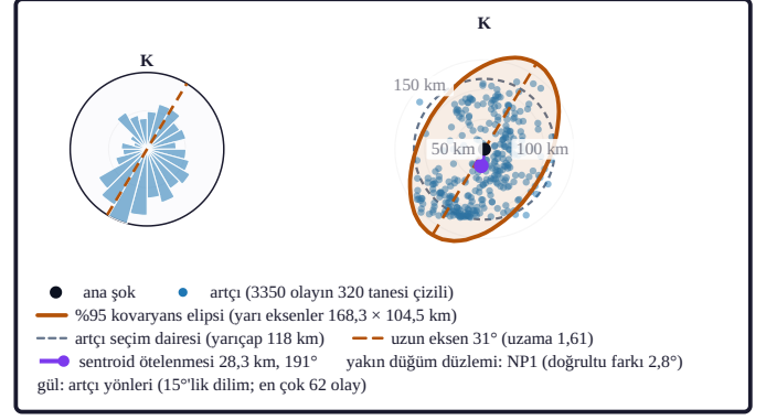
Şekil 9b. Ana şok merkezli düzlemde artçı bulutu (mavi) ve %95 kovaryans elipsi (turuncu) gösterilmiştir. Elips, artçı konumlarının kovaryansından Gauss dağılımı varsayımıyla kurulan bir yayılım ölçüsüdür; artçıların %95'ini içeren bir sınır değildir. Turuncu kesikli doğru elipsin uzun eksenidir, mor ok artçı sentroidinin ana şoka göre ötelenmesidir; gri çemberler ana şoka uzaklığı kilometre cinsinden ölçekler, gri kesikli çember artçıların seçildiği dairedir. Bulut bu daireye dayandığından uzama oranı seçim yarıçapıyla sınırlıdır (gerçek değer için alt sınır) ve sentroid dış merkeze doğru yanlıdır. Uzama oranı 1'e yaklaştıkça bulut izotroplaşır ve yön kestirimi zayıflar; elips ölçüleri ve uzun eksene yakın düğüm düzlemi lejantıdır (telesismik ikinci moment ölçüsünün artçı konumlarına uyarlanmış şekli: McGuire vd., 2002).
