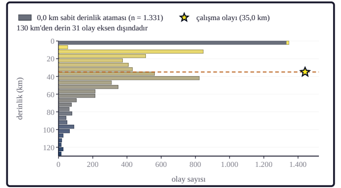
Şekil 2d. Tam katalogta derinlik değeri taşıyan 7.141 olayın %30'u ≤ 10 km derinliktedir. Sabit derinlik atamaları (0,0 km) ölçülmüş derinlik taşımaz. Hiposantr derinlik histogramı (tam katalog): çubuk rengi derinliği gösterir (sıkı sarı, derin lacivert); koyu kesim sabit derinlik atamalarıdır; yıldız ve kesikli çizgi çalışma olayının derinliğidir.
