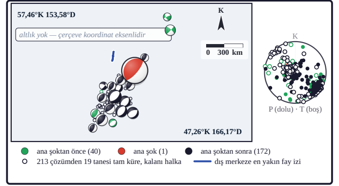
Şekil 7b. Arama penceresinin (ana şoktan 180 gün önce – 30 gün sonra, 660 km yarıçap) odak mekanizması haritasında her odak küresi bir moment tensörü çözümüdür. M_w , çözümü yayımlayan kurumun moment tensörü büyüklüğüdür ve gövdedeki katalog büyüklüğünden farklı olabilir. Küre rengi ana şoka göre zamanı (yeşil önce, kırmızı ana şok, siyah sonra), çapı büyüklüğü taşır. Küreler alt yarıküre eşit alan izdüşümündedir; mavi çizgi dış merkeze en yakın fay izi, ince kırmızı çizgiler haritalanmış diri fay izleridir. Zaman sınıfları bir pencere kuralından gelir ve bir yorum değildir. Arama penceresi raporun analiz penceresinden farklıdır (moment tensörleri ve M_w : Global CMT, Ekström vd., 2012; izdüşüm: Lambert alt yarıküre eşit alan).
