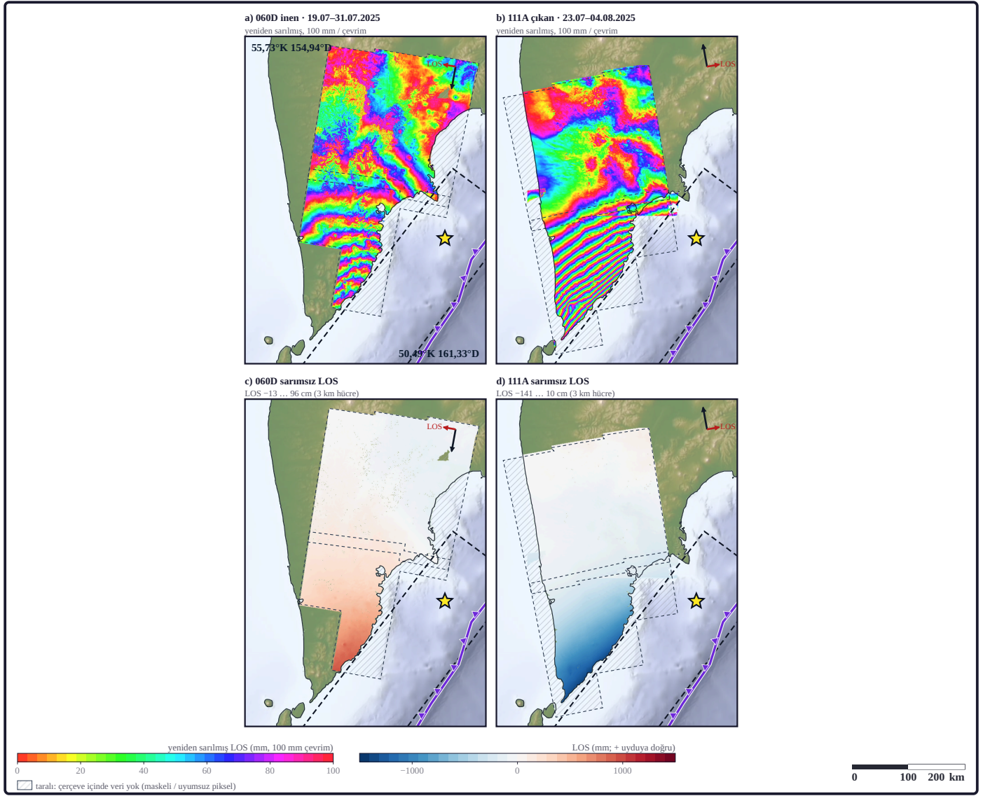
Şekil 25. Sentinel-1 ko-sismik interferogramları (COMET-LiCSAR): 060D inen iz 19.07–31.07.2025; 111A çıkan iz 23.07–04.08.2025; a, b panelleri yeniden sarılmış (100 mm), c, d panelleri sarımsız LOS (+ uyduya doğru); değerler uzak alana göre görelidir; çerçeveler ötelenerek birleştirildi: 060D +280 mm (MAD 0,9), 111A –443 mm (MAD 6,8) (InSAR: LiCSAR contains modified Copernicus Sentinel data 2025 analysed by the Centre for the Observation and Modelling of Earthquakes, Volcanoes and Tectonics [COMET]. LiCSAR uses JASMIN, the UK's collaborative data analysis environment [http://jasmin.ac.uk]; Copernicus Sentinel-1 verisi [değiştirilmiş] [Lazecký vd., 2020]; model konturu: kurum ürünü: USGS NEIC sonlu fay modeli us6000qw60 [U.S. Geological Survey, 2017]; altlık ve kıyı çizgisi: ETOPO 2022 [30" ızgara, NOAA NCEI, doi:10.25921/fd45-gt74]; renk: oleron [Crameri, 2018]).
