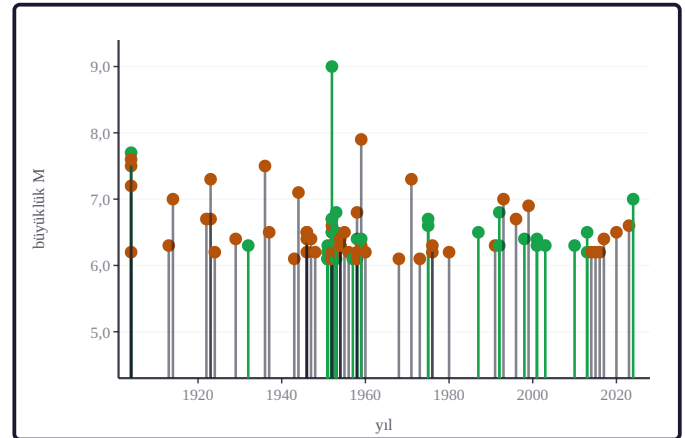
Şekil 35b. Tarihsel eşik üstü depremlerin büyüklükleri yıllara göre çizilmiştir; yeşil yakın kuşak, turuncu bölge kuşağıdır (birleşik katalog, 1900 sonrası; büyüklükler, varsa ISC-GEM Mw: International Seismological Centre, 2026; Di Giacomo vd., 2015, 2018).
