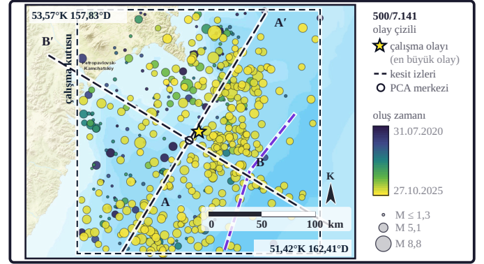
Şekil 8d. Daire rengi oluş zamanını (koyu mor en eski → sarı en yeni), çapı büyüklüğü verir. Öbür imler Şekil 3d'deki gibidir (kesikli dikdörtgen çalışma kutusudur).
