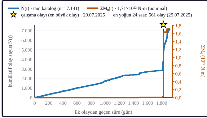
Şekil 6a. Mavi eğri kümülatif olay sayısı N(t) , turuncu eğri kümülatif sismik moment \Sigma M_0(t) değeridir. Sarı yıldız çalışma olayıdır; penceredeki en büyük olay da odur ( M_0 = 10^{[1,5 \cdot M + 9,1]} \text{ N} \cdot \text{m} ; 9,1 sabiti Kanamori, 1977).
