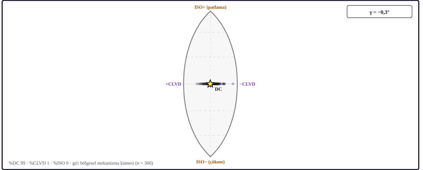
Şekil 10a. Tape ve Tape kaynak tipi lune'unda sarı yıldız bu olayın moment tensörünü, artı imi saf çift kuvvet (DC) merkezini gösterir. Çerçeve \gamma \in [-30^\circ, +30^\circ] ve \delta \in [-90^\circ, +90^\circ] aralığının Hammer eşit alan izdüşümüdür; kesikli yaylar \delta = 0, \pm 30^\circ ve \pm 60^\circ enlemleridir. Sağ ve sol kenarlar \pm CLVD uçları, kutuplar izotropik patlama ve çökme uçlarıdır. Gri noktalar bölgesel mekanizma kümesinin çözümleridir; alt satırdaki yüzeler DC/CLVD/ISO ayrışımıdır (lune: Tape ve Tape, 2012; ayrışım: GCMT tensöründen).
