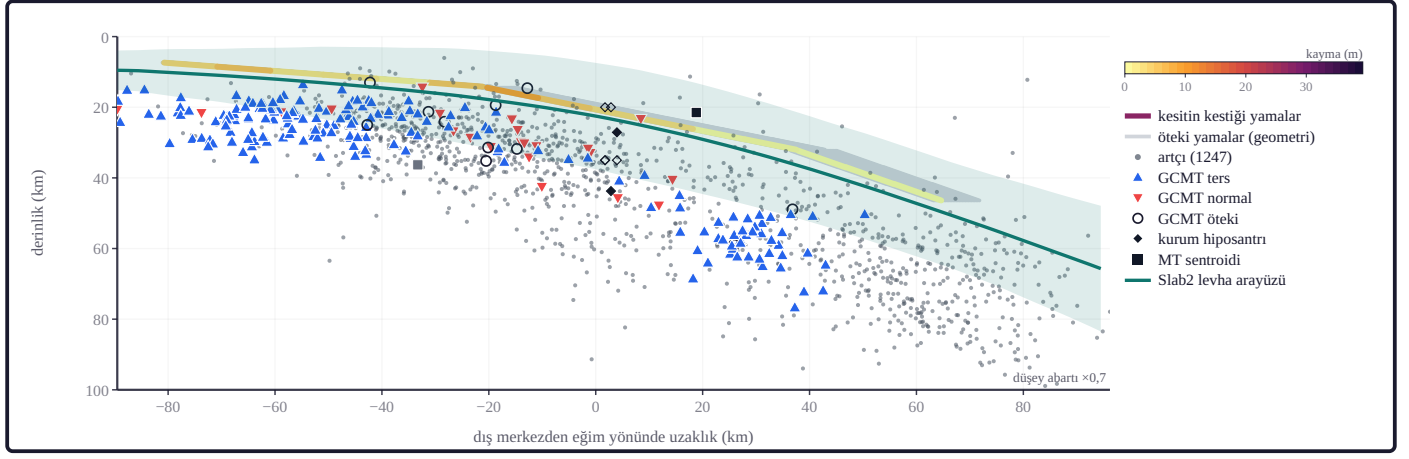
Şekil 15. Kesit dış merkezden geçen ve USGS NEIC us6000qw60 (model 30) modelinin temsili doğrultusuna (217°) dik düşey düzlemdir; yatay eksen eğim yönünde (307°) uzaklıktır, eksi değerler eğim yukarıdır; şerit modelin doğrultu boyunca kapladığı 625 km'dir; renkli parçalar USGS FFM modelinin kesitin kestiği 15 yaması (kayma 0–39,3 m; model), açık gri öteki yamalar (geometri); noktalar artçılar (1.247; sabit derinlikli 1.677 çizilmedi); imler GCMT artçıları, sentroid derinliği; sabit 19 çizilmedi; elmaslar kurum hiposantr derinlikleri (içi boş: sabit / bağımlı) (model: kurum ürünü: USGS NEIC sonlu fay modeli us6000qw60 [U.S. Geological Survey, 2017]; artçılar: USGS NEIC [ComCat] [U.S. Geological Survey, 2017]; GCMT: Dziewonski vd., 1981; levha yüzeyi: Slab2 [Hayes, 2018], Seismo Lab hesabı).
