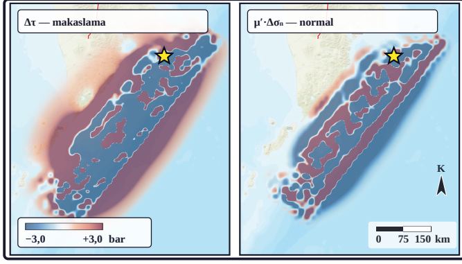
Şekil 9a. \Delta CFs 'in iki bileşeni ayrı panellerde gösterilmiştir: solda makaslama gerilmesi değişimi \Delta\tau , sağda fay düzlemine dik normal gerilme katkısı \mu'\Delta\sigma_n ( \Delta CFs = \Delta\tau + \mu'\Delta\sigma_n ; \Delta\sigma_n çekme artı, artı değer fayın kenetlenmesinin azalmasıdır). Kadraj kaynak çevresine yakınlaştırılmıştır; renk ölçeği ve kaynak geometrisi \Delta CFs haritasıyla aynıdır; yıldız dış merkezdir (bileşen ayrışımı: Okada, 1992 analitik çözümü; kurum ürünü: USGS NEIC sonlu fay modeli us6000qw60 [U.S. Geological Survey, 2017]).
