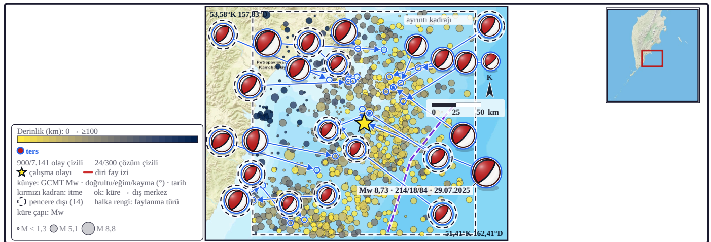
Şekil 35c. Bölgesel odak mekanizması çerçevesi: harita, çevrede yayımlanmış çözümlerin Mw sırasıyla en büyüklüklerini gösterir; ötelenen küreler okla konumlarına bağlıdır. Küreler alt yarıküre izdüşümünde odak mekanizmalarıdır; kırmızı kadrantlar P dalgasının ilk hareketinin itme olduğu bölgelerdir. Mw sırasıyla en büyük 1 çözüm künyelidir (öbür 23 küre künyesizdir); künye çözümün moment büyüklüğünü (GCMT Mw), bir düğüm düzleminin doğrultu, eğim ve kayma açısını ve tarihini verir. Küçük daireler pencere olayları, kesikli dikkörtgen ayrıntı haritasının kadrājıdır (mekanizma kümesi: bölgesel küme [n = 300]; gerilme inversiyonu olay merkezli mekanizma popülasyonundandır [n = 467]; faylar: GEM Global Active Faults [Styron ve Pagani, 2020] — CC BY-SA 4.0).
