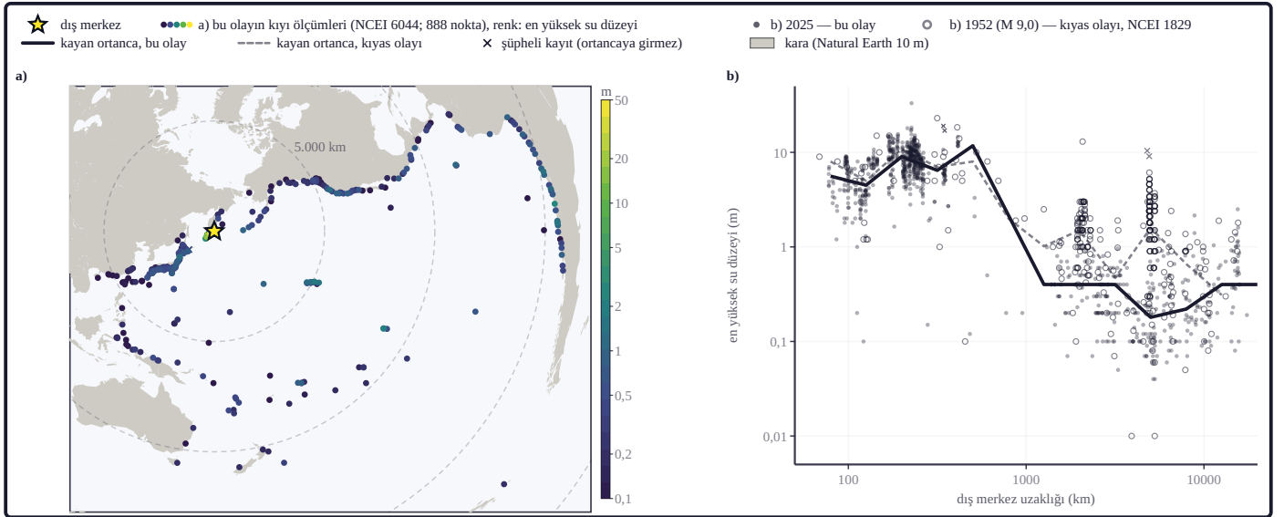
Şekil 31b. Kıyılarda ölçülen tsunami yükseklikleri: haritada (a) NCEI/WDS Küresel Tarihsel Tsunami Veritabanı'nın bu olaya ait 888 kıyı ölçümü, NCEI 6044; DART kayıtları hariç. Renk en yüksek su düzeyidir, logaritmik 0,1–50 m; alt sınır 0,1 m ile verinin %2'lik değerinin büyüğüdür, yüksek değerler üstte çizilir. Uzaklık panosunda (b) aynı ölçümler dış merkez uzaklığına göre log-log eksenle koyu noktalarla gösterilir; gri boş daireler 1952 olayının 315 ölçümüdür, NCEI 1829, M 9,0, ve yalnız bu panoda çizilir; kıyas olayı, iki olayda da en az 3 kayıtlı en çok ortak kesimi olan önceki depremler tsunamidir (14 ortak kesim). Koyu kalın çizgi ve gri kesikli çizgi kayan ortancadır: 0,2 log 10 km genişlikli kovalar, kovada en az 3 şüphesiz ölçüm, en az 3 kova. NCEI'nin şüpheli (doubtful) işaretli kayıtları x ile çizilir ve ortancaya girmez. Bu olayın en yüksek değeri 33,1 m, tek gözlem; NCEI ölçüm türü kodu 9; NCEI olay kaydının en büyük su yüksekliği alanı 17,0 m'dir, iki alan NCEI'nin ayrı tablolarıdır. NCEI kaydı zamanla büyür; nokta sayıları 20.10.2026 tarihli alıma aittir. Harita dış merkez merkezli eşuzaklık izdüşümüdür; gri dolgu Natural Earth 10 m ülke poligonlarının dış halkalarıdır (kamu malı; iç halkalar çizilmedi; altlık pikseli ≈ 21 km), ETOPO 0 m eğrisi değildir (veri: NCEI/WDS Global Historical Tsunami Database [doi:10.7289/V5PN93H7]; kara: Natural Earth 10 m Admin 0 – Countries [kamu malı; naturalearthdata.com]).
