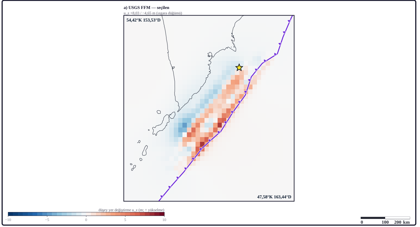
Şekil 28. Panel kayma modelinden hesaplanan kosismik düşey yer değiştirmeler ( u_z , + yükselme): USGS NEIC us6000qw60 (model 30) (seçilen); model ileri hesabı yamaların Okada (1985) yüzey çözümüyle toplamıdır: homojen elastik yarı uzay (katmanlı ortam değil); bütün model değerleri model çıktısıdır; renk ölçeği seçilen modelin tepesine göre \pm 10 m'de doyar; panel kendi uçlarını (kaba ızgara düğümünde) yazar; PB2002 hendek izi, ETOPO 2022 batimetrisindeki hendek ekseninden ortalca \approx 10 km kara (üst levha) yönündedir (iz boyunca 10 km aralya 84 dik kesitte en derin nokta; %10–90 aralığı 5 ile 30 km); iz yayımlandığı gibi çizilmiştir (model: kurum ürünü: USGS NEIC sonlu fay modeli us6000qw60 [U.S. Geological Survey, 2017]; yöntem: Okada, 1985; kıyı çizgisi [0 m eğrisi]: ETOPO 2022 [30" ızgara, NOAA NCEI, doi:10.25921/fd45-gt74]).
