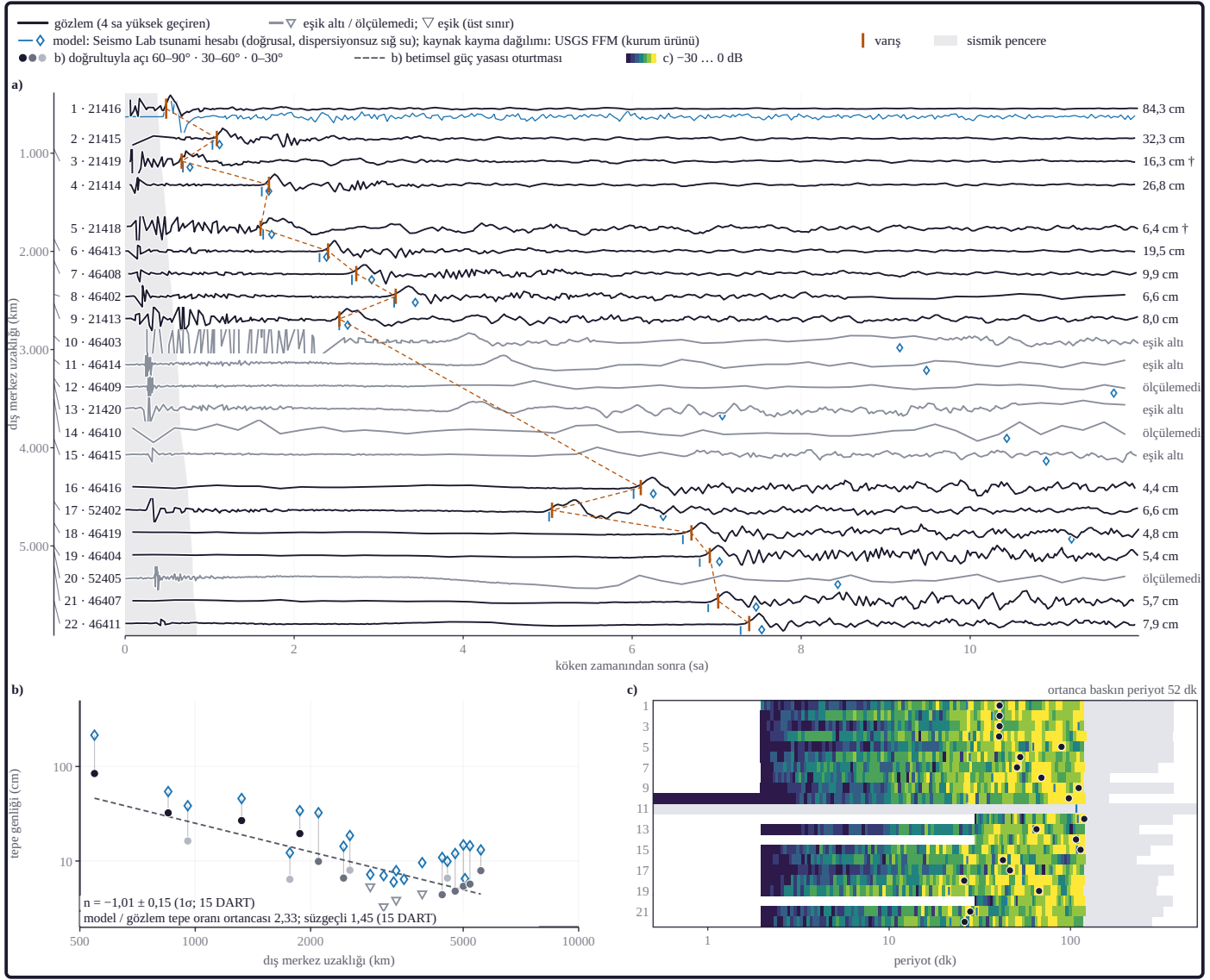
Şekil 32. DART kayıt kesiti, tepe genişliğinin uzaklıkla değişimi ve spektral kesit: 22 DART istasyonunda gelgiti ayıklanmış, olay öncesi tabanı çıkarılmış ve 4 sa Hann yüksek geçirenden geçirilmiş su sütunu yüksekliği sapmaları; gözlem, veri NOAA NDBC DART. Mavi ince çizgi ve \diamond modeldir, gözlem ya da resmi tahmin değildir; hesap: Seismo Lab tsunami hesabı (doğrusal, dispersiyonsuz sığ su); kaynak kayma dağılımı: USGS NEIC us6000qw60 (kurum ürünü); ilk koşul Okada (1985), Tanioka ve Satake (1996) yatay katkısı ve Kajiura (1963) süzgeci; ızgara 2', batimetri NOAA NCEI ETOPO 2022, 60" yüzey modeli; kıyı taşkını yok; model izi gözlemin altında, aynı ölçekle ve gözlemle aynı 4 sa yüksek geçirenden geçirilmiş; yarı yüksekliği 4 birimden küçük izlerde yalnız model tepesi \diamond ve gözlemin algılandığı istasyonlarda model varışı imlenir. Veri tutarsızlığı: NCEI'nin aynı DART için verdiği değer bu ölçümden farklıdır (21415: NCEI 20 cm \leftrightarrow bu çalışma 32,3 cm; 21419: NCEI 9 cm \leftrightarrow bu çalışma 16,3 cm); iki değer ayrı kurumların ayrı yöntemleridir. Kayıt kesitinde (a) izler gerçek uzaklık ölçeğinde dizilidir; 7 birimden yakın izler en çok 12 birim aşağı kaydırılıp gerçek uzaklığa ince gri çizgiyle bağlanmıştır; her iz kendi tepe genişliğine, eşik altında algılama eşiğine göre ölçeklidir; solda uzaklık sırası ve DART numarası, sağda tepe değeri yazar. Tepe genişliği ile uzaklık panosu (b) log-log eksenlidir; kesikli doğru algılanan istasyonların betimsel güç yasası oturtmasıdır, yön etkisi ayıklanmamıştır: n = -1,01 \pm 0,15 (1 \sigma , 15 istasyon); eşik altı istasyonlar eşik değerinde \nabla üst sınırdır ve oturtmaya girmez; nokta tonu çıkış azimutunun GCMT çözümünün doğrultusuyla (214°) açısidir; model / gözlem tepe oranının ortancası 2,33, 10 dk alçak geçirenle 1,45, 15 DART; varış farkının, model eksi gözlem, ortancası -3,1 dk. Spektral kesitte (c) her satır kayıt kesitindeki istasyonun genlik spektrumudur; renk satır içinde -30 ile 0 dB arası, 5 dB basamaklı; açık gri hücreler güvenilir sayılmayan ya da 120 dk'dan uzun periyotlardır; 0 dB düzeyi ve baskın periyot, tepe ve varışın ölçüldüğü yüksek geçiren bantta, 120 dk'ya kadar aranır; \bullet gözlemin, mavi çentik modelin baskın periyodudur, ortancası 52 dk (veri: NOAA National Data Buoy Center [NDBC] DART su sütunu yüksekliği; işlem: bu çalışma [harmonik gelgit ayıklama, Hann süzgeci, genlik spektrumu, güç yasası oturtması]; model: Seismo Lab hesabı, doğrusal sığ su; kayma modeli: kurum ürünü: USGS NEIC sonlu fay modeli us6000qw60 [U.S. Geological Survey, 2017]; batimetri NOAA NCEI ETOPO 2022, 60" yüzey modeli, doi:10.25921/fd45-gt74; doğrultu: kurum ürünü: GCMT moment tensörü çözümü [Ekström vd., 2012]).
