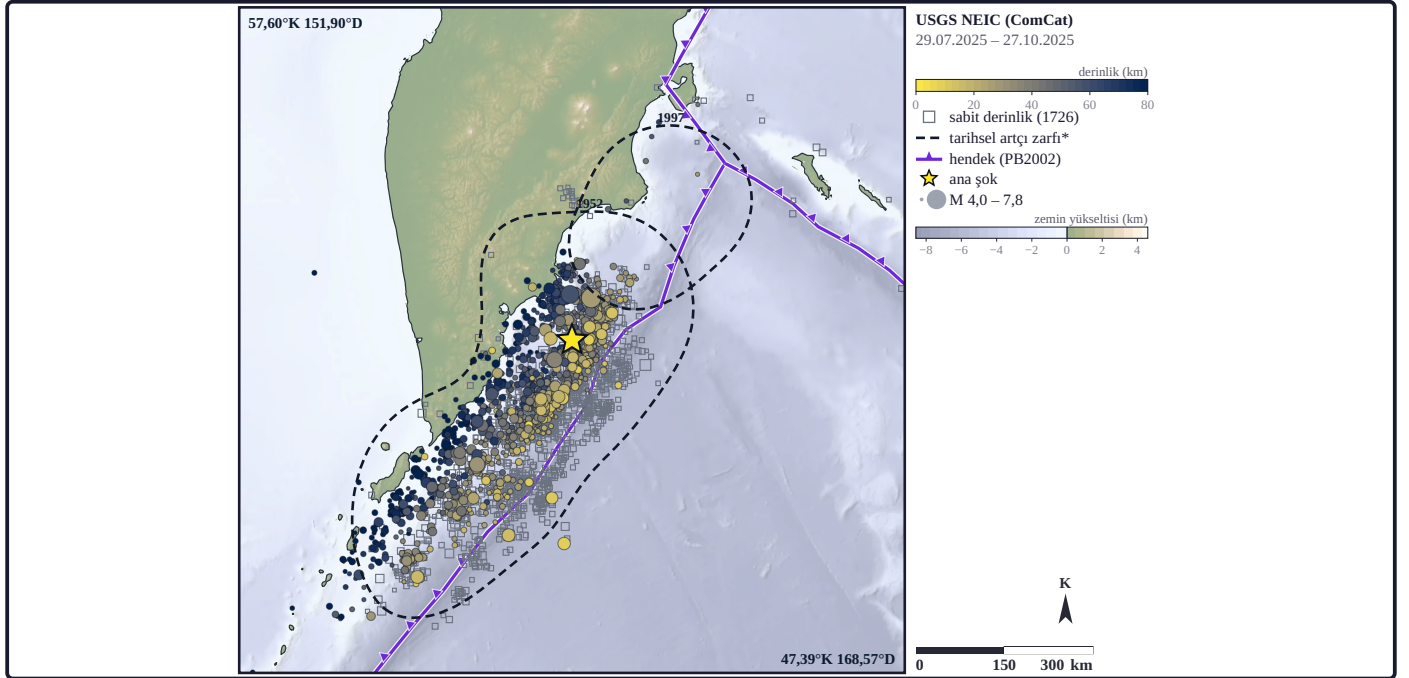
Şekil 4c. Noktalar USGS NEIC (ComCat) kataloğunun kendi raporlarıdır; ana şoktan sonraki 90 gün (29.07.2025 – 27.10.2025), dış merkezin artçı yarıçapı kutusu, n = 3.017; boyut büyüklüğe göre; renk derinliktir (0–80 km; 103 olay daha derin, en koyu renkte); içi boş gri kareler kurumun sabit derinlik değerlerindeki raporlardır (10 / 35 km; 1.726 olay, %57) — bu derinlikler ölçülmüş değildir; kesikli çizgiler 1952, 1997 depremlerinin ilk 30 gündeki artçılarından katalogdan türetilmiş zarflardır; yayımlanmış kırılma poligonları değildir (katalog: USGS NEIC [ComCat] [U.S. Geological Survey, 2017]; artçı zarfları: bu çalışma [katalogdan]; levha sınırı: Bird, 2003 [iz, ETOPO 2022 hendek ekseninden ortanca ≈ 10 km kara yönünde]; altlık ve kıyı çizgisi: ETOPO 2022 [30" ızgara, NOAA NCEI, doi:10.25921/fd45-gt74]; renk: oleron [Crameri, 2018]).
