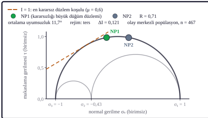
Şekil 7c. Gerilme inversiyonunun normalleştirilmiş Mohr diyagramında yatay eksen normal gerilme \sigma_n , dikey eksen makaslama gerilmesi \tau 'dir. Üç yarım çember asal gerilmelerle kurulan gerilme durumunu, turuncu kesikli doğru \mu sürtünme katsayısıyla tanımlı en kararsız düzlem koşulunu (kararsızlık indeksi I = 1 ) gösterir; iki nokta çalışma olayının iki düğüm düzleminin ( \sigma_n, \tau ) konumudur ve doğruya yakın olan düzlem bu gerilme alanında kaymaya daha yakındır. Şekil oranı R , ortalama kayma yönü düzensizliği ve iki düzlemin kararsızlık farkı \Delta I lejantıdır (Vavryčuk, 2014; kararsızlık ölçütü).
