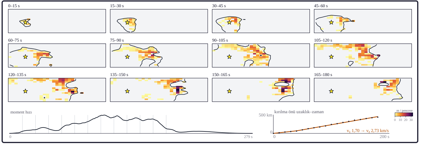
Şekil 20. Kırılma anlık görüntüleri: USGS NEIC us6000qw60 (model 30) kayma modelinin açılmış fay düzleminde (yatay doğrultu boyunca, düşey eğim aşağı) 12 ardışık 15 s'lik pencerede açığa çıkan kayma; renk pencere içindeki kaymadır (ortak ölçek 0–33,1 m; model çıktısı); 180 s'den sonra toplam kaymanın %8,2'si (momentin %6,3'ü) açığa çıkar; panolar ve bu kalan toplam kaymayı verir (fark %0,0); kaynak zaman işlevi yama başına yükselme ve düşme süreli asimetrik kosinüstür (modelin kendi parametreleri); siyah eğri pencere sonundaki kırılma zamanı eş eğrisidir (yama kırılma zamanlarının sürekli enterpolasyonu); küçük pano kırılma önu uzaklık-zaman: v_1 1,70 → v_2 2,73 km/s (model: kurum ürünü: USGS NEIC sonlu fay modeli us6000qw60 [U.S. Geological Survey, 2017]; yöntem: bu çalışma [açılmış düzlem, pencere integrali]).
