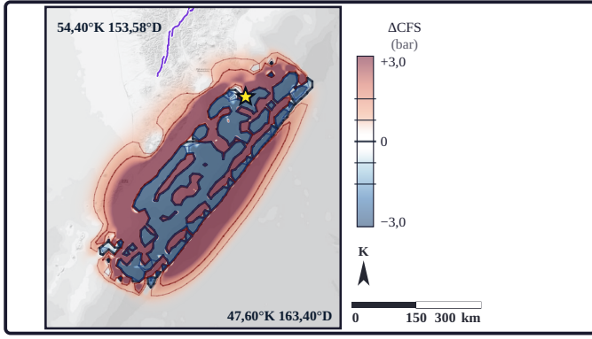
Şekil 8a. Harita statik Coulomb gerilme değişimini ( \Delta CFS ) gösterir (kırmızı artış, mavi azalma; \pm 3,0 bar). \Delta CFS USGS NEIC kaynağının 465 yamasından kaynakla eş yönelimli alıcıda ( s/d/r = 217^\circ/7^\circ/80^\circ ), 15,3 km derinlikte, \mu' = 0,40 ile hesaplanmıştır. Yıldız dış merkezdir; çizgiler \Delta CFS konturlarıdır. Mor çizgiler diri fay izleridir; renk çubuğundaki çentikler kontur düzeyleridir; altlık gri tonludur, renkler yalnız \Delta CFS 'indir ( \Delta CFS : Okada, 1992; King vd., 1994; altlık [gri tonlu]: Esri, HERE, Garmin, © OpenStreetMap contributors, and the GIS user community; diri faylar: GEM Global Active Faults [Styron ve Pagani, 2020] — CC BY-SA 4.0; kurum ürünü: USGS NEIC sonlu fay modeli us6000qw60 [U.S. Geological Survey, 2017]).
