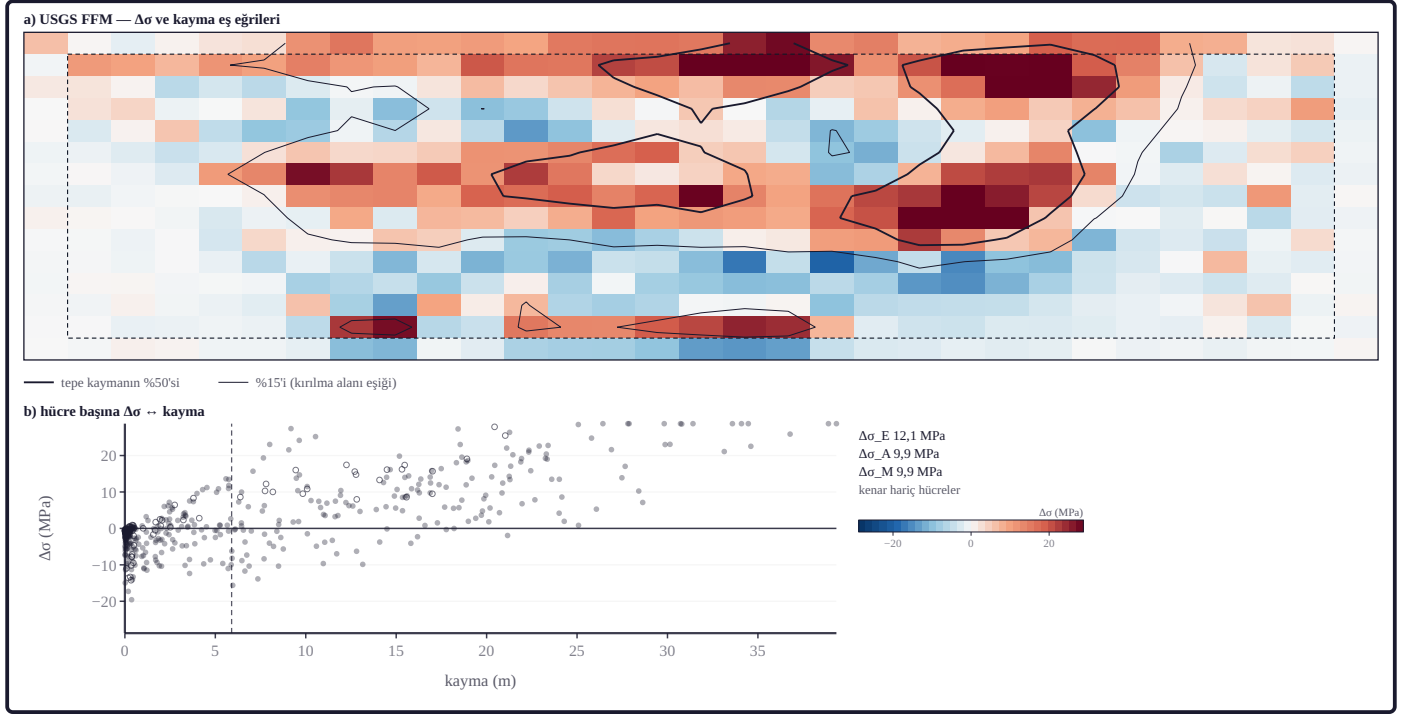
Şekil 21. Fay düzleminde kayma ve statik gerilme düşümü: a) Ripperger ve Mai (2004) \Delta\sigma ( \pm 28,8 MPa; \mu_{eff} 31 GPa; model) ve kayma eş eğrileri; b) hücre başına \Delta\sigma \leftrightarrow kayma; USGS NEIC us6000qw60 (model 30): \Delta\sigma_E 12,1 MPa (bütün hücreler 12,3), \Delta\sigma_A 9,9, \Delta\sigma_M 9,9 MPa; \pm 28,8 MPa dışında kalan 10 hücre b panosunda ölçük sınırında gösterilmiştir; sıg kenar deniz tabanına (serbest yüzey) bir hücreden yakındır ve tepe kaymanın USGS NEIC us6000qw60 (model 30) modelinde %53,5 kadar kayma taşır: hendeğe ulaşan kayma; sonsuz ortam varsayımı bu hücrelerde geçersiz olduğundan kenar hariç değerler esas alınır (model: kurum ürünü: USGS NEIC sonlu fay modeli us6000qw60 [U.S. Geological Survey, 2017]; yöntem: Ripperger ve Mai, 2004; Okada [1992] denetimi).
