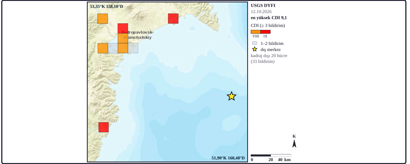
Şekil 30a. Harita USGS “Did You Feel It?” (DYFI) ürününün (12.10.2026) 10 km'lik hücrelerindeki topluluk şiddetini (CDI) gösterir; CDI hücredeki bildirimlerden hesaplanan gözlem değeridir; ürünün 125 bildiriminin 112'si 29 hücrededir; renkli hücreler en az 3 bildirimli 11 hücredir ve rengi CDI değerinin en yakın tam şiddet düzeyidir; bunlardan en yüksek CDI 9,1 (Petropavlovsk-Kamchatskiy, 3 bildirim, dış merkeze 133 km); kadraj dışında 20 hücre (4'ü renkli, 11'i şüpheli; 33 bildirim) kalır; dış merkeze en uzak renkli hücre 2.463 km uzaktadır; gri hücreler 1-2 bildirimlidir ve renklendirilmemiştir; yıldız çalışma olayının dış merkezidir; altlık: Sources: Esri, HERE, Garmin, © OpenStreetMap contributors, and the GIS user community (veri: USGS “Did You Feel It?” [DYFI]; yöntem: Wald vd., 2011; eşik: Atkinson ve Wald, 2007).
