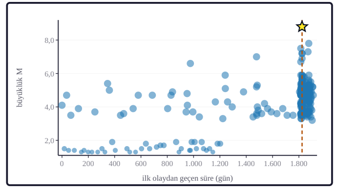
Şekil 2b. Pencere kataloğu 7.141 olaydır (320 olay çizilidir); en büyük olay çalışma olayıdır (Mw 8,8); Mc = 4,2 üstünde 2.354 olay vardır. Büyüklük-zaman dağılımı: yatay eksen ilk olaydan geçen süre (gün), dikey eksen büyüklüktür. Her mavi daire bir olaydır ve daire çapı büyüklükle ölçeklidir; turuncu kesikli dikey çizgi ve yıldız çalışma olayını işaretler (seyreltme eşit adımlıdır; en büyük 10 olay her durumda çizilmiştir).
