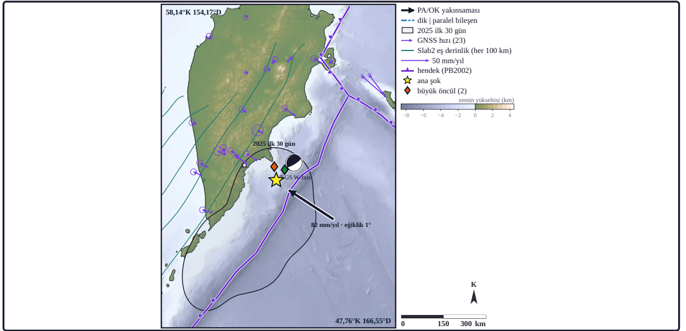
Şekil 10b. Tektonik çerçeve: levha yakınsaması, levha geometrisi ve GNSS hızları: koyu kalın ok PA/OK yakınsaması 82 mm/yıl; mavi düz çizgi dik 82, mavi kesikli çizgi paralel 2 mm/yıl; eğiklik 1^\circ (bu çalışma); mor oklar OK sabit GSRM v2.1 GNSS hızları ( n = 23 ; elips %95); ince koyu çizgili açık alan bu depremin artçı zarfı (ilk 30 gün); küre ana şok MT (kurum ürünü: USGS W-fazı); sarı yıldız ana şok, renkli eşkenar dörtgen öncül (ana şok mekanizması: kurum ürünü: USGS NEIC W-fazı [Mww] [U.S. Geological Survey, 2017]; artçı zarfı: bu çalışma [katalogdan]; GNSS hızları: Kreemer vd., 2014, doi:10.1002/2014GC005407; levha yakınsaması: GSRM v2.1 kutupları; dik / paralel bileşen ve eğiklik bu çalışmanın hesabı [PB2002 hendek kesimi]; levha sınırı: Bird, 2003 [iz, ETOPO 2022 hendek ekseninden ortalca \approx 10 km kara yönünde]; altlık ve kıyı çizgisi: ETOPO 2022 [30" ızgara, NOAA NCEI, doi:10.25921/fd45-gt74]; renk: oleron [Crameri, 2018]; levha yüzeyi: Slab2 [Hayes, 2018], Seismo Lab hesabı).
