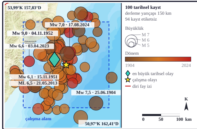
Şekil 35a. Çalışma olayından önceki eşik üstü kayıtlarda daire çapı büyüklüğü, dolgu rengi oluş dönemini gösterir. Turkvaz elmas derlemenin en büyük kaydı, sarı yıldız çalışma olayıdır. Kayıt eşiği yakın kuşakta M \geq 5 , bölge kuşağında M \geq 6 olarak alınmıştır. Mavi kesikli dikdörtgen çalışma alanıdır (birleşik katalog, 1900 sonrası; derleme yarıçapı 150 km, yakın kuşak 60 km).
