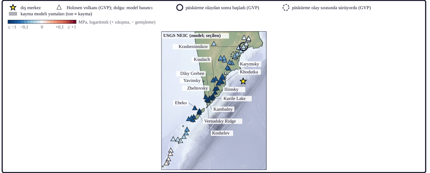
Şekil 22. 58 Holosen volkanı (GVP; min(dış merkez, kırılma izi) ≤ 300 km; aday kümesi USGS NEIC kırılma iziyle kurulmuştur). Üçgen dolgu volkanın altında 2–10 km derinlikteki eşsismik kaya basıncı değişiminin ortalamasıdır ( P = -(\sigma_1 + \sigma_2 + \sigma_3)/3 ; + sıkışma, - genişleme; renk işaretli logaritmik ölçekte ( \pm 0,01 MPa'ya dek doğrusala yakın), \pm 1 MPa'da doygun); basınç MODEL çıkışıdır: USGS NEIC, kamu malı (USGS) kayma modelleriyle ( \mu = 30 GPa, \nu = 0,25 ). Basınç homojen elastik yarı uzay varsayımıyla Okada (1992) çözümünden hesaplanmıştır; topoğrafya ve katmanlı ortam yoktur. Gri tonlu dörtgenler panel modelinin yamalarının yüzey izdüşümüdür (ton kaymayla orantılı). Halka GVP'ye göre olay penceresindeki püskürme durumudur (Krashennnikov: olaydan sonra başladı, 3 gün sonra; Karymsky: olay sırasında sürüyordu; gün farkı volkanın nominal yerel takvim günüdür (GVP tarihleri saat taşımaz; \pm 1 gün). Öbür imler Şekil 6d'deki gibidir. Zemin ETOPO 2022 gölgeli kabartmasıdır (oleron: mavi tonlar deniz, yeşil-kahve tonlar kara); ince koyu çizgi aynı ızgaranın 0 m eğrisidir (gelgit kıyı çizgisi değildir) (volkanlar ve püskürmeler: Global Volcanism Program, Smithsonian Institution; basınç: bu çalışma [model; Okada, 1992]; model: kurum ürünü: USGS NEIC sonlu fay modeli us6000qw60 [U.S. Geological Survey, 2017]; altlık ve kıyı çizgisi: ETOPO 2022 [30" ızgara, NOAA NCEI, doi:10.25921/fd45-gt74]; renk: oleron [Cramer, 2018]).
