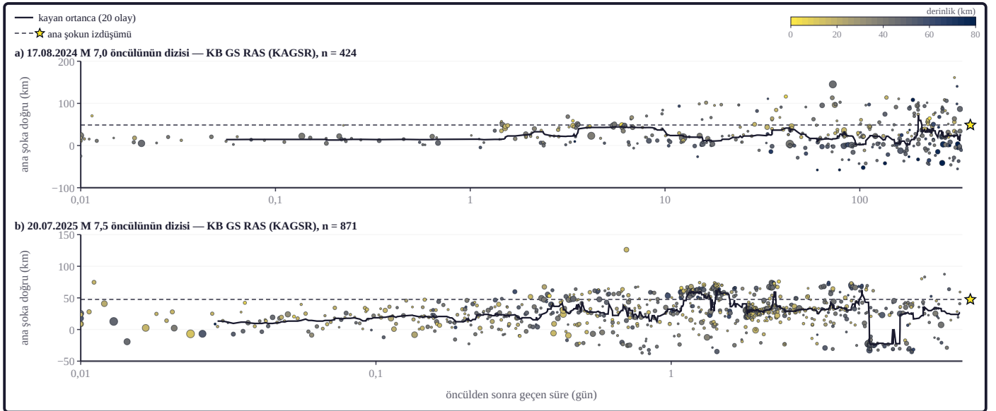
Şekil 5b. Her pano bir büyük öncül dizisidir: yatay eksen öncülden sonra geçen süre (gün, logaritmik), dikey eksen olayın öncülden ana şoka uzanan doğrultuya izdüşümüdür (km; artı yön ana şoka doğru); daireler seçilen katalogun raporlarıdır (renk derinlik, ortak 0–80 km ölçeği; 15 olay daha derin, en koyu renkte; boyut büyüklük); koyu çizgi 20 olaylık kayan ortanca, kesikli yatay çizgi ve sarı yıldız ana şokun izdüşümüdür; katalog her dizide bu çalışmanın kuralıyla seçildi: iki katalogun tamlik büyüklüğünün (azami eğrilik + 0,2) büyüğü ortak eşik alındı, bu eşğin üstünde olay sayısı büyük olan katalog kullanıldı — a) KB GS RAS (KAGSR) (Mc 4,6; USGS NEIC (ComCat) 39, KB GS RAS (KAGSR) 50 olay); b) KB GS RAS (KAGSR) (Mc 4,4; USGS NEIC (ComCat) 193, KB GS RAS (KAGSR) 276 olay) (katalog: KB GS RAS [KAGSR]; katalog seçimi, izdüşüm ve kayan ortanca: bu çalışma).
