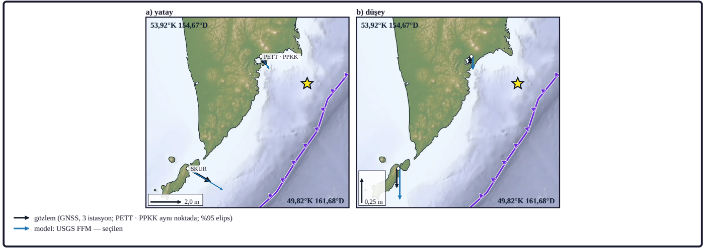
Şekil 27. Siyah oklar GNSS gözlemidir (3 istasyon): Nevada Geodetic Laboratory günlük konumlarında olay gününü dışlayan iki pencerenin ortanca farkı (2025-07-21 – 2025-07-28 ↔ 2025-07-30 – 2025-08-02); elips ve çentik %95 belirsizliktir; PETT ve PPKK istasyonları 33 m arayla şekil ölçeğinde aynı noktadadır; tek işaret ve tek etiketle (PETT · PPKK) gösterilmiştir; önce-penceresi büyük öncülden sonra başlar; mavi oklar model ileri hesabı: Okada (1985) homojen yarı uzay ileri hesabı; model çıktısı; PB2002 hendek izi ETOPO 2022 ekseninden ≈ 10 km kara (üst levha) yönündedir (model: kurum ürünü: USGS NEIC sonlu fay modeli us6000qw60 [U.S. Geological Survey, 2017]; yöntem: Okada, 1985; GNSS: Blewitt vd., 2018; Blewitt vd., 2016; altılık ve kıyı çizgisi: ETOPO 2022 [30" ızgara, NOAA NCEI, doi:10.25921/fd45-gt74]; renk: oleron [Cramer, 2018]).
