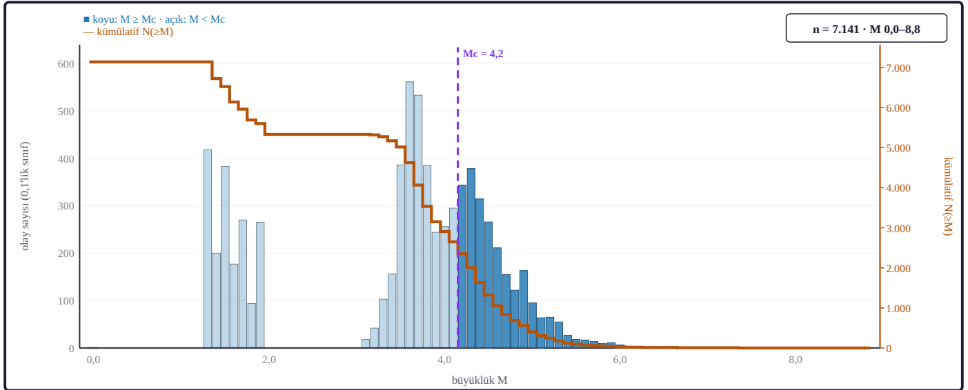
Şekil 34. Pencere kataloğunun tamamında tamlık büyüklüğü M_c = 4,2 olarak benimsenmiştir (uyum iyiliği ölçütü); bu eşikte uyum iyiliği %92,4 düzeyindedir; pencerenin en büyük olayı çalışma olayıdır ( M_w 8,8 ). Mavi çubuklar 0,1 genişliğindeki büyüklük sınıflarına düşen olay sayısıdır (sol eksen); turuncu eğri kümülatif N(\geq M) sayımıdır (sağ eksen). Mor kesikli çizgi pencere kataloğunun tamamının tamlık büyüklüğüdür; olay sonrası dönemin b değeri bu çizgiyle değil, o dönemin kendi tamlık eşiğiyle ( M_c = 4,9 ) kestirilmiştir. Çizginin altındaki sınıflar açık dolguludur (tam katalog, n = 7.141 ).
