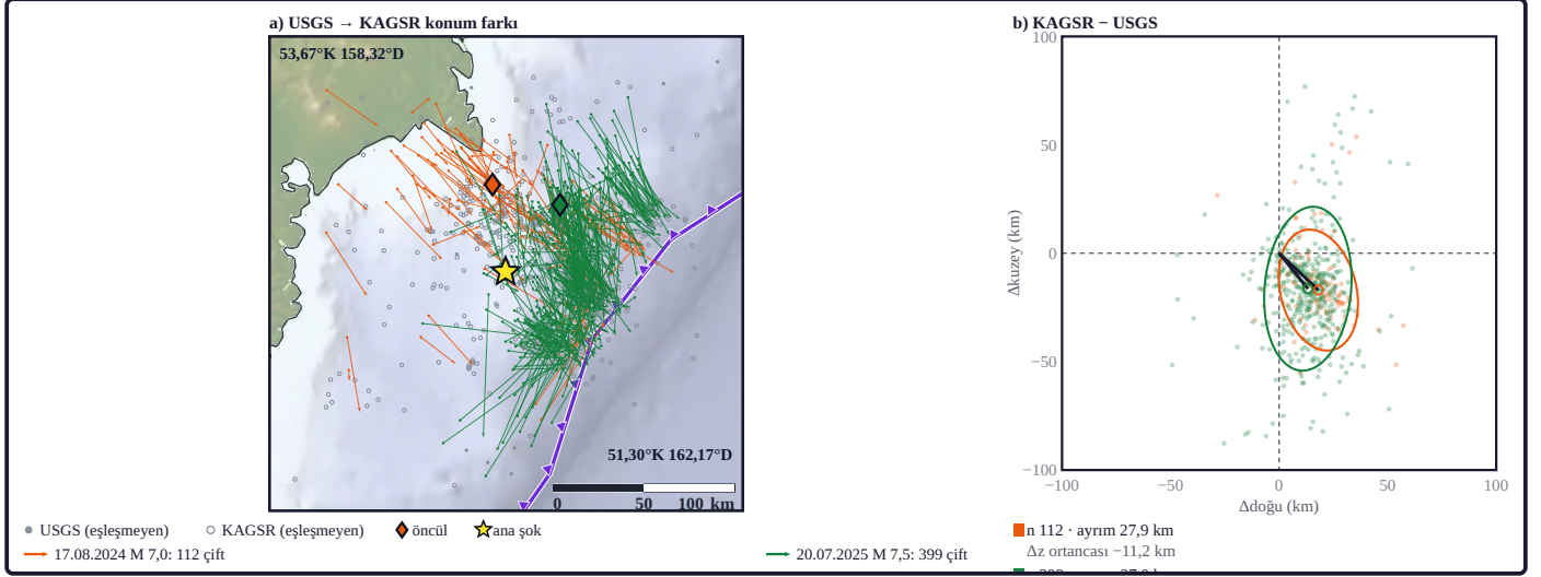
Şekil 5a. a) Büyük öncül dizilerinde iki katalogun aynı olay saydığı her çift için USGS NEIC (ComCat) konumundan KB GS RAS (KAGSR) konumuna ok (renk dizi: turuncu 17.08.2024 M 7,0 dizisi, yeşil 20.07.2025 M 7,5 dizisi; pencere öncülden 1 sa önce başlar ve öncülden en çok 336,4 gün sonra ya da ana şokta biter); eşleşmeyen raporlar gri: USGS NEIC (ComCat) dolu, KB GS RAS (KAGSR) içi boş daire; b) çift başına KB GS RAS (KAGSR) - USGS NEIC (ComCat) konum farkının doğu ve kuzey bileşenleri (eşit ölçek, \pm 100 km); koyu ok pencerenin ortanca farkıdır, ucundaki halka dizinin renginde; elips ortanca çevresindeki %68 kovaryans elipsidir (en az 10 çift); pano altındaki değerler çift sayısı, ayırım ortancası ve \Delta z ortancasıdır ( \Delta z yalnız sabit derinlikli olmayan eşlerden); PB2002 hendek izi ETOPO 2022 ekseninden \approx 10 km kara (üst levha) yönündedir (kataloglar: USGS NEIC [ComCat] [U.S. Geological Survey, 2017]; KB GS RAS [KAGSR]; ötelenme: bu çalışma; altlık ve kıyı çizgisi: ETOPO 2022 [30" ızgara, NOAA NCEI, doi:10.25921/fd45-gt74]; renk: oleron [Crameri, 2018]).
